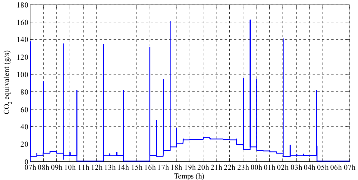
Fig. 4.67. CO 2 équivalent (g/s)
