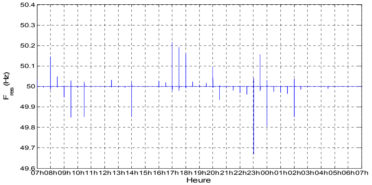
Fig. 4.28. Fréquence réseau
