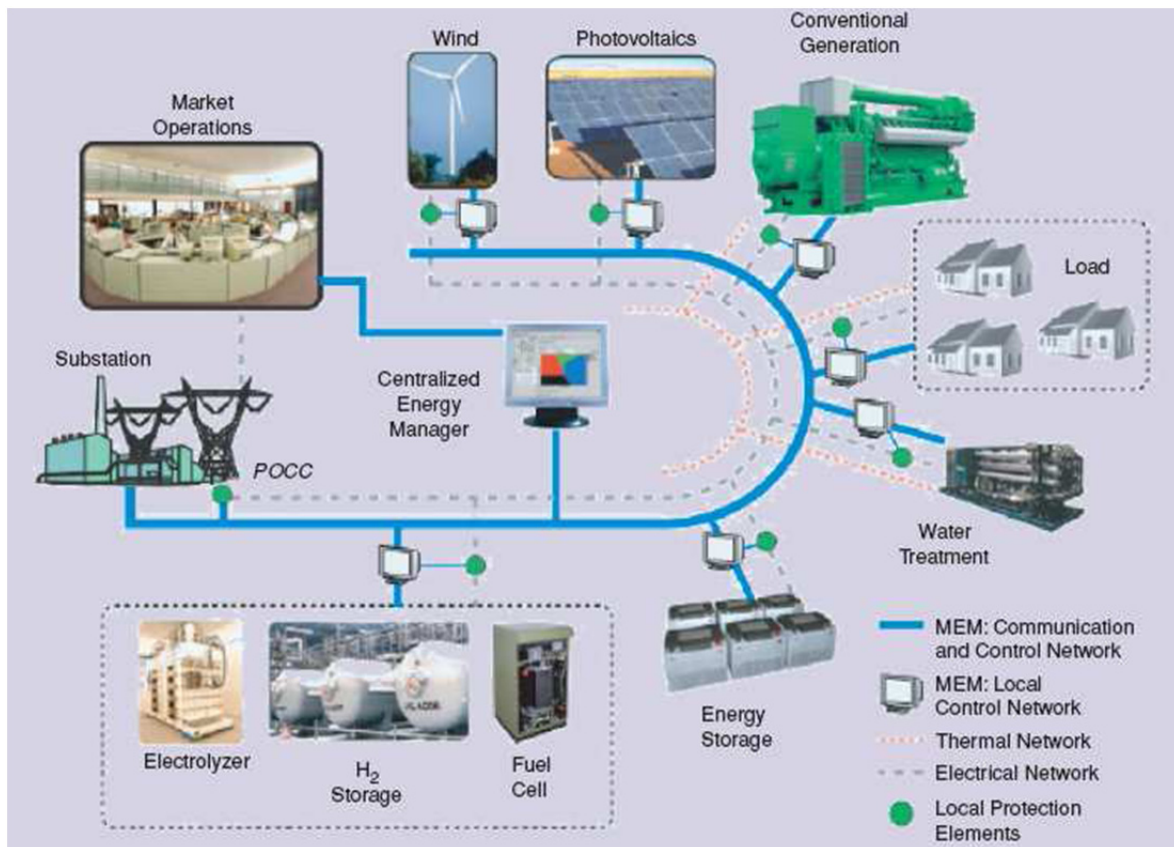
Fig. 1.19. Architecture du micro-réseau expérimental de General Electric [Cer 10]
