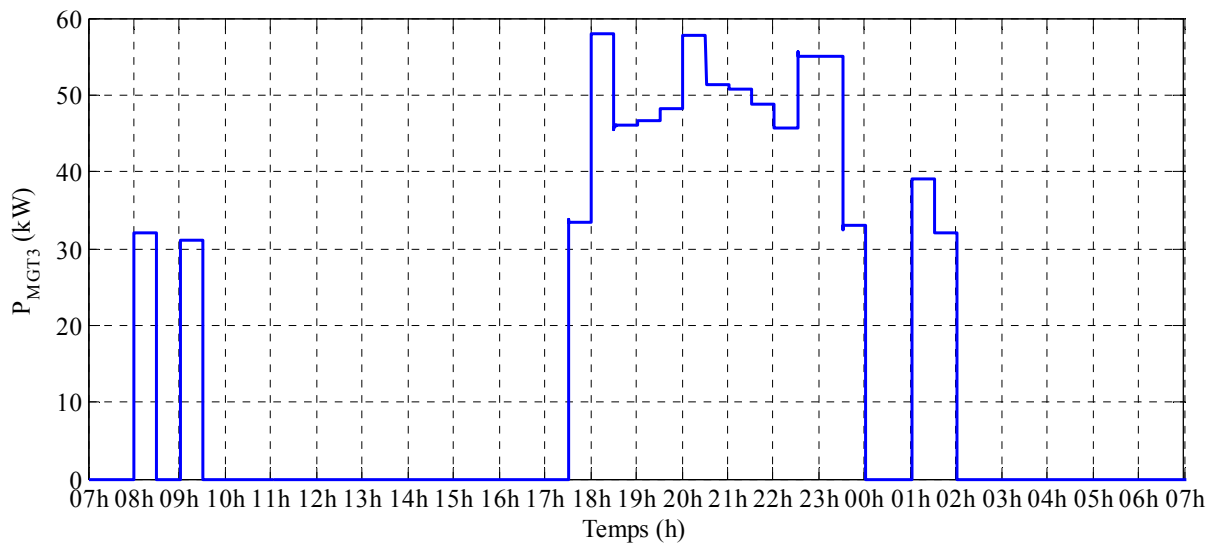
Fig. 4.80. P_{MGT\_3}
