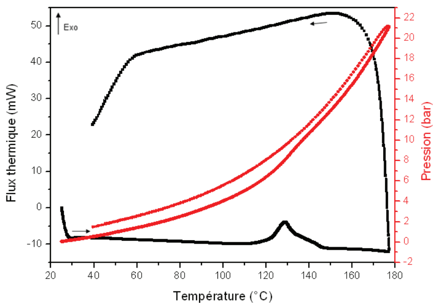
Figure 3-15: Thermogramme du HKUST-1 avec une vitesse de chauffe de 0,1°C/mn (expérience 4)
