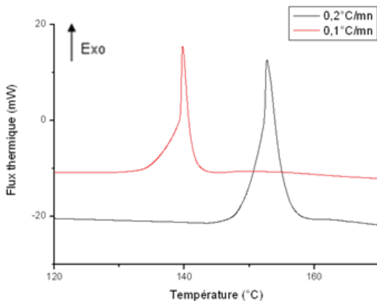
Figure 3-13 : Comparaison des thermogrammes du mélange \text{Cu}(\text{NO}_3)_2 \cdot \text{H}_2\text{O}/\text{EtOH} à 0,1 et 0,2°C/mn
