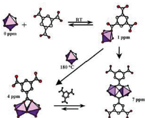
Figure 1-13 : Formation des intermédiaires durant la synthèse des MIL-96, MIL-100 et MIL-110 108
