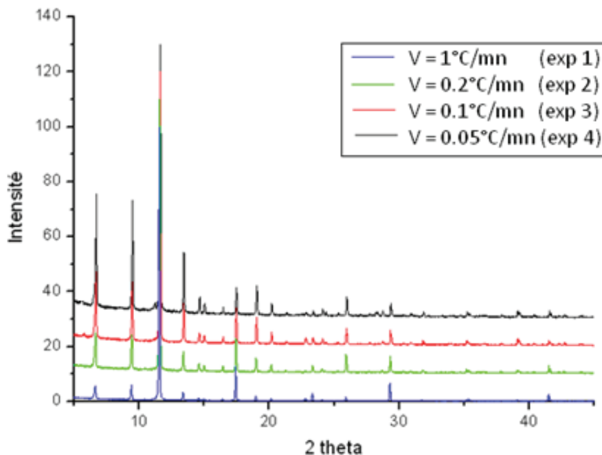
Figure 3-23 : Comparaison par DRXP des échantillons obtenus en calorimétrie C80 à des vitesses de chauffe différentes
