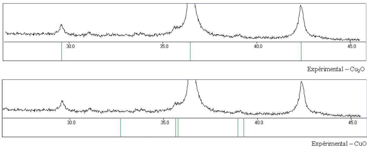
Figure 3-12 : Comparaison entre les diffractogrammes théoriques d'oxydes de cuivre et l'échantillon formé lors de la synthèse solvothermale
