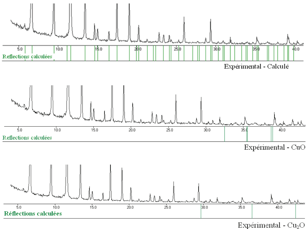
Figure 3-14 : Comparaison entre les diffractogrammes de poudre du CuO/ Cu 2 O / calculé de l'expérience 10
