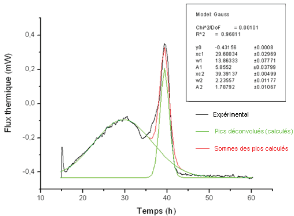
Figure 3-31 : Déconvolution du thermogramme de la synthèse en isotherme avec les valeurs de centre ( X_c ), largeur ( w ) et aire ( A ) (expérience 13)
