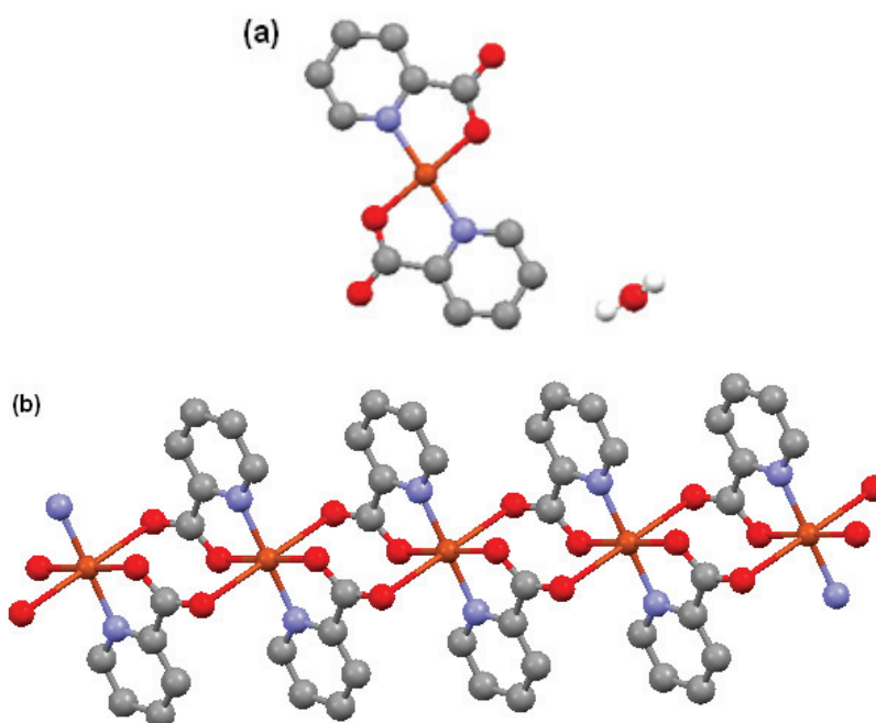
Figure 5-30 : Représentations de : (a) l'unité asymétrique de [[\text{Cu}^{\text{II}}(\text{ap})_2]\cdot 2\text{H}_2\text{O}]_n et (b) la chaîne formée (cuivre : orange/oxygène : rouge/carbone : gris/ azote : bleu/ hydrogène : blanc)
