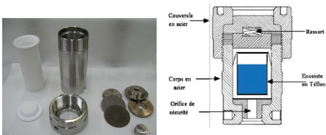
Figure 2-3 : Matériels nécessaires pour la synthèse solvothermale (téflon et autoclave)
