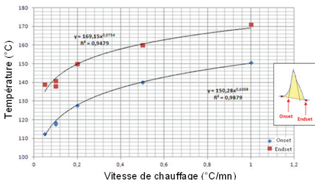
Figure 3-32 : Domaine de réaction et de cristallisation en fonction de la vitesse de chauffage
