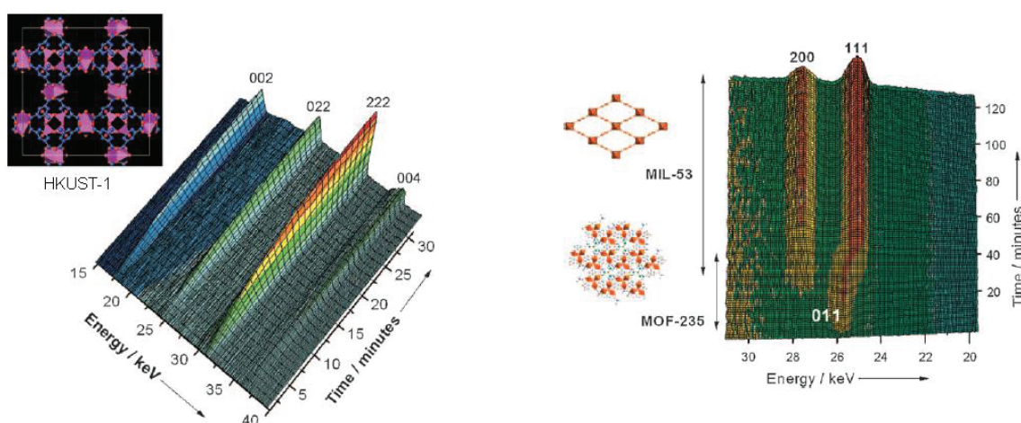
Figure 1-15 : Mesures EDXRD réalisées pendant la cristallisation du HKUST-1 à 125°C (g) et du MIL-53 à 150°C (d) 2
