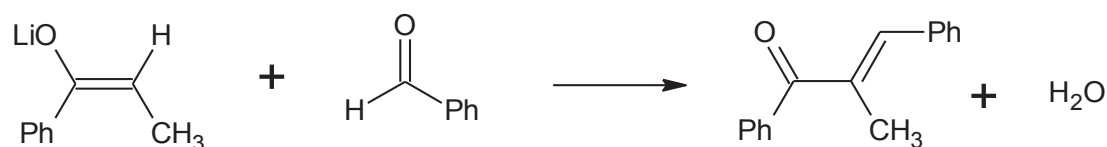
Figure 3-6 : Condensation d'aldol
