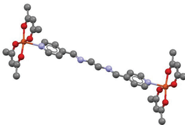
Figure 5-9 : Représentation de [\text{Cu}^{\text{II}}(\text{ped})(\text{acac})_2] (cuivre : orange/oxygène : rouge/carbone : gris/ azote : bleu)
