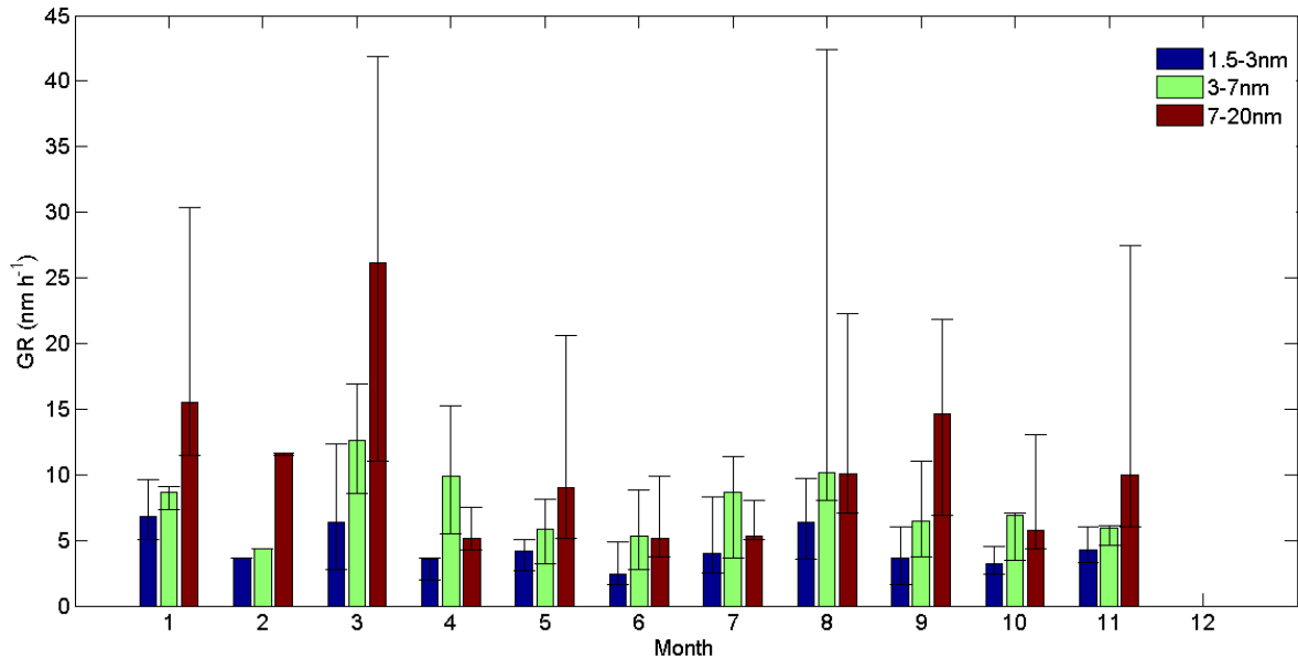
Figure 4-10 Variations mensuelles du taux de croissance médian des particules pour les trois intervalles de diamètres 1.5-3 nm, 3-7 nm et 7-20 nm pour les événements simples et les événements placés en première position lors d'événements multiples. Les extrémités inférieure et supérieure des barres d'erreurs correspondent au premier et troisième quartile, respectivement.
