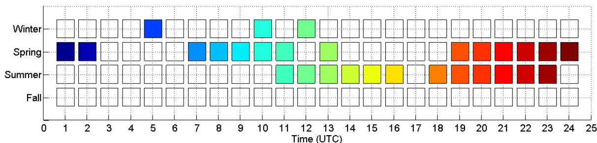
Figure 5-7 Résultat du test de Mann - Whitney appliqué aux diamètres du mode des embryons négatifs obtenus les jours avec et sans évènement de FNP séparément pour chaque saison. Les carrés sont colorés lorsque pour l'heure correspondante l'hypothèse nulle d'échantillons présentant des médianes différentes ne peut être rejetée avec un seuil de 5%.
