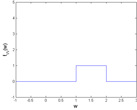
FIGURE 1.1.: Densité de W \sim \mathcal{U}_{[1,2]}
