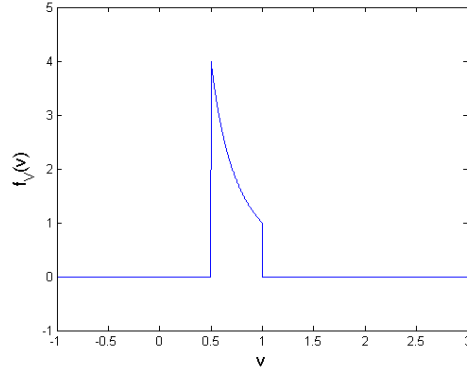
FIGURE 1.2.: Densité de V = \frac{1}{W}
