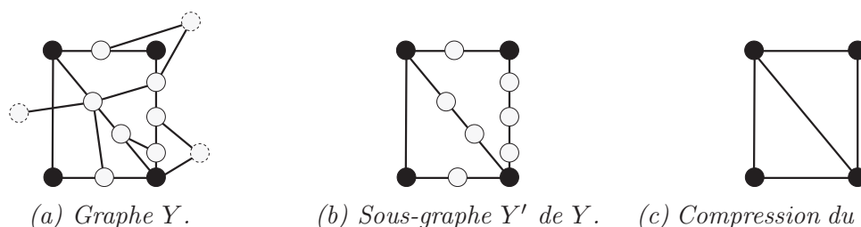
FIGURE 1.8 – Exemple de compression de graphe effectuée par TSMiner (inspiré de [68]). Les sommets noirs représentent les sommets externes d'un ensemble de chemins indépendants tandis que les sommets blancs à bord plein en sont les sommets internes. Les trois sommets de Y dont les contours sont en pointillés ne font pas partie de l'ensemble de chemins indépendants.
