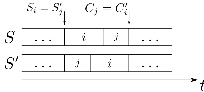
FIGURE 11 – Ordonnancements S et S'
