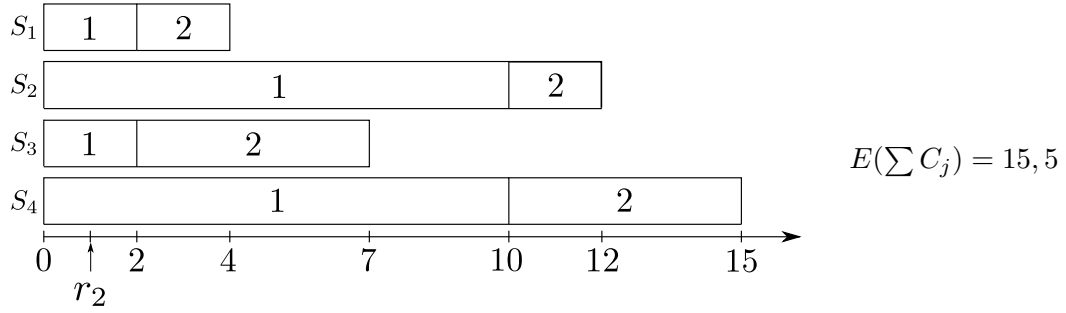
FIGURE 2 – Ordre de priorité \{1, 2\} dans la classe des politiques statiques ou dynamiques, avec ou sans préemption, ou ordre de priorité \{2, 1\} dans la classe des politiques statiques ou dynamiques sans préemption
