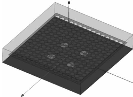
Figure 22 Structure d'une antenne à cavité FP excitée par un réseau de patchs circulaires [39]
