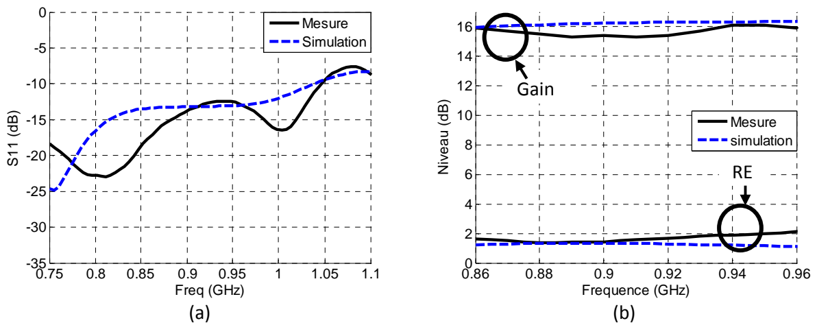
Figure 61 Module du coefficient de réflexion(a), gain et rapport d'ellipticité en fonction de la fréquence (b) pour (\varphi=\theta=0^\circ)
