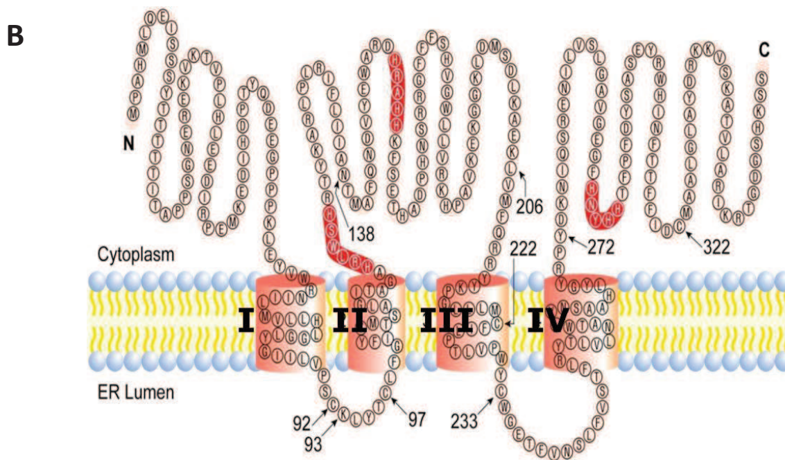
Figure 12 : Réaction enzymatique et représentation schématique de la SCD1.
