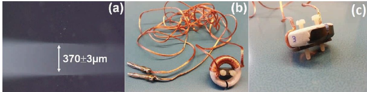
Figure III. 6 (a) Cliché de l'entrefer en microscopie inversée pour déterminer sa largeur. (b) et (c) Photographies de l'inducteur prêt à être utilisé.
