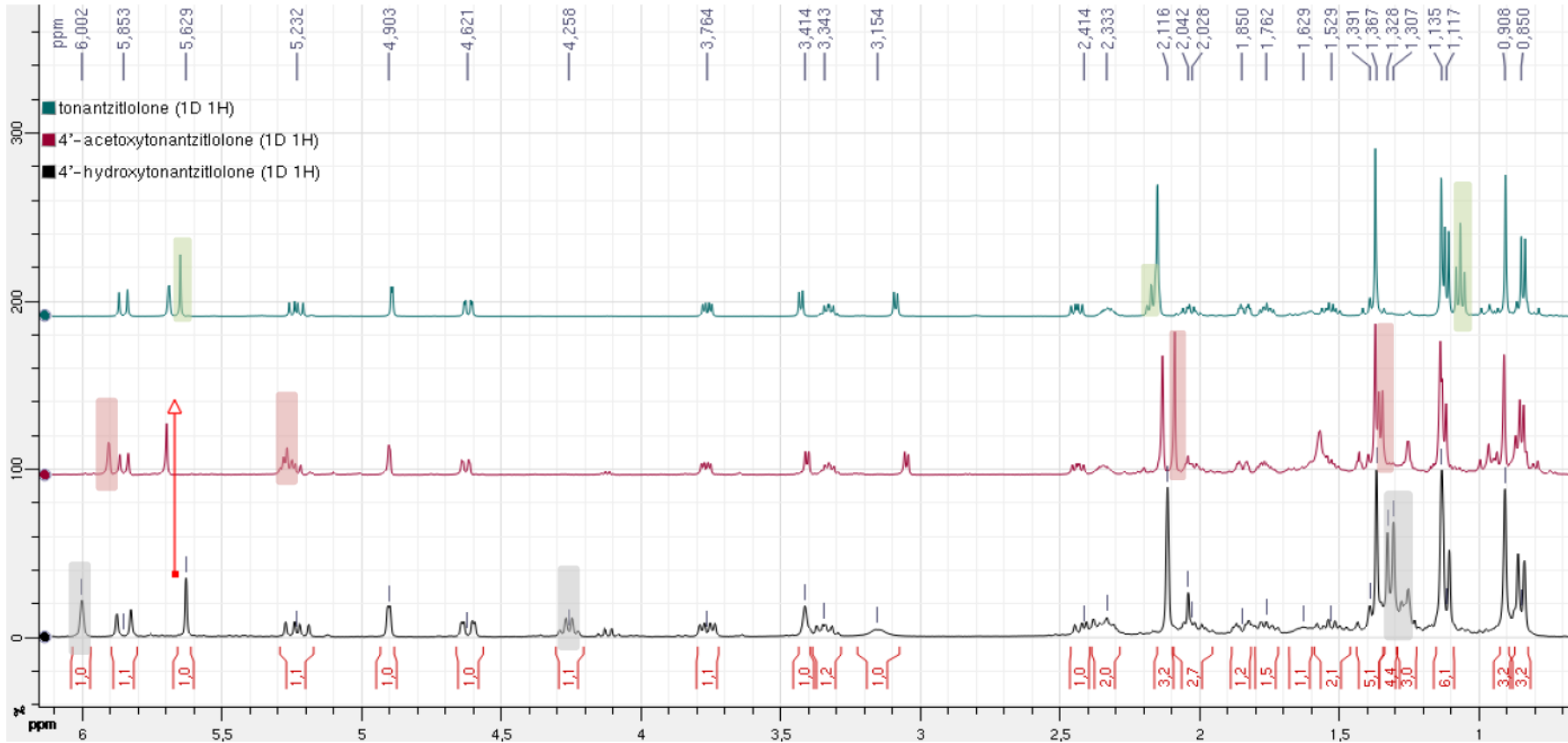
Figure 50 : Spectre RMN ^1\text{H} de la 4'-hydroxytonantzitlone ( \text{CDCl}_3 - 300 MHz) et comparaison avec les spectres RMN ^1\text{H} de la tonantzitlone et de la 4'-acétoxytonantzitlone
