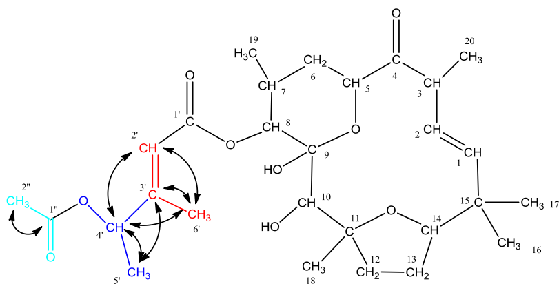
Figure 49 : Corrélations HMBC de la chaîne latérale de la 4'-acétoxytonantzitlolone
