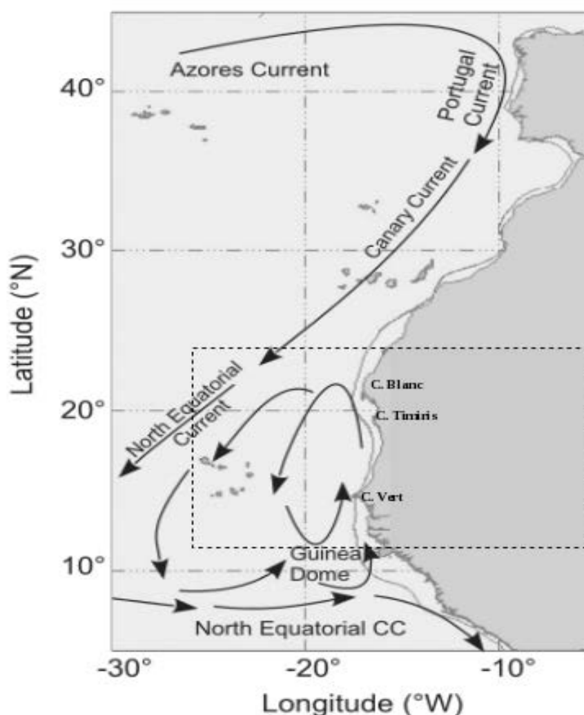
Figure 1.5 – Carte schématisée de la zone d'étude (cadre en tireté), incluant la péninsule Ibérique et la région d'upwelling Nord-Ouest Africaine et ces principaux courants de surface : les courants des Açores et du Portugal, le Courant Nord Equatorial et le Contre Courant Nord Equatorial. L'isobathe 200 m est indiqué en ligne continue. (adaptée de, Benazzouz et al., 2014).
