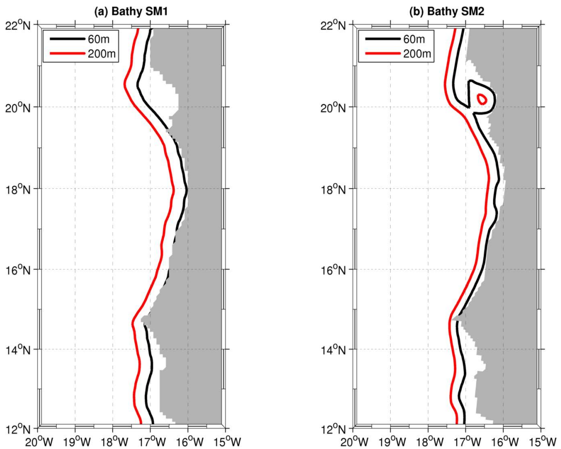
Figure A.1 – Profile spatiale de Bathymetrie pour les configurations ROMS (a) SM1 and (b) SM2 (right). Les isobathes 60m (ligne en noire) et 200 m (rouge) sont superposées. La cavité dans SM2.
