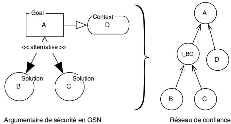
FIGURE 3.26 – Inférence mixte2
