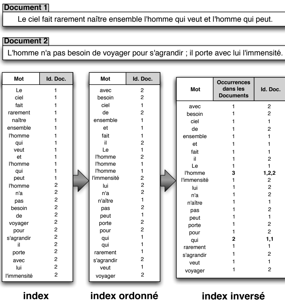
FIGURE 1 – Exemple adapté de (Manning et al., 2008) d'un index inversé constitué depuis un corpus de deux documents (deux citations de François René de Chateaubriand, Extraits de "Mémoires d'outre-tombe" pour le document 1 et de "De la restauration et la monarchie élective" pour le document 2).
