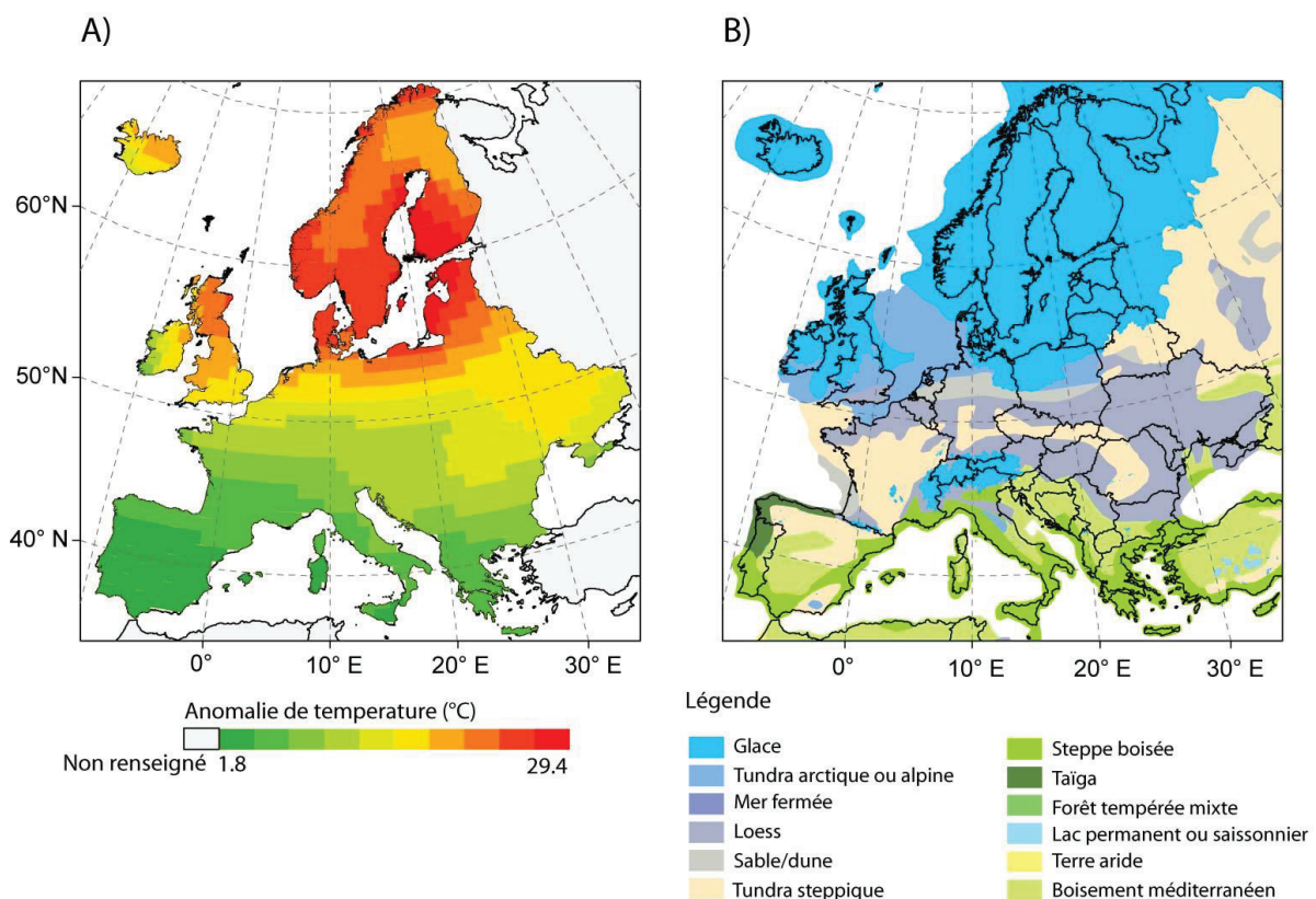
Figure 6 Cartes illustrant les conditions climatiques du dernier maximum glaciaire (-20 000 ans). A) L'anomalie de température (différence entre les températures actuelles et celles estimées lors du dernier maximum glaciaire) est un prédicteur de la variabilité climatique au cours du Pléistocène (Araújo et al. 2008 ; Leprieur et al. 2011). B) Carte de la couverture paysagère lors du dernier maximum glaciaire permettant de voir notamment l'étendue des glaciers (en bleu), (carte réalisée à
