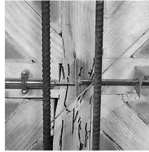
(b) Dû au cisaillement : rupture dans le bois au niveau de la connexion centrale
