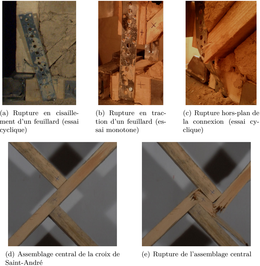
FIGURE 6.11 – Les différents modes de ruptures observés dans les assemblages au cours des essais sur cellule élémentaire
