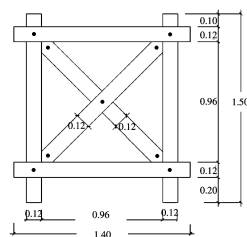
(b) Dimensions de la structure
