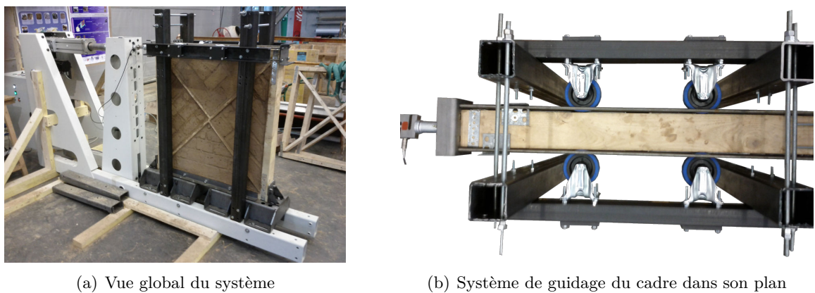
FIGURE 6.2 – Seconde étape de la conception du « mini-mur »
