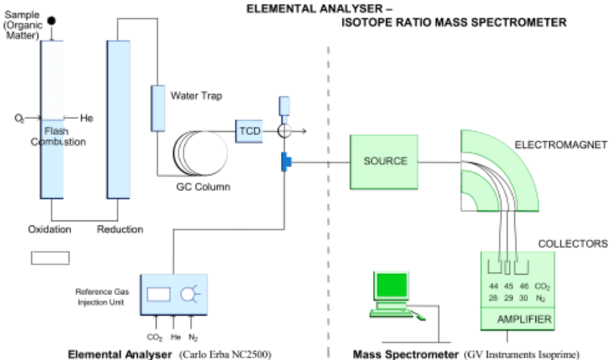
Figure II.14: Schéma de l'analyseur élémentaire couplé à un spectromètre de masse (K. Charlier).
