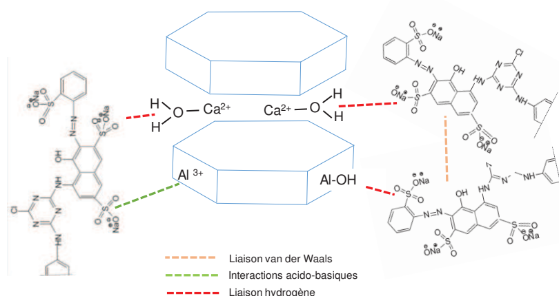
Figure 57 : Schéma d'adsorption du colorant RR 120 sur un feuillet de smectite.
