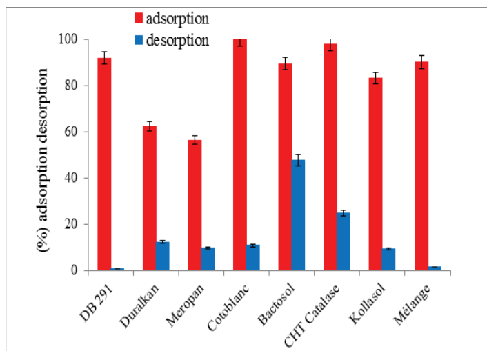
Figure 43 : Pourcentages d'adsorption et de désorption de DB 291 pour l'argile de Fouchana, en fonction des additifs
