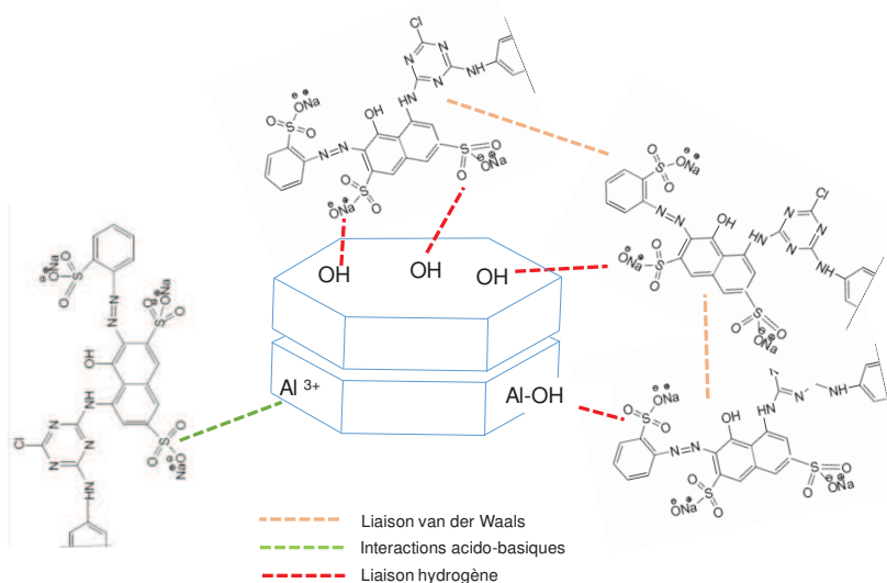
Figure 58 : Schéma d'adsorption du colorant RR 120 sur un feuillet de kaolinite
