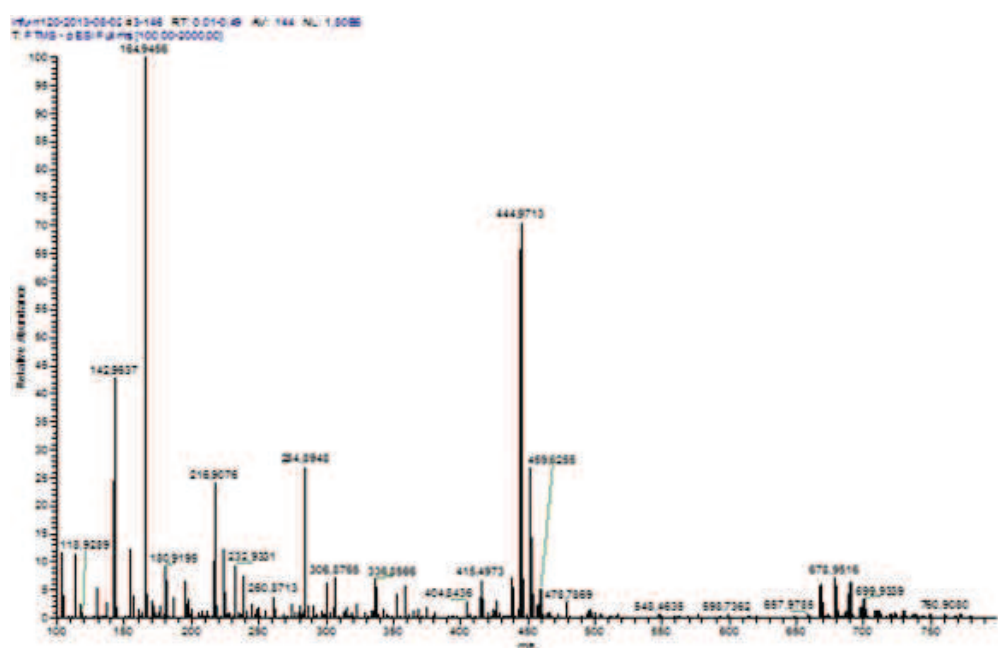
Figure 14 : Spectre de masse du surnageant RR 120 en mode négatif et en solution acide
