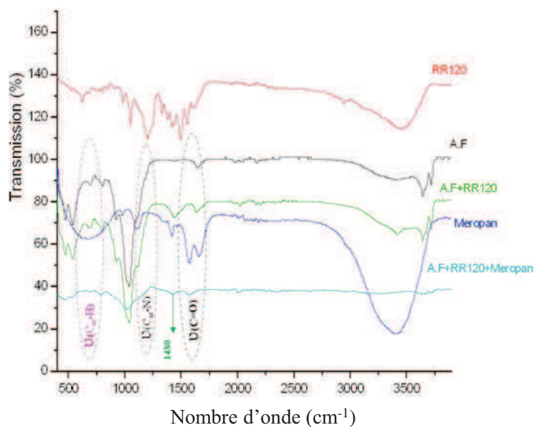
Figure 56 d : Spectre IR de RR 120, de Meropan et de l'argile de Fouchana avant et après adsorption de RR120
