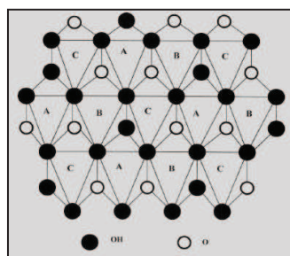
Figure 3 : Projection d'une couche octaédrique idéale d'un minéral de type 1/1 montrant la position des atomes d'oxygène et des groupements hydroxyles des différents sites octaédriques (Driests et Tchoubar, 1990)
