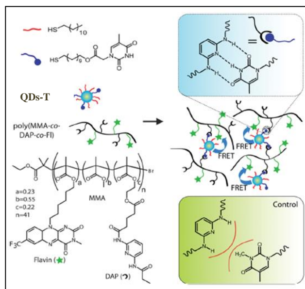
Figure 1.46: Auto-assemblage entre les QDs-T et le poly(MMA- co -DAP- co -FI). 133
