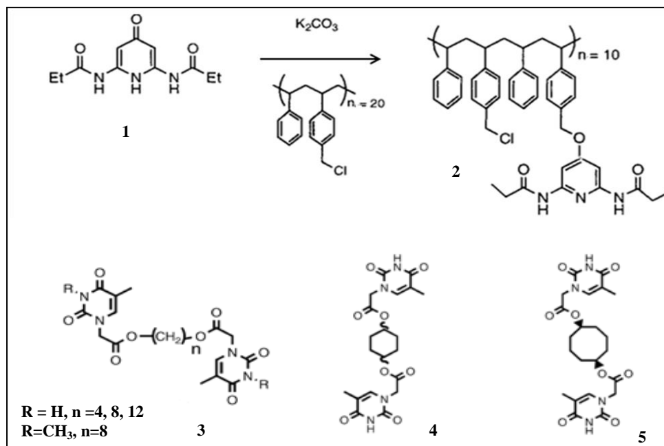
Figure 1.36: Structures du (1) 2,6-dipropionamidopyridin-4-one, (2) du copolymère statistique poly( S-co-CMS ) modifié par le motif DAP, (3,4,5) des molécules di-fonctionnalisées par le motif thymine. 114
