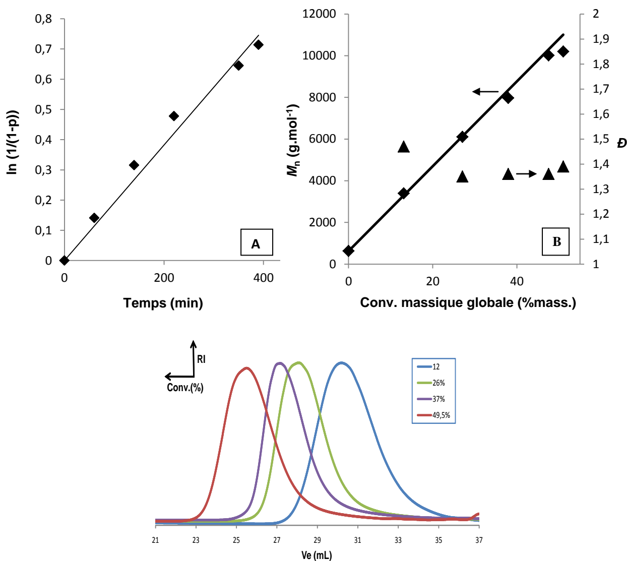
Figure 2.20: (A) Evolution de la conversion globale molaire logarithmique en fonction du temps, (B) évolution de la masse molaire moyenne en nombre expérimentale ( \blacklozenge ), de la dispersité ( \blacktriangle ) et de la masse molaire moyenne en nombre théorique (-) en fonction de la conversion globale massique (CES THF, calibration PS), (C) évolution des chromatogrammes d'exclusion stérique (CES THF, calibration PS) lors de la copolymérisation du S et du VDM amorcée par la MAMA-DAD à 110°C dans du toluène anhydre.
