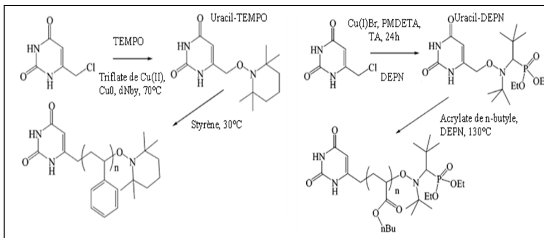
Figure 1.37: Stratégies de synthèse des amorceurs Uracil-TEMPO, Uracil-DEPN et des polymères fonctionnels PS et PABu. 116
