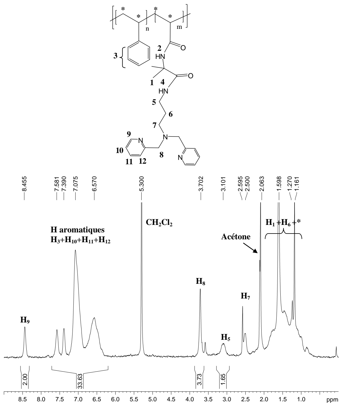
Figure A.7: Spectre RMN ^1\text{H} du poly(S- co -VDM modifiés par la DiPPA)-DAD P 13 , (200 MHz, CH 2 Cl 2 ).
