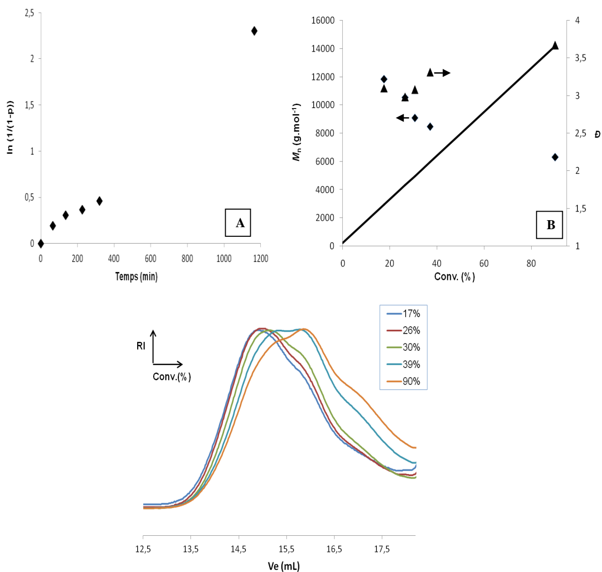
Figure 4.4: (A) Evolution de la conversion logarithmique au cours du temps, (B) évolution de la masse molaire moyenne en nombre expérimentale ( \blacklozenge ), de la dispersité ( \blacktriangle ) et de la masse molaire moyenne en nombre théorique (-) en fonction de la conversion, (C) évolution des chromatogrammes d'exclusion stérique (CES THF, calibration PMMA) lors de l'ATRP du MMA en solution dans le DPE à 60°C amorcée par le MBP en présence de nanoparticules hybrides de \text{SiO}_2@OH@poly(S-co-CMS) modifiés par la DiPA) partiellement protégées par le TMES ( G_6 ).
