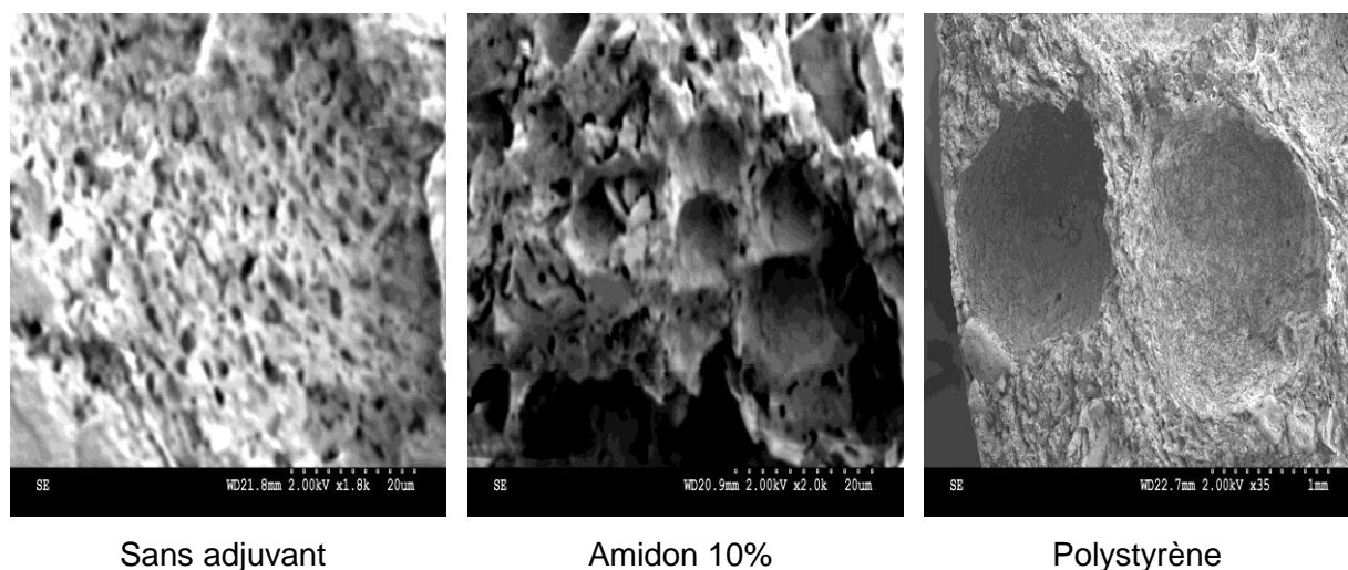
Figure 4.14. Observation microscopique des éprouvettes par MEB
