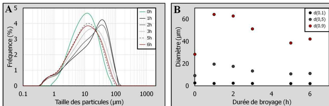
Figure III. 15 : Influence de la durée de broyage sur A- la répartition granulométrique et B- les diamètres d(0,1) , d(0,5) et d(0,9) de la suspension \text{K}_{100}\text{D}_{0,2} en présence de trois corps broyant de 26 mm de diamètre
