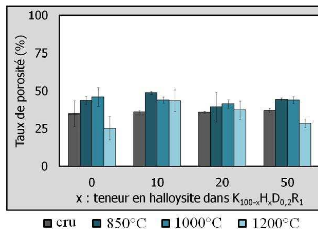
Figure IV. 20 : Influence de la teneur en halloysite et de la température de traitement thermique sur le taux de porosité des bandes K_{100-x}H_xD_{0,2}R_1
