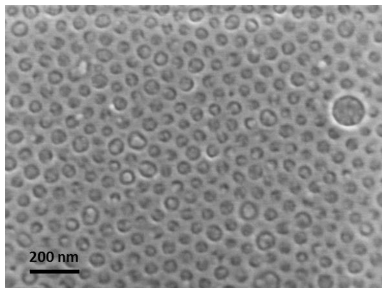
Figure 138 : Cliché MEB de NC09-Ox400 obtenu avec un MEB équipé avec un détecteur In-lens travaillant à 1 kV et une distance de travail WD = 3,1 mm.
