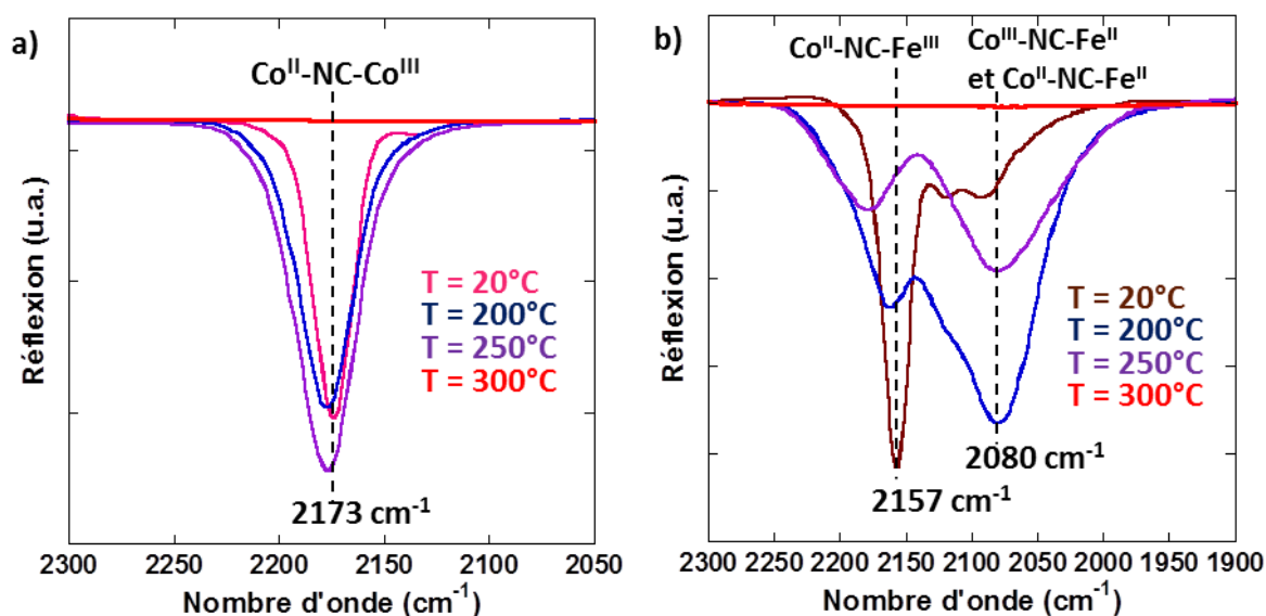
Figure 37 : Spectres Infra-rouge, sur la gamme de vibration des cyanures, avant et après calcination à 20, 200, 250 et 300°C de a) CoCo et b) CoFe .
