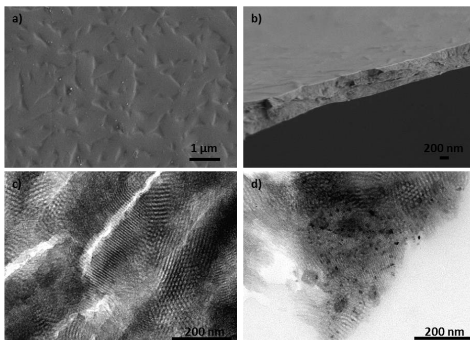
Figure 31 : Clichés MEB du film mince de silice mésoporeuse contenant les ions \text{Co}^{2+} : a) vu du dessus et b) vu de la tranche. Clichés MET microtomés c) du film mince de silice mésoporeuse contenant les ions \text{Co}^{2+} et d) du nanocomposite ABP \text{RbCoFe} /Film de silice mésoporeuse. D'après la référence [61].
