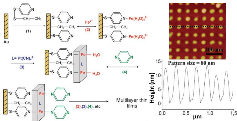
Figure 25 : Schéma de la méthode de croissance couche-par-couche d'un film de clathrates FePt et image AFM avec son profil de hauteur de plots FePt ainsi obtenus. D'après la référence [73].
