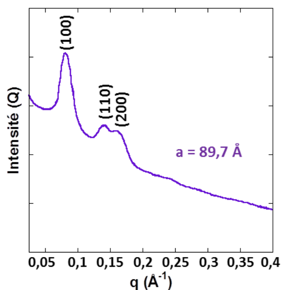
Figure 104 : Diffractogramme des rayons X aux petits angles de Mono CoFe-Ox500f-Red700 .
