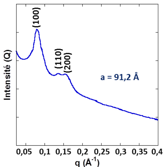
Figure 107 : Diffractogramme des rayons X aux petits angles de Mono CoFe-Ox500f-Red600 .
