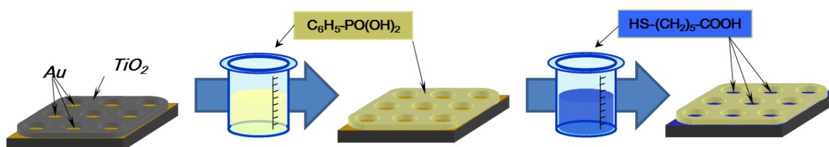
Figure 111 : Schéma des étapes de fonctionnalisation sélective des surfaces de TiO_2 et d'or (étape 4).
