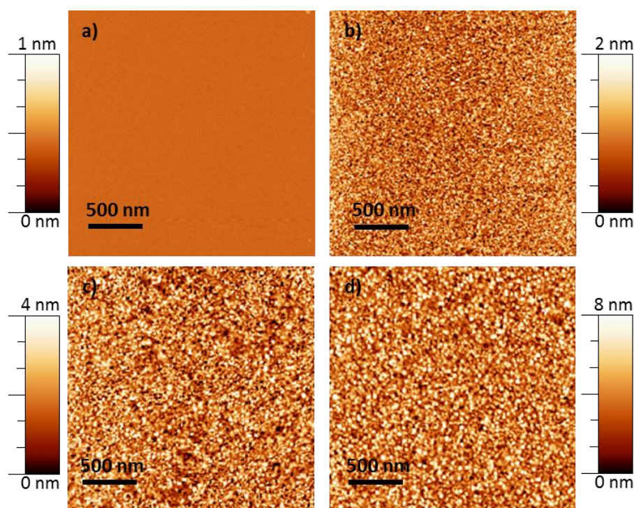
Figure 120 : Images AFM a) du substrat de Si, b) de Au10 , c) de Au20 and d) de Au50 .
