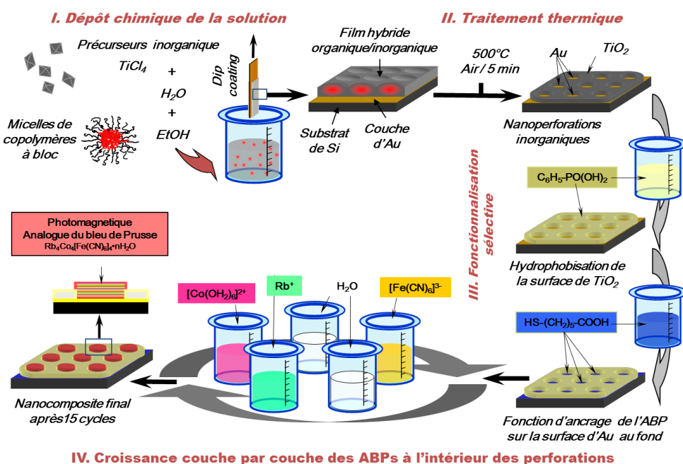
Figure 27 : Croissance couche-par-couche de l'ABP \text{RbCoFe} dans les nanoporeux d'un film mince de \text{TiO}_2 . D'après la référence [34].
