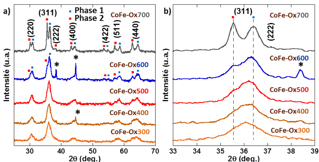
Figure 44 : Diffractogrammes de CoFe-Ox300 , CoFe-Ox400 , CoFe-Ox500 , CoFe-Ox600 et CoFe-Ox700 a) entre 30 et 70° puis b) agrandissement autour du pic (311) des structures spinelles. Les pics du support en aluminium sont marqués d'un astérisque (*) lorsqu'ils ont été observés.
