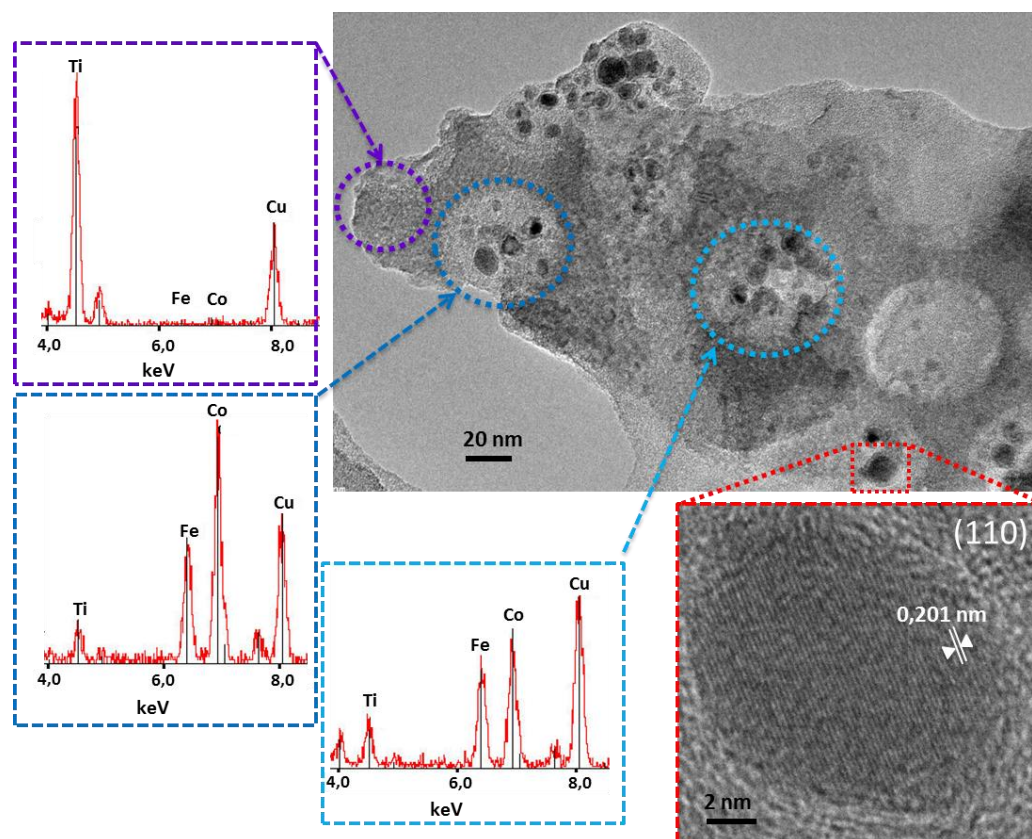
Figure 140 : Clichés MET-EDS de NC09-Red400 et images EDX réalisées à l'endroit des cercles pointillés.
