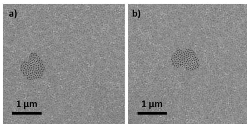
Figure 123 : Clichés MEB des échantillons a) Au20NC et b) Au50NC . Les images MEB ont été obtenues avec un MEB équipé d'un détecteur In-Lens travaillant à 1 kV et une distance de travail WD = 3,3 \text{ mm} .
