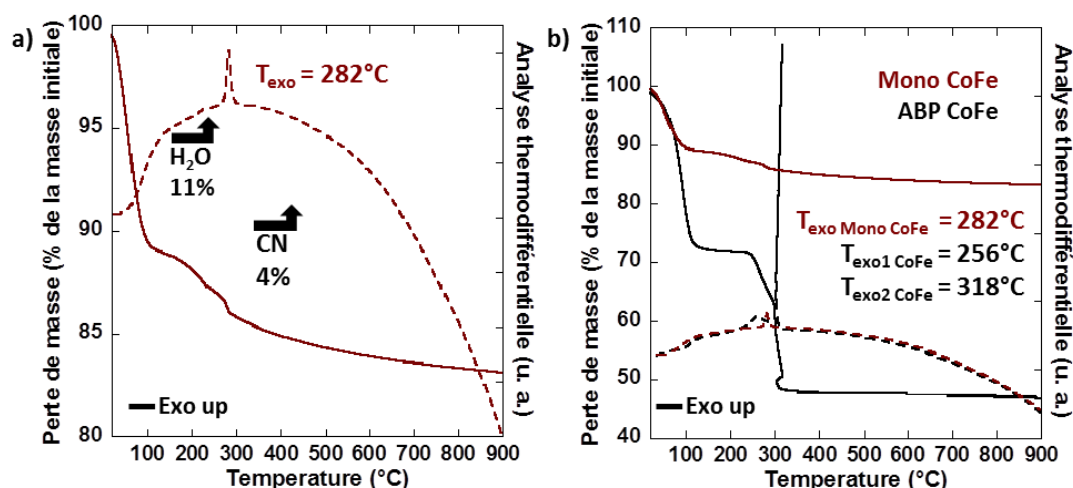
Figure 85 : Analyses thermogravimétriques et thermogravimétriques sous air avec une montée de 5°C/min de a) Mono CoFe et b) comparaison avec CoFe .
