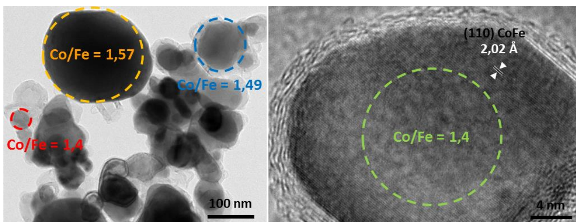
Figure 60 : Images MET-HR et mesures EDX de CoFe-Met700 .
