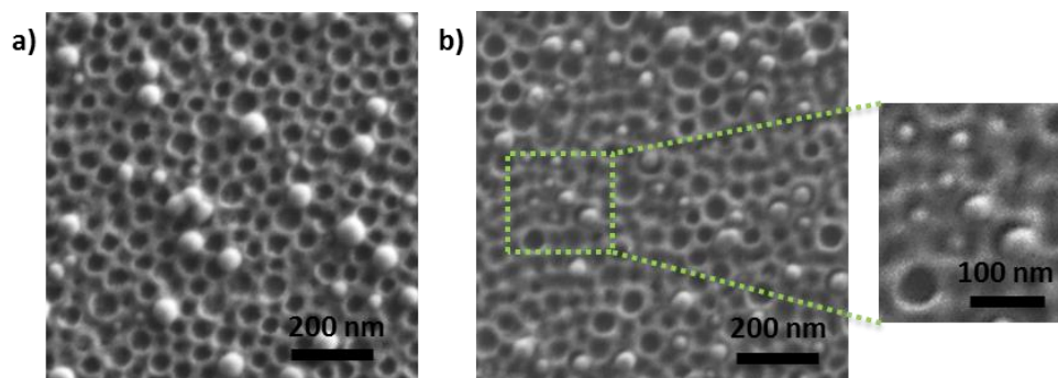
Figure 132 : Clichés MEB de a) NC07 et b) NC08 . Les images MEB ont été obtenues avec un MEB équipé d'un détecteur SE2 travaillant à 1 kV et une distance de travail WD = 3,1 mm.
