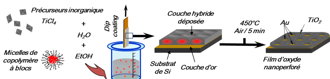
Figure 110 : Schéma de l'élaboration de la couche de TiO_2 nanoporeuse (étapes 2 et 3).
