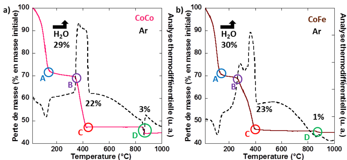
Figure 156 : Courbes d'analyse thermique sous Ar de a) CoCo et b) CoFe . Les courbes de perte de masse sont représentées en trait plein et les analyses thermodifférentielles en pointillé.
