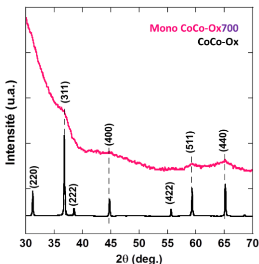
Figure 79 : Diffractogrammes des rayons X de Mono CoCo-Ox700 et CoCo-Ox700 .
