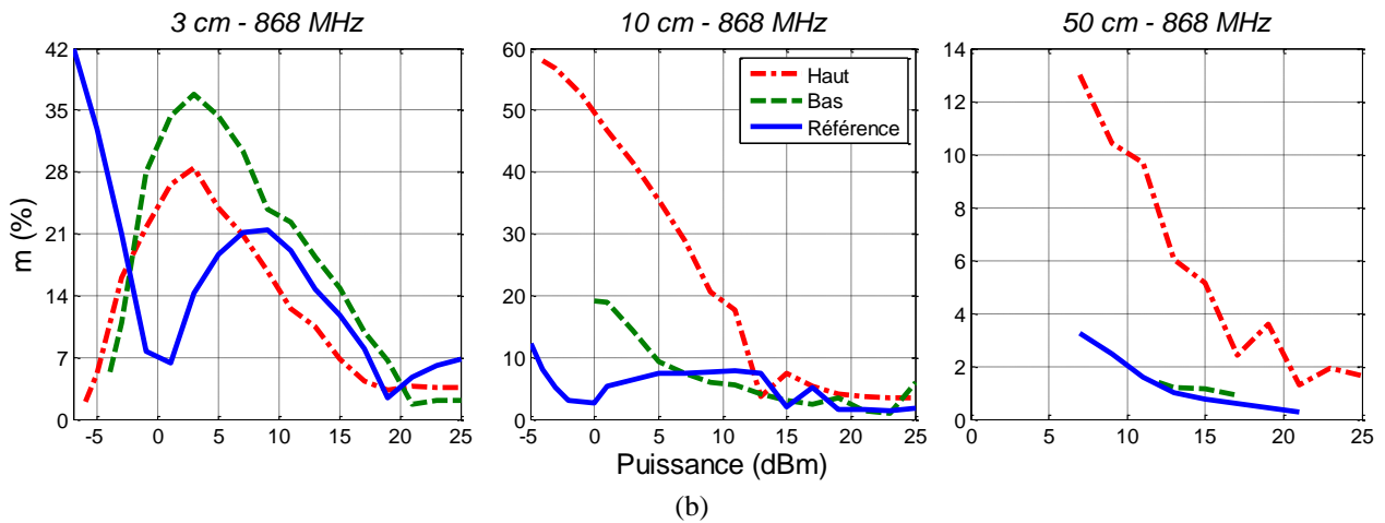
Fig. 3-33 – Indice de modulation des tags à (a) 865 MHz et à (b) 868 MHz.
