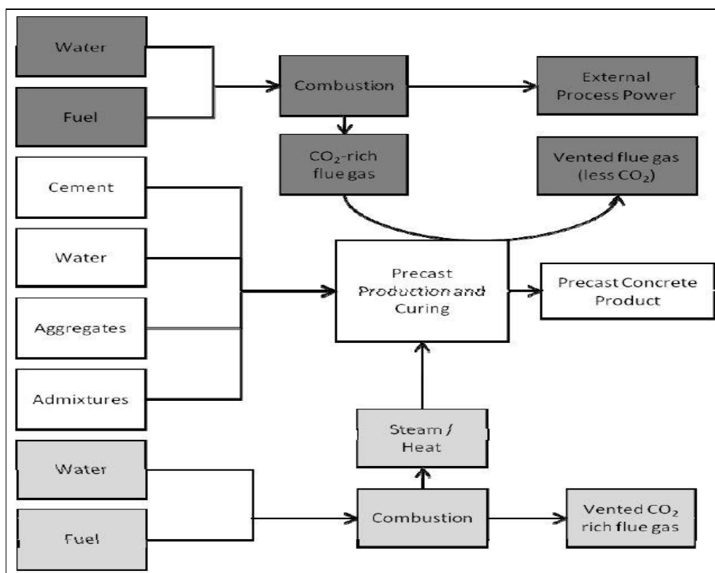
Figure 24. Diagrammes de blocs de Carbon Sence Solutions Inc du processus de durcissement de béton de CO2 accélérée (en haut, éclos) et le processus de durcissement à la vapeur conventionnelle (en bas, foncé). Les deux processus partagent le processus de production de béton commune (au milieu, pas de remplissage) [110].
