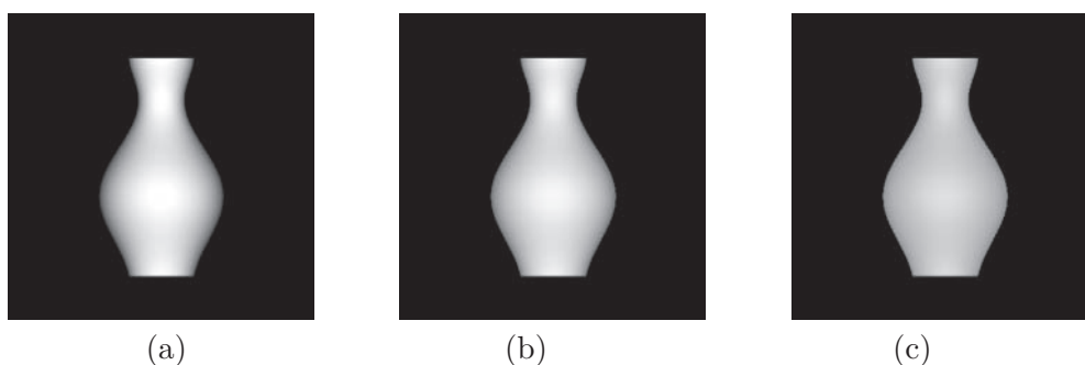
FIGURE 6.15 – Images de synthèse d'un vase texturé, calculées avec le modèle d'Oren-Nayar (6.6) : (a) \sigma = 0 (modèle lambertien); (b) \sigma = 0,25 ; (c) \sigma = 0,5 . Plus la valeur de \sigma est élevée, plus le relief semble aplati.
