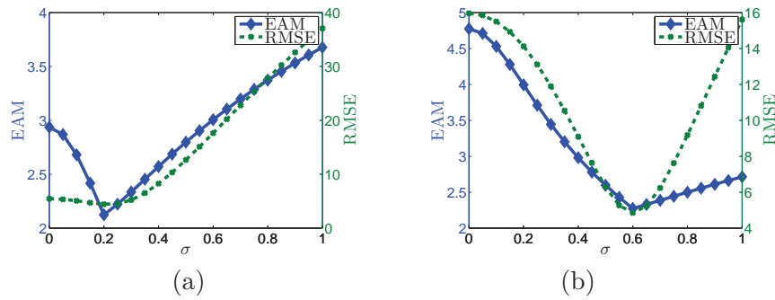
FIGURE 6.17 – Pour estimer la rugosité, il suffit d’utiliser le schéma itératif (6.9) pour différentes valeurs de \sigma , et de sélectionner l’estimation qui minimise la RMSE entre les images reprojctées et les images d’origine. On constate sur ces deux graphes que la RMSE est minimale pour une valeur : (a) très proche de la valeur réelle \sigma = 0, 2 ; (b) égale à la valeur réelle \sigma = 0, 6 . Nous avons également porté sur ces graphes l’évolution de l’EAM entre les champs de normales estimé et réel, en fonction de \sigma , dont le minimum coïncide parfaitement avec la valeur réelle de \sigma . L’EAM peut donc sembler plus pertinente que la RMSE pour estimer la rugosité, mais en général, l’EAM n’est pas calculable car on ne dispose pas de la vérité terrain.
