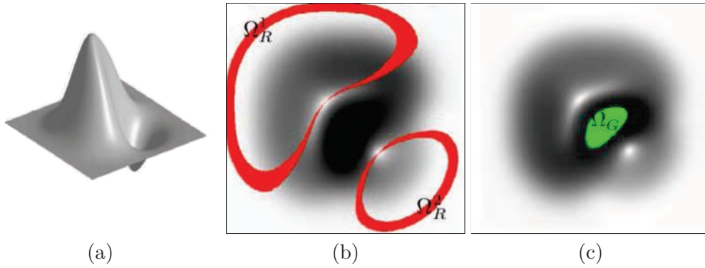
FIGURE 4.4 – Points singuliers d'une surface synthétique. (b)-(c) Deux images de synthèse de la surface lisse (a) telles que tous les points soient éclairés deux fois, sur lesquelles sont superposés les ensembles \Omega_R = \Omega_R^1 \cup \Omega_R^2 (en rouge) et \Omega_G (en vert).
