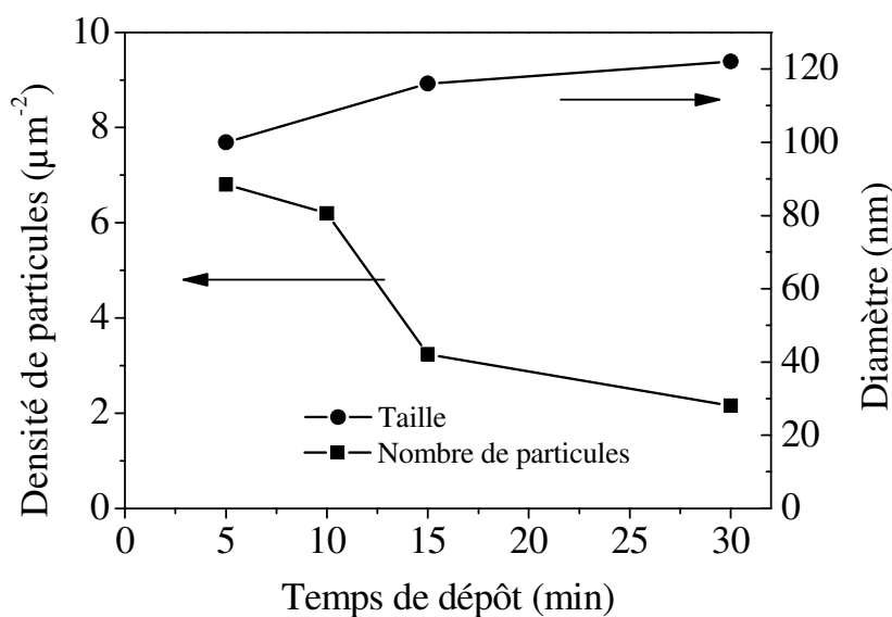
Figure 5-10. Evolution de la densité et du diamètre des particules de palladium avec le temps.
