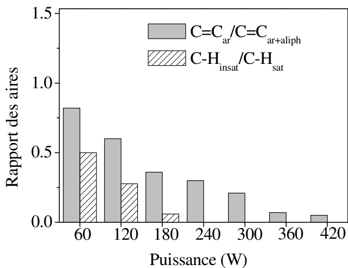
Figure 3-7. a) spectres FTIR de la polyaniline obtenue à différentes puissances ; b) rapport de bandes C=C_{ar}/C=C_{ar+aliph} (bandes pleines) et C-H_{insatsat}/C-H_{satsat} (bandes hachurées). T_{ANi}=40^{\circ}C , T_{sub}=10^{\circ}C ; t=10 min.
