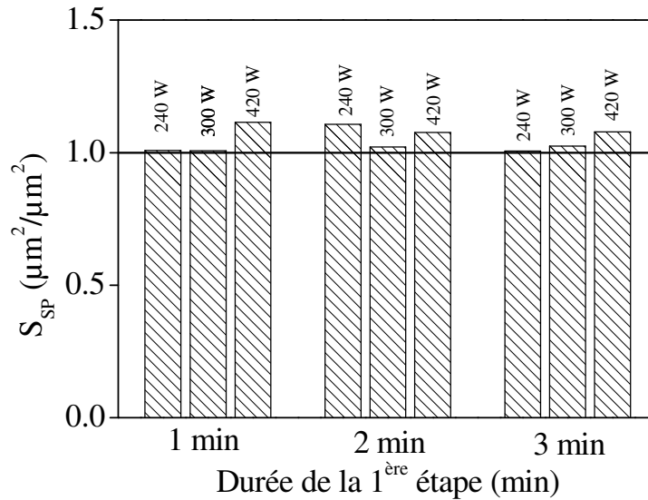
Figure 6-13. Evolution de la surface spécifique S_{\text{sp}} des couches de PANI plasma en fonction du temps de dépôt.
