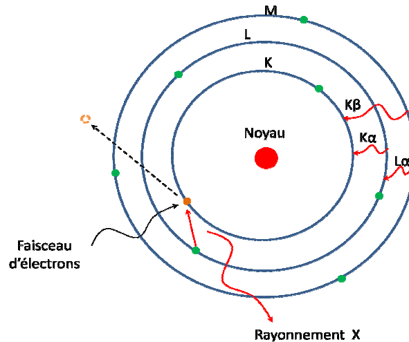
Figure 2-14. Schéma d'émission des rayons X lors de l'excitation de l'échantillon.
