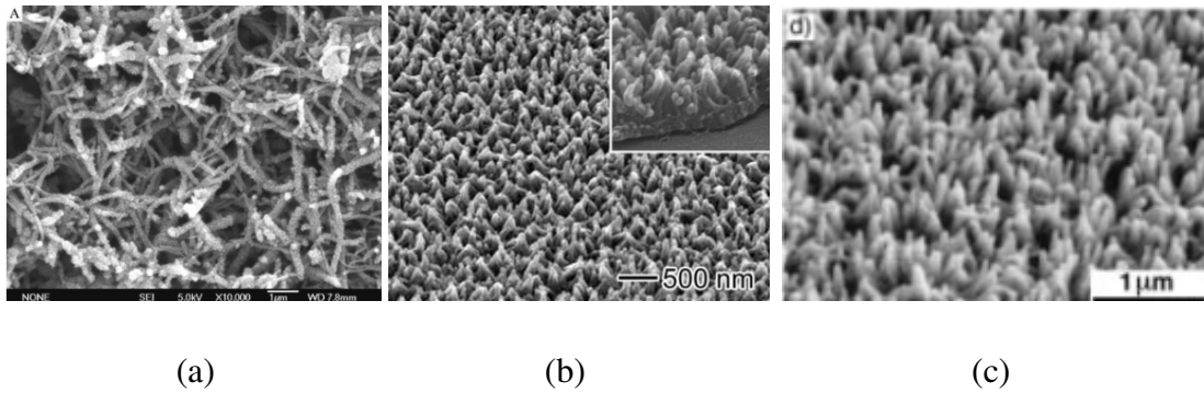
Figure 1-14. Nanostructures de PANi : a) enchevêtrées 63 ; b) ordonnées (synthèse chimique) 65 ; c) ordonnées (synthèse électrochimique) 45 .
