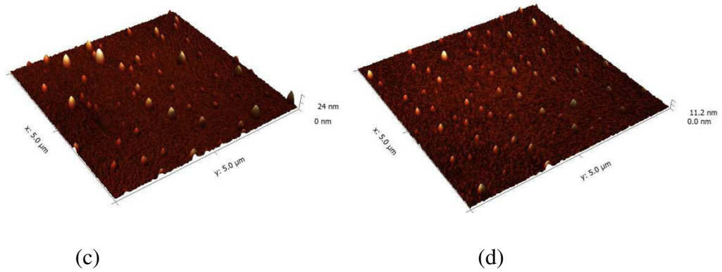
Figure 4-4. Images AFM de PANi : a) non-traitée ; b) 5 sccm ; c) 10 sccm ; d) 30 sccm. P=420 W, t=5 min.
