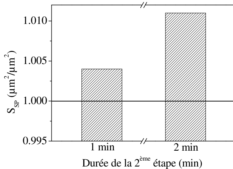
Figure 6-16. Evolution de la surface spécifique de la couche de PANI plasma en fonction du temps de dépôt de la 2 ème étape.
