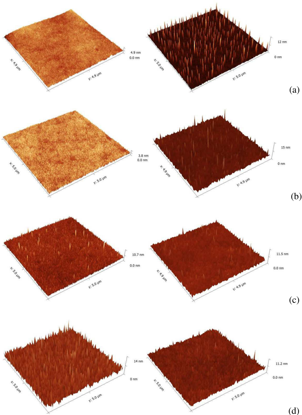
Figure 3-12. Images AFM des surfaces obtenues à P = 240 W (à gauche) et à P = 300 W (à droite) en fonction du temps de dépôt : a) 1 min ; b) 3 min ; c) 5 min ; d) 7,5 min. T_{\text{ANi}}=40^{\circ}\text{C} , T_{\text{sub}}=10^{\circ}\text{C} .
