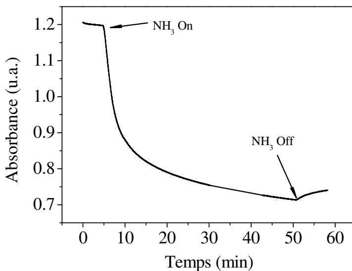
Figure 6-7. Evolution de l'absorbance d'une couche de PANi (1 min-240 W, 26 min-60 W) exposées à une concentration en NH 3 de 4618 ppm.
