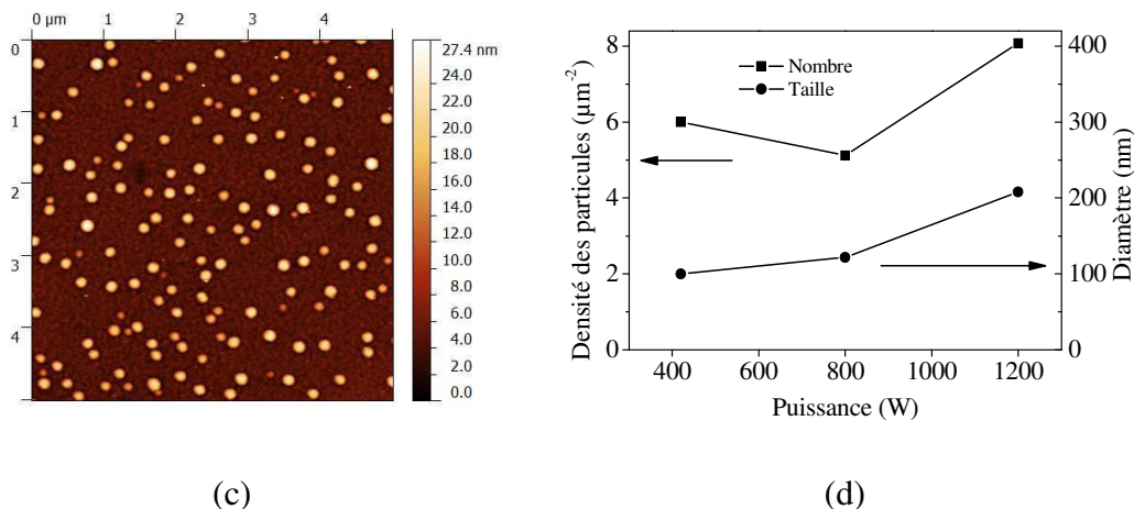
Figure 5-12. Distribution des particules du palladium sur la surface de la PANi. Q_{Ar}=5 sccm, t=5 min, U_{Pd}=-200 VDC. a) 420 W ; b) 800 W ; c) 1200 W. d) La densité et le diamètre moyen des particules en fonction de la puissance.
