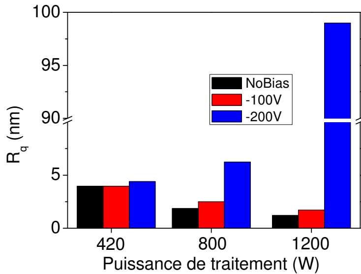
Figure 4-9. Influence de la polarisation du substrat sur la structuration de la surface. Q_{\text{ANi}}=5 sccm, t=5 min.
