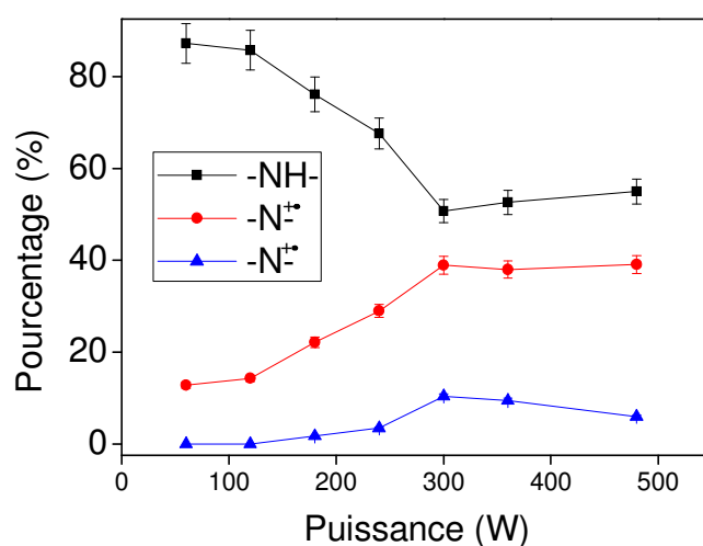
Figure 3-10. Evolution du pourcentage des sous-structures dans la décomposition des pics haute résolution : a) C1s; b) N1s. T_{ANi}=40^{\circ}C , T_{sub}=10^{\circ}C , t=10 min.
