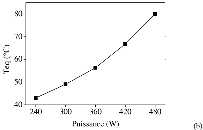
Figure 3-19. a) Evolution de la température du substrat pour différentes puissances avec le temps ; b) Température d'équilibre ( T_{eq} ) en fonction de la puissance. T_{ANi}=40^{\circ}C , T_{sub}=10^{\circ}C
