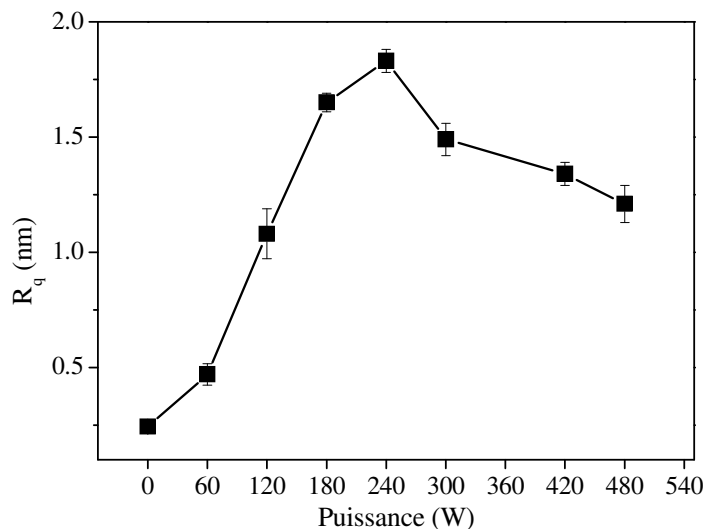
Figure 3-15. Rugosité R_q de la PANi en fonction de puissance. T_{ANi}=40^{\circ}C , T_{sub}=10^{\circ}C , t=10 min.
