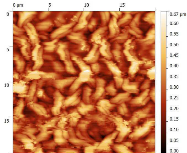
Figure 4-12. Image AFM de la surface obtenue après le traitement de la PANi à 1200 W et U_{\text{sub}} = -200 VDC.
