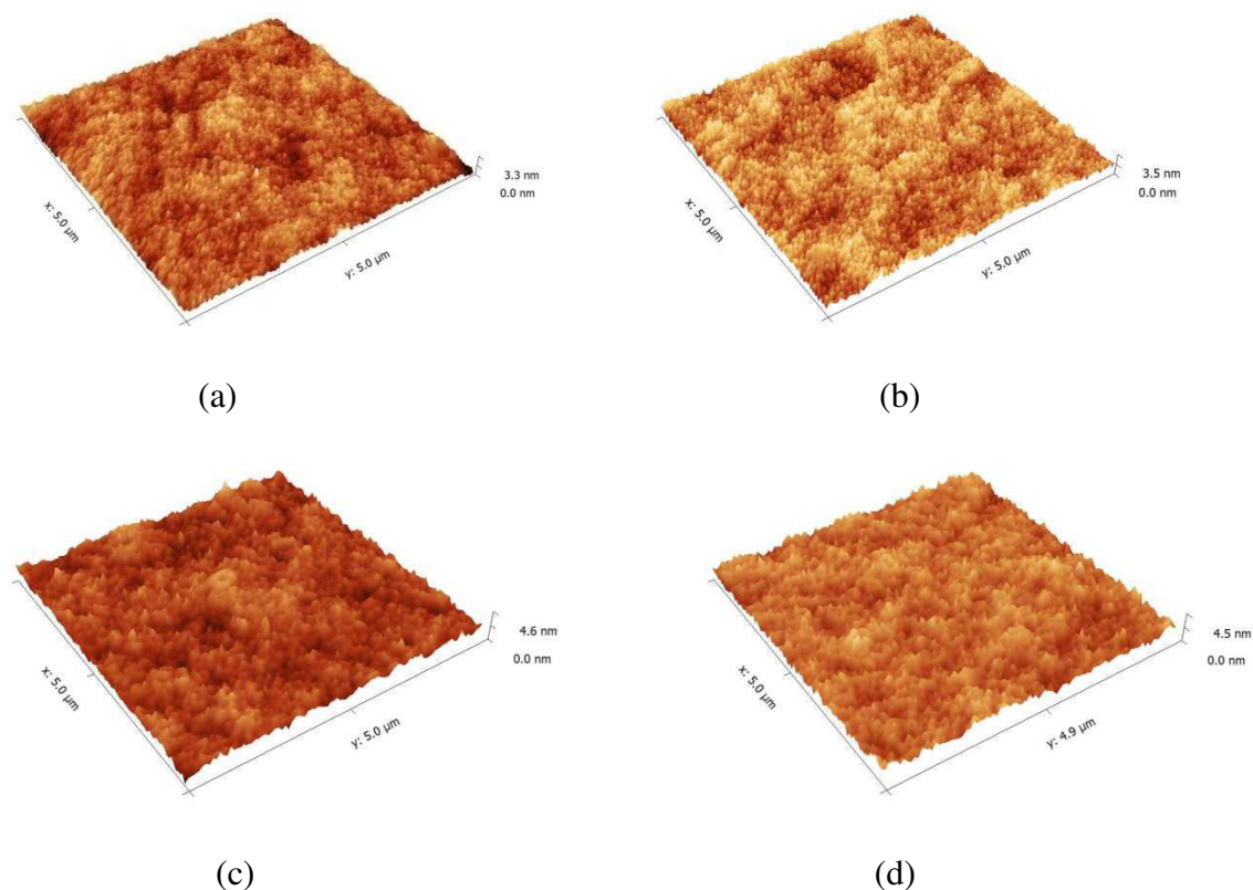
Figure 3-11. Images AFM de la polyaniline obtenue aux différentes durées de dépôt : a) 5 min ; b) 10 min ; c) 15 min ; d) 20 min. P=60 W, T_{ANi}=40^{\circ}C , T_{sub}=10^{\circ}C .
