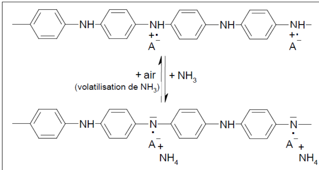
Figure 6-2. Mécanisme chimique de détection de l'ammoniac par la polyaniline.
