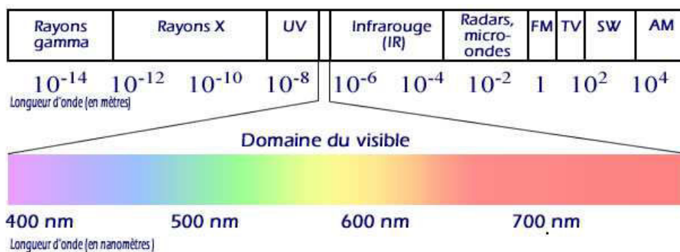
Figure 2-5. Spectre électromagnétique.
