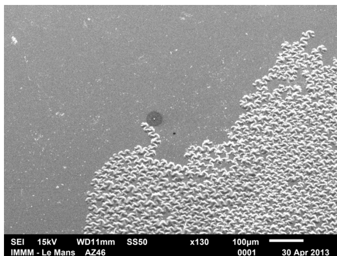
Figure 3-16. Cliché MEB caractéristique d'un dépôt instable. P=300\text{ W} , t=10\text{ min} , T_{\text{ANi}}=40^{\circ}\text{C} , T_{\text{sub}}=10^{\circ}\text{C} .
