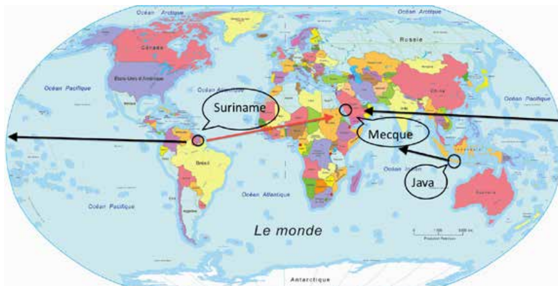
Figure 12 : Direction de la Mecque depuis Java et depuis le Suriname. La flèche rouge indique la direction de la prière pour les Musulmans surinamiens à tendance réformiste ; les flèches noires indiquent la direction que prennent les Musulmans de l'Île de Java et les Musulmans surinamiens à tendance traditionaliste javanaise, dans leur majorité descendants d'immigrants venus de cette île (LES STATS DU MONDE, 2014).
