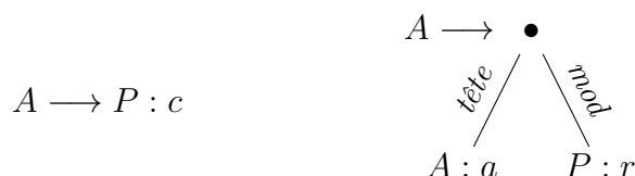
FIGURE 4.4 – Productions supplémentaires pour l’ajout de subordonnées
