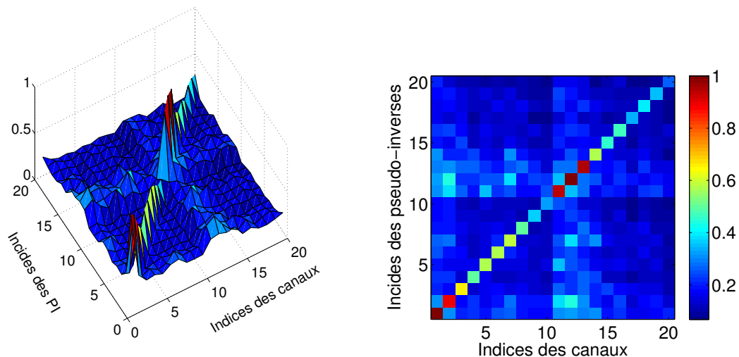
FIGURE B.3 – Niveaux de corrélations calculés entre les fonctions de transfert mesurées et les pseudo-inverses correspondants obtenus par retournement temporel.
