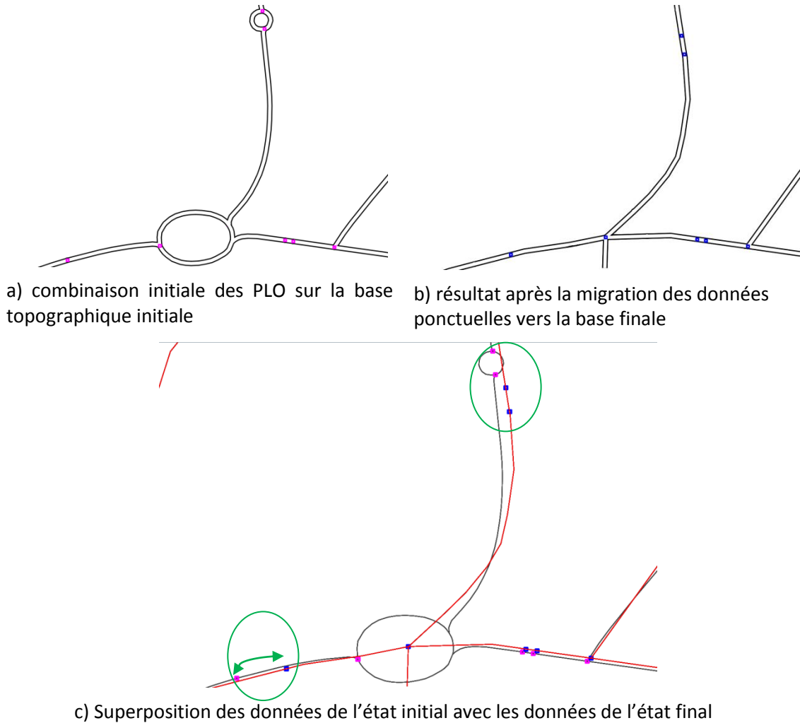
Figure 126. Exemple du cas d'un grand rond-point
