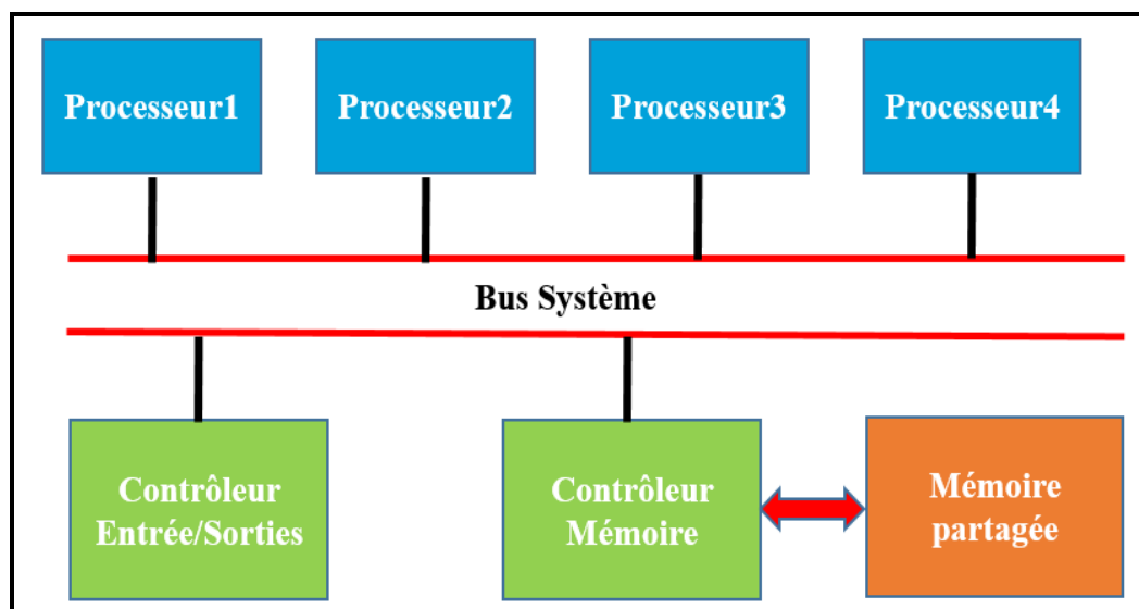
Figure 19. Architecture matérielle de base pour un SMP: exemple de machine SMP avec quatre processeurs (4 sockets sur une carte mère par exemple).
