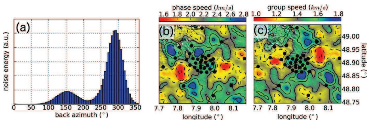
Figure III.15 : Modèles hypothétique de bruit (a) et cartes de dispersion hypothétiques des ondes de Rayleigh à 2s de période en vitesse de phase (b) et de groupe (c). Le modèle de bruit est obtenu à partir de deux gaussiennes centrées sur 290° et 150° de back-azimut et dont l'amplitude est exprimée en unités arbitraires. Les cartes de dispersion sont construites à partir de la vitesse des ondes de Rayleigh à 2s de période à laquelle on ajoute des anomalies de vitesse gaussiennes aléatoires. Les points noirs représentent les stations du réseau.
