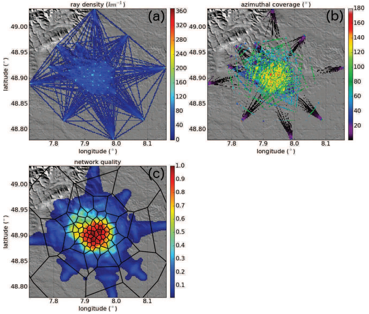
Figure III.13 : Construction d'une grille irrégulière pour la paramétrisation de la carte de dispersion des ondes de Rayleigh à une fréquence donnée. (a) : densité de rais inter-stations. L'échelle de couleur correspond à la longueur cumulée des rais traversant chaque pixel, exprimée en km/km 2 . (b) : couverture azimutale du réseau. Elle est définie par l'angle supplémentaire du plus grand gap azimutal rencontré dans chaque pixel. Un pixel croisé par un seul rai donne une couverture de 0° et un pixel croisé par des rais uniformément distribués en azimut donne une couverture proche de 180°. (c) : Combinaison (arbitraire) de la densité de rais et de la couverture azimutale pour la détermination d'un indicateur de « qualité » du réseau variant de 0 à 1. Cette fonction est utilisée pour la construction d'une grille irrégulière de Voronoï offrant une meilleure résolution dans les zones où le réseau est dense et bien couvert en azimut.
