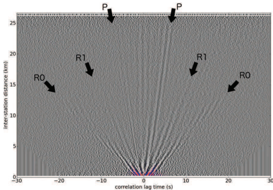
Figure V.8: Fonctions de corrélation obtenues sur le réseau EstOf. Les corrélogrammes sont regroupées par distances inter-station, moyennées par gamme de distance (à \pm 150 m), et filtrées entre 0.33s et 1.42s (0.7Hz et 3Hz). Les flèches noires marquées P, R0 et R1 indiquent trois arrivées distinctes interprétées
