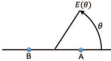
Figure 1.9 : géométrie du problème. \theta est la coordonnées polaire d'une source de bruit dans le plan horizontal et dans le référentiel de la paire de station AB. E(\theta) est la distribution azimutale de l'énergie des sources de bruit.
