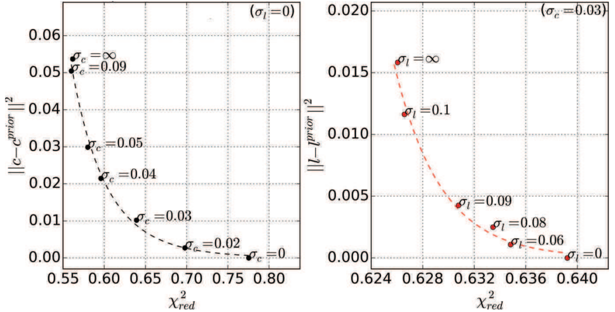
Figure III.24 : Ajustement des incertitudes a priori sur les paramètres de dispersion pour la régularisation du problème inverse à 2.5s de période. Gauche : détermination de l'incertitude a priori sur la vitesse de phase. La dérivée de la courbe de dispersion est fortement contrainte ( \sigma_l = 0 ). La valeur \sigma_c = 0.03 minimise à la fois le coût sur les données \chi_{red}^2 et la norme des écarts entre le modèle de vitesse en vitesse de phase réel et calculé \|c - c^{prior}\|^2 . Droite : détermination de l'incertitude a priori sur la dérivée de la courbe de dispersion pour une valeur de \sigma_c = 0.03 fixe. La valeur retenue pour l'incertitude a priori sur la dérivée de la courbe de dispersion est \sigma_l = 0.09 .
