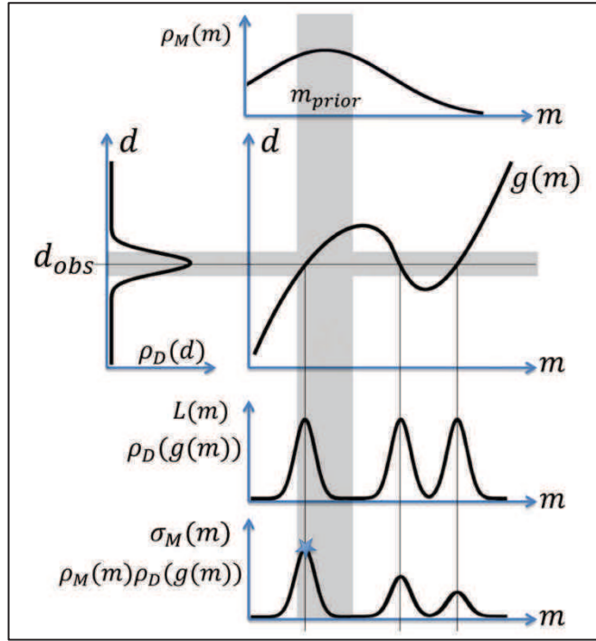
Figure III.1 : Représentation schématique de la « combinaison des états d'information » pour la résolution des problèmes inverses selon Tarantola (2005). L'axe horizontal dénommé « m » désigne l'espace des modèles. L'axe vertical « d » désigne l'espace des données. La loi g(m) est la théorie du problème inverse et relie les deux espaces, elle est supposée parfaite ici. \rho_D désigne la densité de probabilité sur l'espace des données et d_{obs} est la mesure la plus probable. \rho_M désigne la densité de probabilité a priori et m_{prior} est le modèle favori. L est la loi de vraisemblance des modèles et \sigma_M est la densité de probabilité a posteriori qui permet de déterminer les différentes solutions du problème inverse. L'étoile bleue représente le modèle qui satisfait au mieux l'ensemble des informations a priori données par \rho_D et \rho_M .
