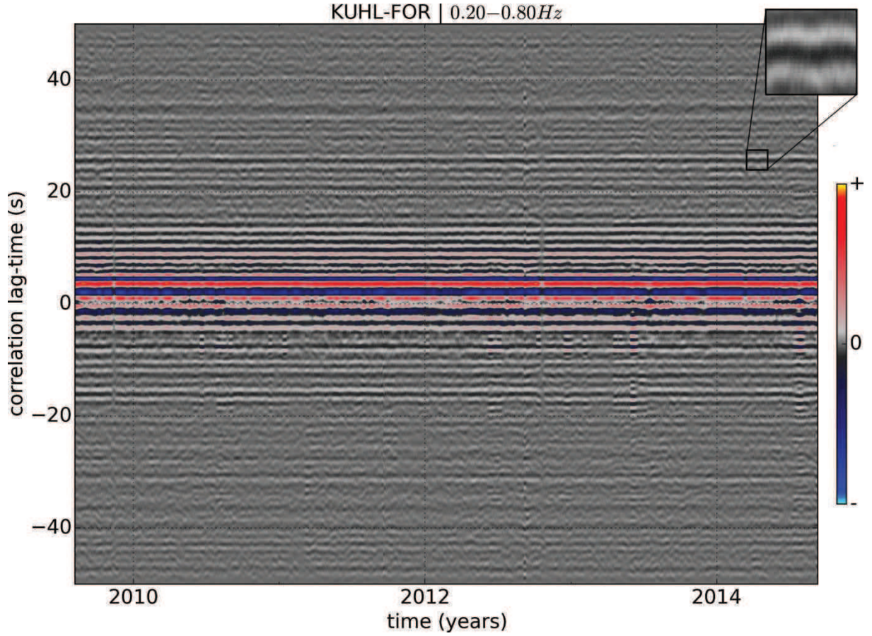
Figure IV.2 : Fonctions de corrélation de la paire de stations KUH-L et FOR du réseau permanent de Soultz-sous-Forêts, composantes verticales. Les stations sont distantes de 4.5km et l'azimut de la paire de stations est de 300°N. Les fonctions de corrélation sont moyennées sur une fenêtre glissante de largeur 10 jours avançant par pas de 1 jour. Les traces sont filtrées entre 1.25s et 5s (0.2 et 0.8Hz). Les petites instabilités de la phase (zone agrandie) sont pour la plupart causées par des petites variations des sources de bruit.
