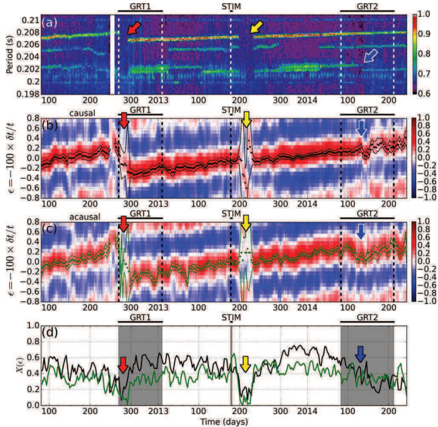
Figure IV.13 : Comparaison entre le contenu spectral des fonctions de corrélation et les mesures d'étirement de la coda de la fonction de corrélation RITT-BETS. Les fonctions de corrélation sont moyennées sur une fenêtre de 10 jours avançant par pas de 3 jours. Le signal est filtré au voisinage de la fréquence 4.8Hz selon un filtre Gaussien. La coda est définie par l'intervalle 10s – 30s après la date d'arrivée du groupe du mode fondamental de l'onde de Rayleigh. Les codas causale et acausale de référence sont obtenues en moyennant les fonctions de corrélation sur toute la période mars 2012 – septembre 2014. (a) Spectre médian de l'ensemble des fonctions de corrélation au voisinage de la période 0.207s (4.8Hz). L'échelle de couleur correspond à l'amplitude du spectre médian exprimé en unités arbitraires. (b et c) mesure d'étirement de la coda causale et acausale. L'échelle de couleur donne l'amplitude de la fonction de corrélation en étirement X(\epsilon) . Les points noirs et verts correspondent à l'évolution temporelle du coefficient d'étirement \epsilon , les lignes noires et vertes correspondent aux incertitudes sur les mesures d'étirement prédites par la formule de Weaver et al. (2011). (d) Evolution du coefficient de corrélation maximal entre la coda de référence et la coda courante pour les parties causale (courbe noire) et acausale (courbe verte). Les lignes verticales pointillées indiquent les forages de puits GRT1 et GRT2 et les stimulations chimique et hydraulique du puits GRT1 (notées STIM).
