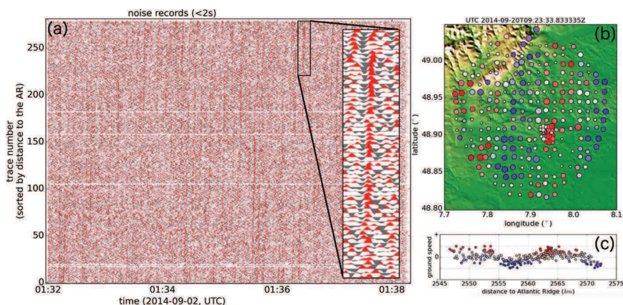
Figure V.3 : Observation du bruit de fond sismologique par le réseau EstOf au-delà de 2s de période. (a) traces sismologiques obtenues par les capteurs du réseau le 2 septembre 2014. Les traces sont filtrées à l'aide d'un filtre passe-bas de fréquence coin 0.5Hz, normalisées par leur écart type et triées en fonction de la distance du capteur à la dorsale médio-Atlantique (à l'ouest). On distingue des arrivées cohérentes très répétitives (encadré). (b) représentation spatiale du bruit de fond enregistré le 20 septembre 2014 et traversant le réseau dans la direction ENE-OSO. La taille des points et la couleur correspondent à l'amplitude de la vitesse du sol (le rouge correspond à une amplitude positive et le bleu à une amplitude négative). (c) représentation du champ d'onde de la figure (b) à une dimension. L'axe des abscisses représente la distance à la ride médio-Atlantique en km.
