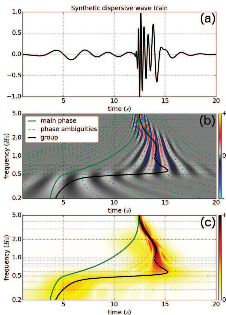
Figure III.3 : Méthode de détermination des lois de dispersion par analyse temps-fréquence (a) : Train d'onde dispersif synthétique obtenu selon la loi de dispersion du mode fondamentale de l'onde de Rayleigh calculée dans le modèle de vitesse moyen de Soultz-Sous-Forêts pour une distance source-récepteur de 10km. La forme d'onde est filtrée dans la gamme de fréquence 0.2 et 5Hz. (b) : mise en évidence du caractère dispersif de l'onde par la méthode des filtres gaussiens multiples : chaque ligne de la figure b correspond à la forme d'onde filtrée dans le voisinage d'une fréquence représentée en ordonnée. La courbe verte correspond à la date théorique d'arrivée de la phase principale du signal (elle s'obtient grâce à la loi de dispersion en vitesse de phase), les lignes vertes pointillées représentent les multiples ambiguïtés de phase associées à la phase
