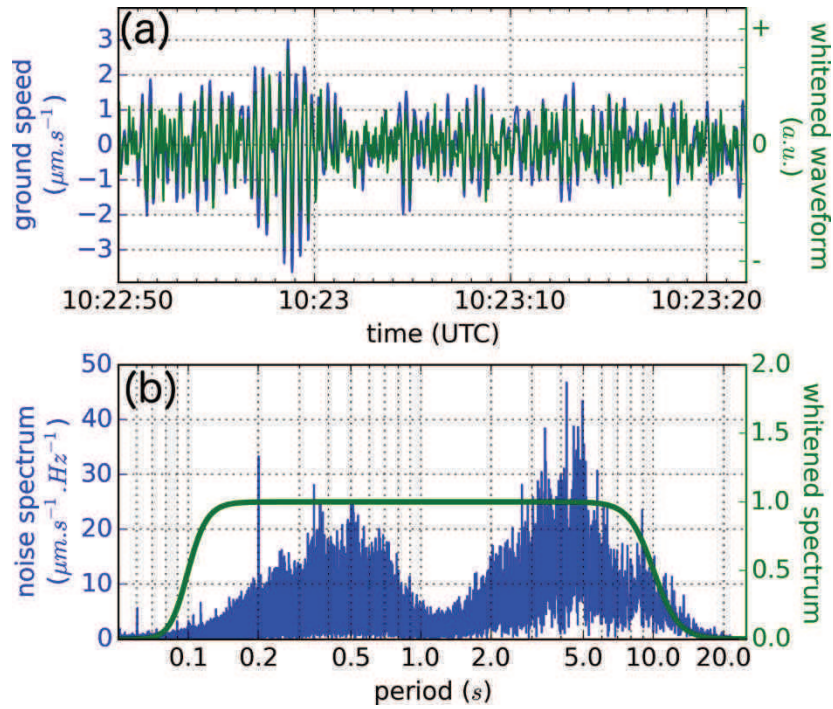
Figure II.4 : Méthode de normalisation fréquentielle (blanchiment spectral) utilisée dans cette thèse. (a) La trace bleue correspond à la vitesse du sol en \mu\text{m.s}^{-1} mesurée à la station RITT, composante verticale, le 14 janvier 2013 aux alentours de 10h23 (TU). La trace verte correspond à la forme d'onde après blanchiment spectral exprimée en unités arbitraires. (b) Spectre du bruit enregistré sur la même station entre 10h et 11h (TU) avant (spectre bleu) et après (spectre vert) l'opération de blanchiment spectral.
