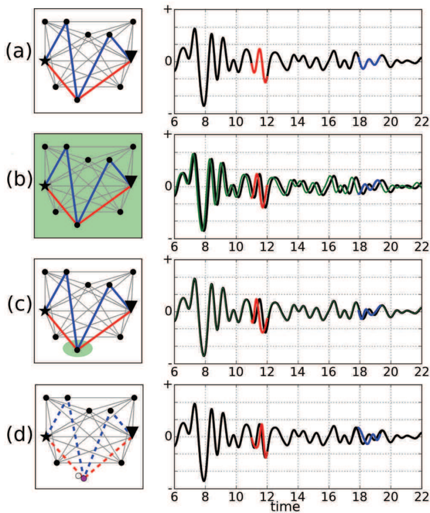
Figure IV.1 : Représentation schématique des perturbations de la coda causées par un changement du milieu. (a) Schéma représentant la diffraction multiple des ondes dans un milieu diffractant (points noirs). Les traits gris représentent les différents trajets des ondes depuis la source (étoile) vers le récepteur (triangle). Les traits rouge et bleu sont deux trajets possibles des ondes affectant des parties distinctes du signal. (b) Compression temporelle de la coda causée par une diminution homogène de la vitesse, symbolisée par la zone verte. Le décalage temporel est plus important pour le trajet bleu que pour le trajet rouge. (c) Décohérence de la coda causée par une variation locale de la vitesse, la perturbation n'est vue que par certains trajets et n'affecte que certaines parties du signal. (d) Perte de cohérence de la coda causée par un petit déplacement des points diffractants, le point mauve représente la nouvelle position d'un des points diffractants et les traits pointillés correspondent aux nouveaux trajets des ondes.
