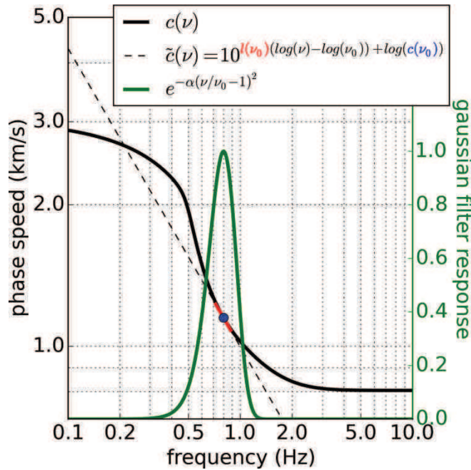
Figure III.12 : Paramétrisation de la courbe de dispersion au voisinage de la fréquence \nu_o . La loi de dispersion (courbe noire) est approchée par une loi linéaire du domaine \log c = f(\log \nu) (courbe pointillée). La courbe verte correspond au filtre passe-bande gaussien défini suivant Bensen et al. (2007) centré sur \nu_o = 0.8 \text{ Hz} et de paramètre \alpha = 15 .
