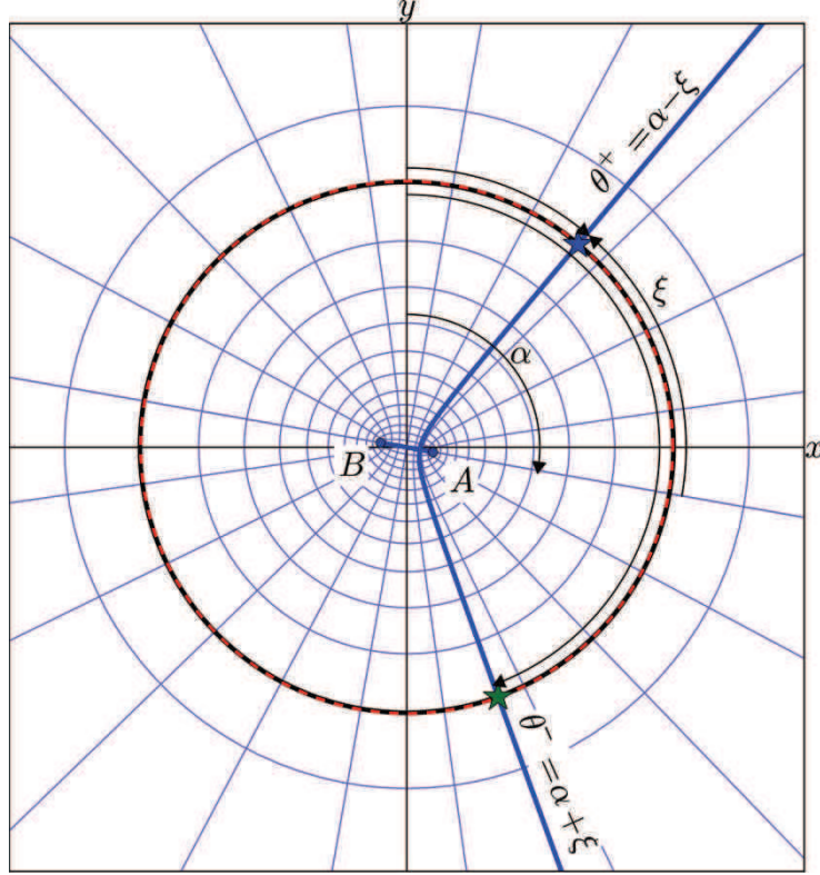
Figure III.14 : Paramétrisation du modèle de bruit. Des sources de bruit effectives (étoiles bleue et verte) sont positionnées sur une ellipse (représentée en trait noir plein) de paramètre \mu_o . Si \mu_o est suffisamment grand, cette ellipse se confond avec un cercle de rayon R \approx a \cosh \mu_o (trait rouge pointillé). Les sources sont repérées par rapport au nord grâce à leur back-azimuth noté \theta variant de 0 à 2\pi . Dans le référentiel d'une paire de station (points A et B), les sources sont repérées par le paramètre hyperbolique \xi variant de 0 à \pi . L'angle \alpha correspond à l'orientation de la paire AB par rapport au nord.
