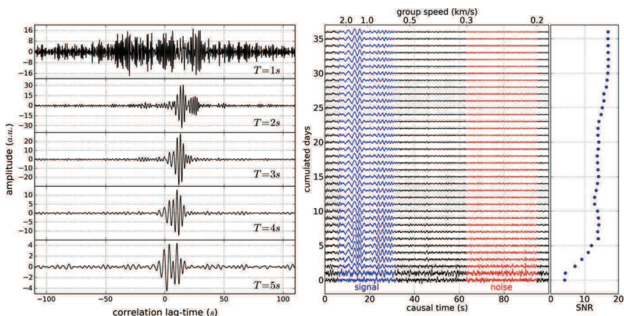
Figure V.4 : ( gauche ) émergence de la fonction de Green dans la fonction de corrélation de 1 à 5s de période pour la paire de capteurs 072-171 du réseau EstOf orientée dans l'axe dominant du bruit ambiant (296.76°) et séparée d'une distance de 18.94km. Les amplitudes sont exprimées en unités arbitraires. T désigne la période. ( droite ) Evolution de la partie causale du corrélogramme entre 1s et 5s de période en fonction du nombre de jours de bruit utilisés (axe vertical). La partie bleue de la trace (comprise entre les vitesses de groupe 0.6km/s et 3.3km/s) correspond à la fenêtre de signal, la partie rouge (0.2 à 0.3km/s) correspond à la fenêtre de bruit. Le rapport signal-sur-bruit est défini par le maximum de l'enveloppe sur la fenêtre de signal divisé par la moyenne quadratique de la fonction de corrélation dans la fenêtre de bruit (Bensen et al., 2007). Son évolution est représentée sur la partie la plus à droite de la figure (points bleus).
