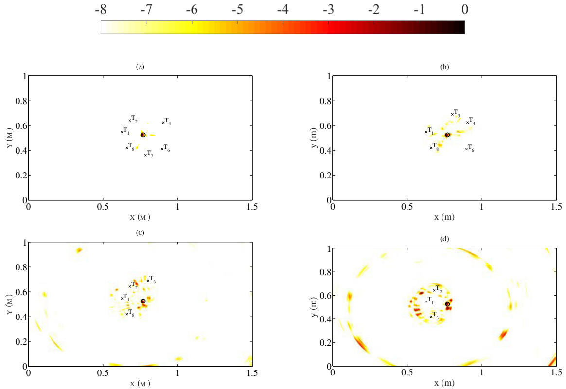
Figure 3.16 – Images de localisation par corrélation de bruits acoustiques (en décibel) : a) 6 capteurs, b) 5 capteurs, c) 4 capteurs et d) 3 capteurs, respectivement. Le défaut est placé à (1,12 , 0,57) m.
