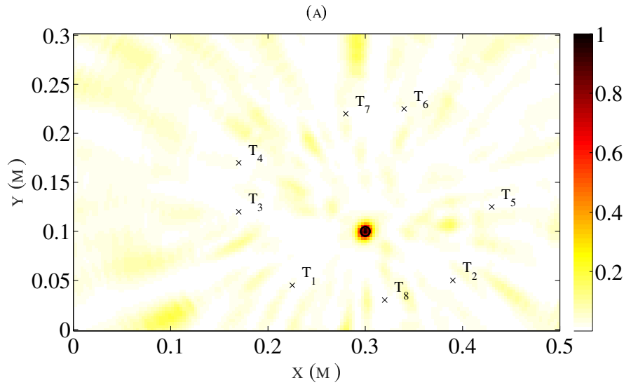
Figure 3.4 – Résultat de localisation passive de défaut obtenu à partir de \Delta \mathbf{s}(t) . Le maximum d'intensité correspond à la position du défaut (0,3 , 0,1) m.
