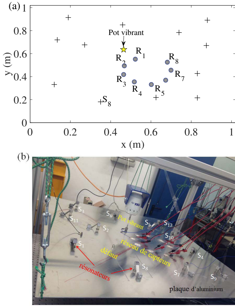
Figure 4.2 – (a) Schéma du dispositif expérimental : le pot vibrant génère le champ BF primaire. 12 systèmes masse-ressort S_1...S_{12} (+) sont collés à la plaque. Chaque résonateur secondaire ramène le champ primaire BF en un champ secondaire HF (interactions poutre-surface de contact), et le réinjecte à la plaque. (b) Photographie du banc de test utilisé.
