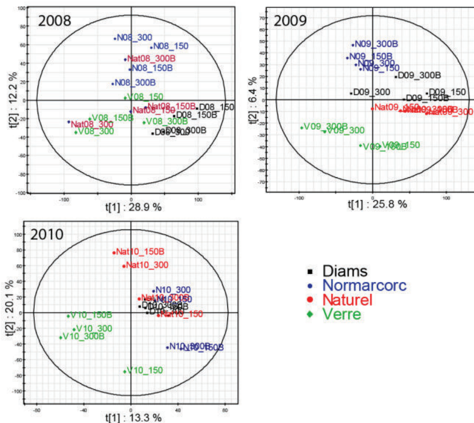
Figure 37: PLS-DA pour chaque millésime, 2008, 2009 et 2010 des masses issues de l'analyse FTICR-MS en fonction du type d'obturateur (diams® en noir, nomacorc en bleu, naturel en rouge et ampoule en verre en vert).
