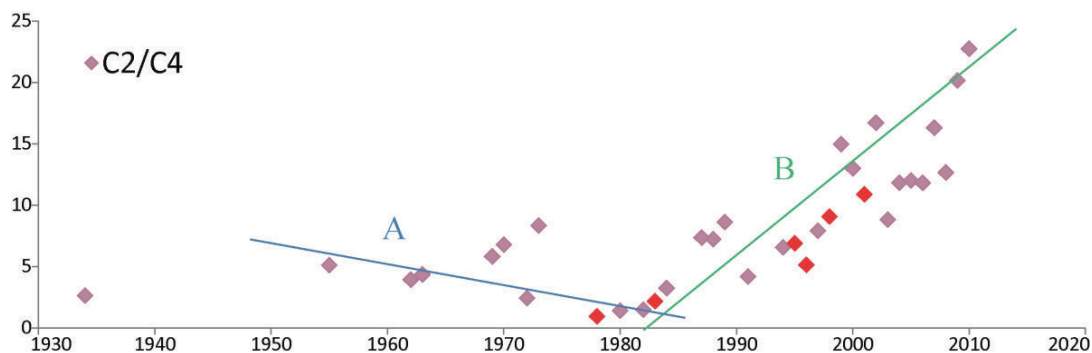
Figure 46: Évolution du rapport des composantes C2 sur C4 en fonction des millésimes pour la série verticale de Corton Charlemagne. L'évolution du rapport C2/C4 présente deux tendances avec une rupture de pente au niveau des années 1980-1990. Code couleur : rose rapport des composantes C2/C4, rouge vins détectés comme oxydés lors de la dégustation, courbe bleu première tendance du rapport C2/C4 et courbe verte deuxième tendance du rapport C2/C4.
