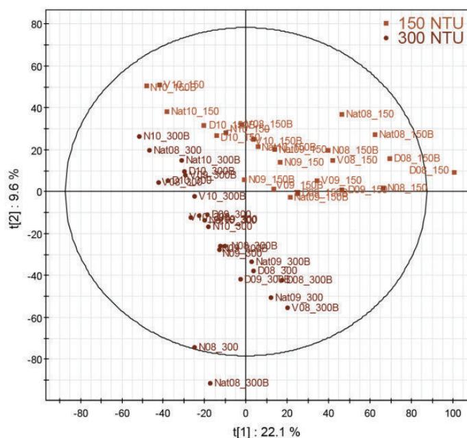
Figure 38: PLS-DA des échantillons de vins en fonction de l'intensité du débourage, 150 NTU (en marron clair) et 300 NTU (en marron foncé) indépendamment du millésime, du bouchage et de la présence de bentonite en vinification.
