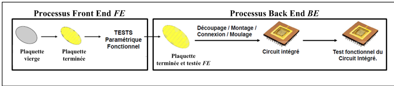
Figure 1.5 : Représentation du processus global de transformation d'une plaquette de silicium en un circuit intégré
