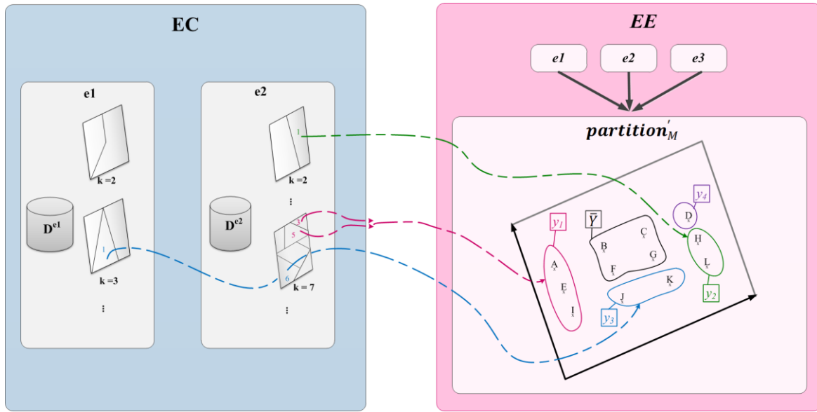
Figure 4.10: Exemple des deux types de règles à identifier. La flèche verte représente une règle simple et la bleue une règle de trajectoire. Les groupes y_1 , y_2 , y_3 et y_4 sont les sous-phénomènes à expliquer; \bar{Y} contient les autres produits.
