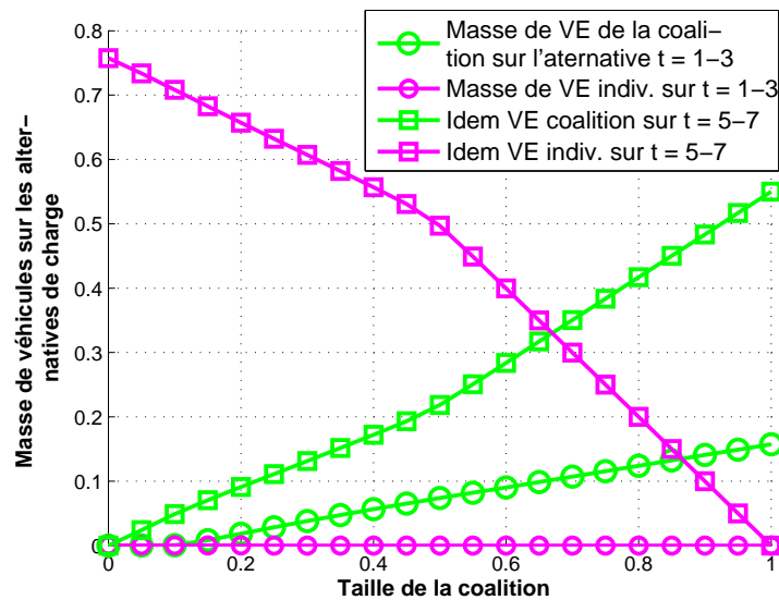
FIGURE 6.7 – Configuration d’équilibre composite en fonction de la taille de la coalition \Omega dans le cadre d’une charge nocturne ( T = 7, C = 3 ) et avec une métrique physique linéaire f^{\text{RD}}(\ell_t) = \ell_t . Les propriétés de monotonie établies dans le cas réduit T = 3, C = 2 semblent toujours valides. N.B : VE est utilisé pour "véhicule électrique".
