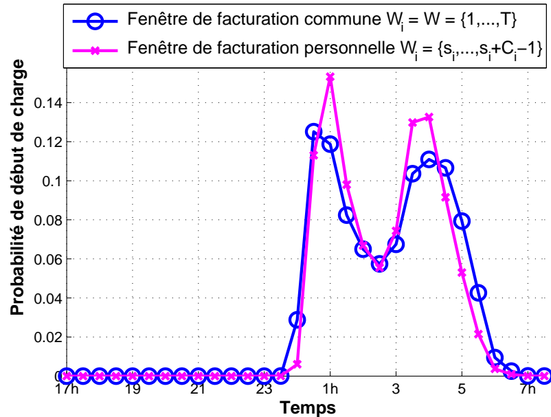
FIGURE F.5 – Distribution des instants de début de charge n obtenus avec l'Algorithme 3.1 dans le cas de la mobilité statistique : impact du choix de la fenêtre de facturation W_i . Les distributions sont très proches.
