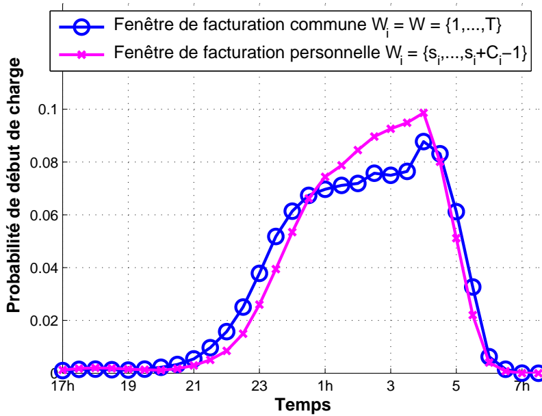
FIGURE F.6 – Distribution des instants de début de charge n obtenus avec l’Algorithme 3.1 dans le cas bruité : impact du choix de la fenêtrée de facturation \mathcal{W}_i . Les distributions sont relativement proches.
