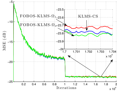
(a) MSE
