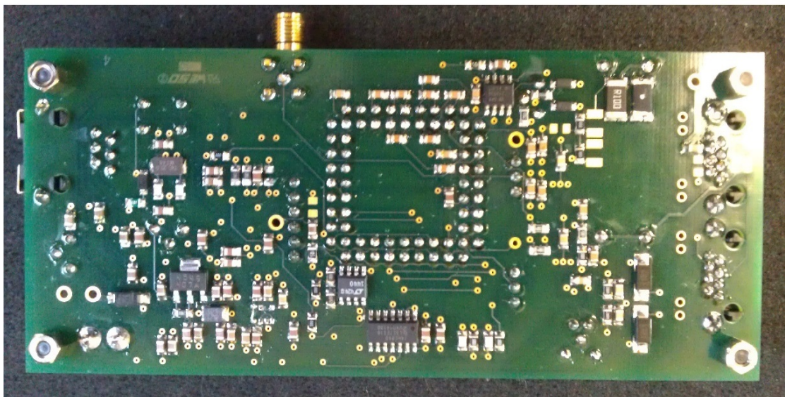
FIGURE 5.34: Démonstrateur final du système de calibrage, intégrant le prototype ARCaD 4 et la génération du courant de référence. Cette carte ne nécessite qu'une source d'alimentation de 12V pour fonctionner. Dimensions = 70mm × 170mm.
