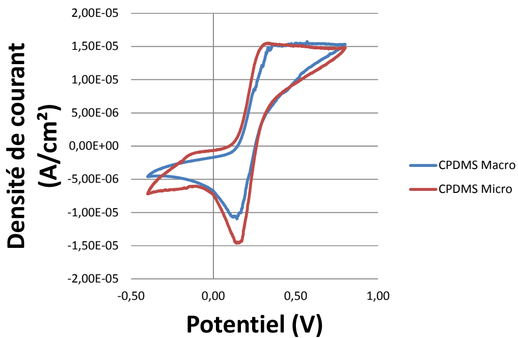
Figure 110 : Voltammétrie cyclique d'électrodes de CPDMS macroscopique (rouge) et microscopique (bleu) dans une solution de 1 mM de ferrocène dans du KCl 0,1 M
