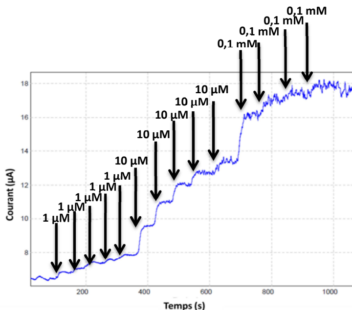
Figure 62 : Chronoampérométrie d'une électrode de diamant fonctionnalisée par de l'acétylcholinestérase sur chitosane dans une solution de PBS 10X avec ajouts d'acétylcholine. L'augmentation de concentration est indiquée.
