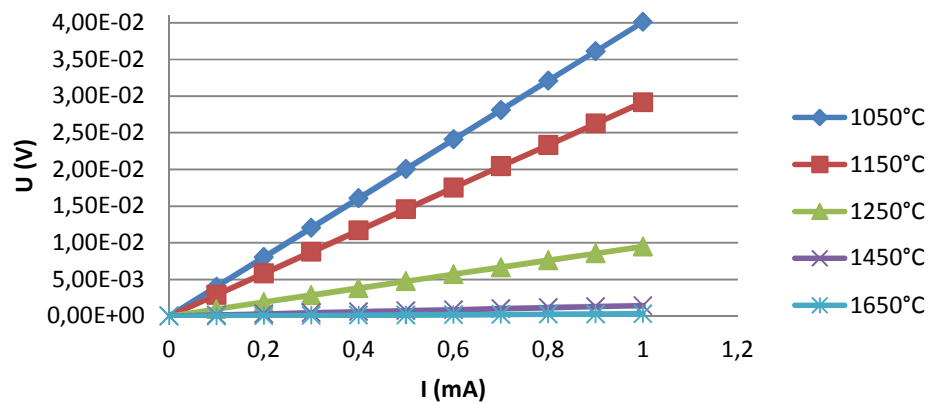
Figure 42 : Caractérisation 4 points d'échantillons de PPF sur SiC recuit à différentes températures
