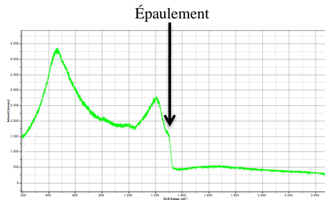
Figure 37 : Spectre Raman d'un échantillon de diamant dopé bore sur SiC
