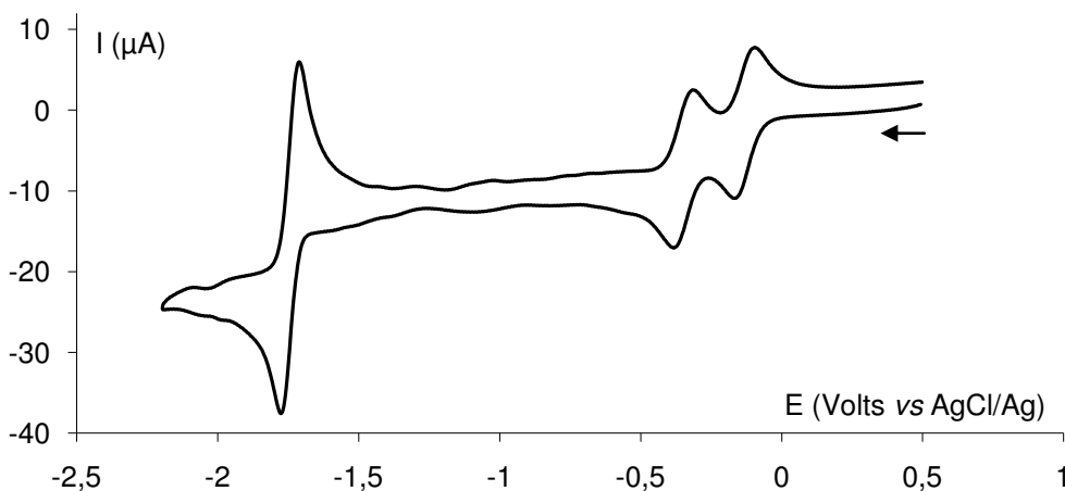
Figure II-13 : Voltampérogramme de 22^{2+} , dans l'acétonitrile en présence de \text{NBu}_4\text{PF}_6 (0,1 M) (Vitesse de balayage 0,1 \text{ V}\cdot\text{s}^{-1} , électrode de travail en carbone vitreux).
