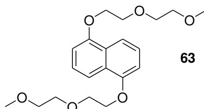
Figure III-10 : Dérivé de 1,5-dihydroxynaphtalène utilisé comme template dans la synthèse de la « Blue-Box »
