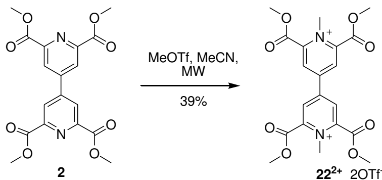
Figure II-12 : Schéma de synthèse du viologène 22^{2+}2\text{OTf}^-
