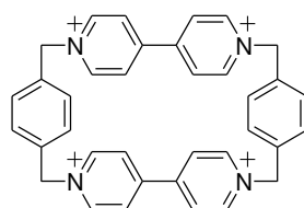
Figure I-18 : Représentation schématique de la « Blue-Box ». 53
