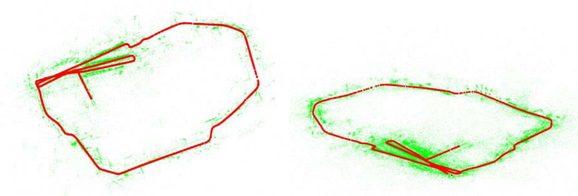
(c) Reconstruction de l'algorithme de SLAM avec 2056 images clés et 47K points 3D.
