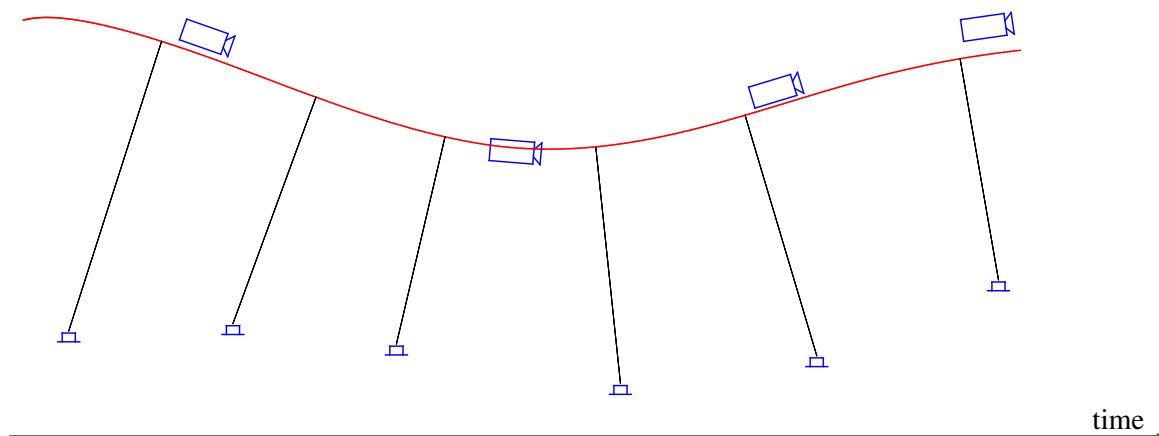
(b) Interpolation et dérivation des poses caméra.
