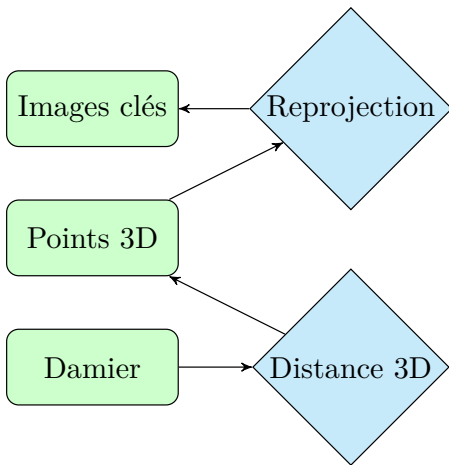
(a) Graphe du MCSLAM
