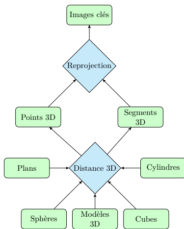
(b) Graphe
