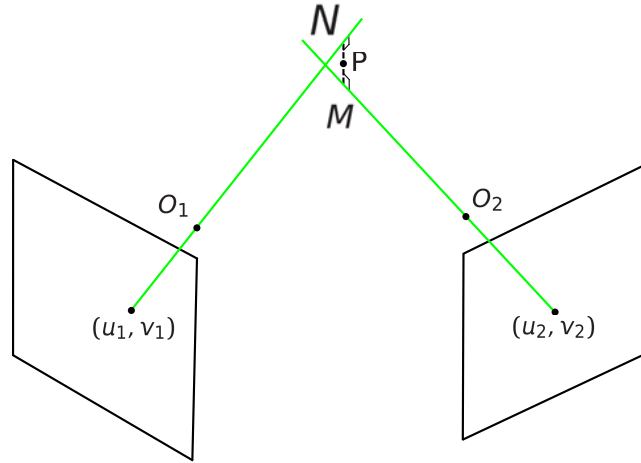
FIGURE 1.10 – Illustration de la méthode de triangulation du point milieu. Le point triangulé est choisi comme le milieu du segment minimal et orthogonal aux deux droites rétro-projetées.
