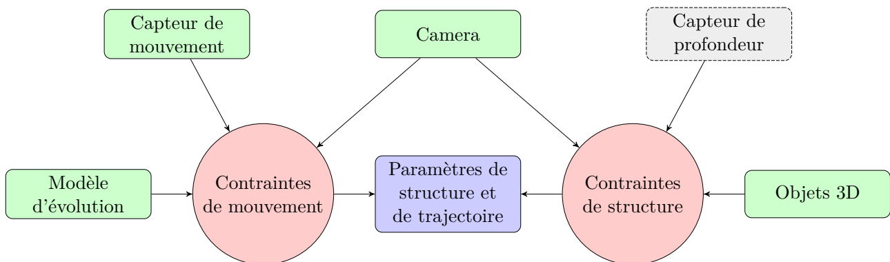
FIGURE 8.1 – L'algorithme M-CSLAM est conçu pour être facilement configurable. Il peut gérer des configurations faisant intervenir différentes contraintes. Par exemple, un capteur de profondeur pourrait être intégré dans le système.
