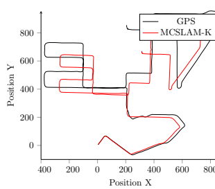
(h) Trajectoire
