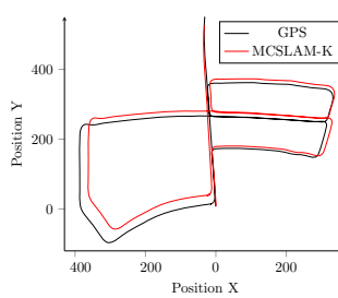
(d) Trajectoire
