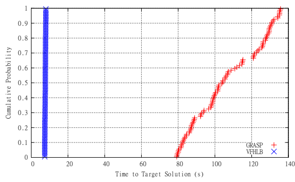
(c) TTTPlot: 20-0.8-30-3
