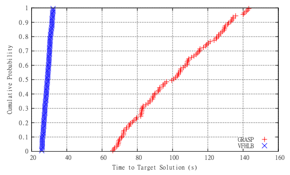
(d) TTTPlot: 20-0.8-30-4
