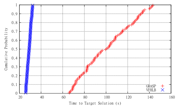
(d) TTTPlot: 20-0.8-30-4
