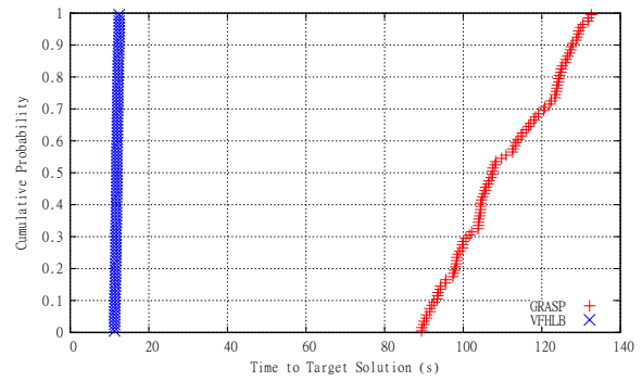
(b) TTTPlot: 20-0.8-30-2
