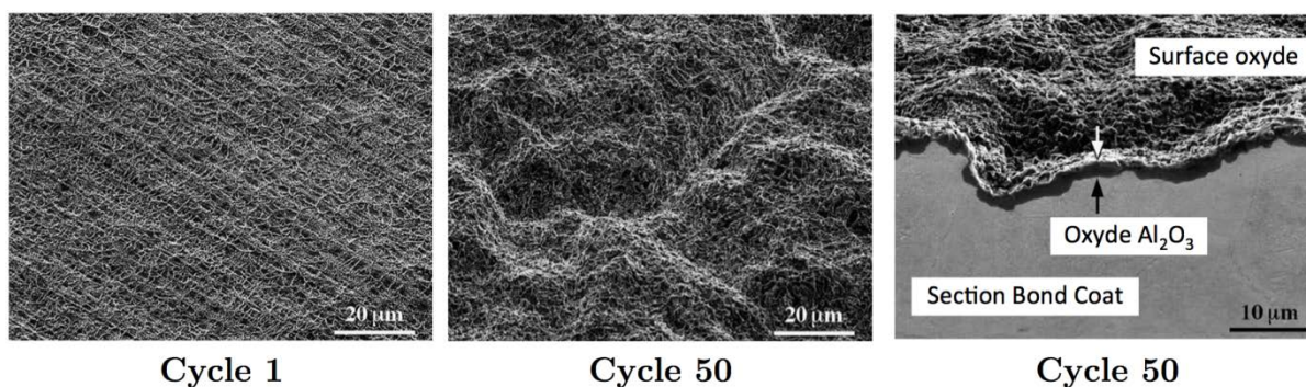
Figure 1.8: Illustration du phénomène de rumpling d'une couche de liaison type (\text{Ni}, \text{Pt})\text{Al} entre le 1 er et le 50 ème cycle d'une heure à 1200^\circ\text{C} [65].
