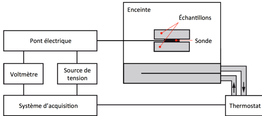
Figure 2.10: Schéma de l'analyseur thermique Hot Disk utilisé pour la mesure de conductivité thermique et de diffusivité thermique de pastilles frittées de zircon YSZ:Ln 3+ .
