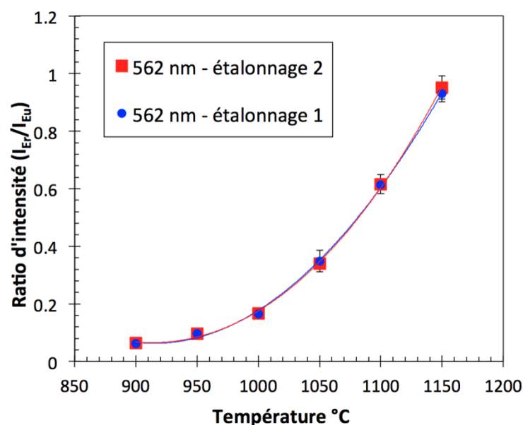
Figure 5.22 : Évolution du ratio d'intensité de fluorescence R_I en fonction de la température pour deux montages expérimentaux de mesure différant par le volume de poudre sondée (nombre de centres fluorescents excités) et par la distance d'observation.
