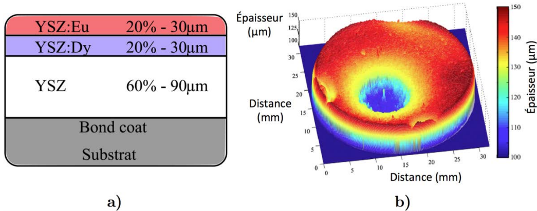
Figure 1.33 : (a) Structure d'une BT multicouche développée pour l'évaluation quantitative de l'érosion [144], (b) reconstruction 3D du profil d'érosion de l'échantillon à partir des images de fluorescence [29].
