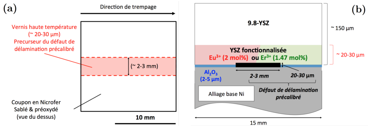
Figure 5.3: (a) Schéma en vue du dessus de la préparation du substrat Nicrofer avant le dépôt du revêtement fonctionnalisé illustrant la position et les dimensions de la couche de vernis pré-curseur du défaut de décohésion pré-calibré, (b) schéma de la section de la BT dimensionnée, contenant une zone de décohésion pré-calibrée et une couche fonctionnalisée YSZ:Eu 3+ ou YSZ:Er 3+ de 20-30 μm au niveau de l'interface céramique/métal.
