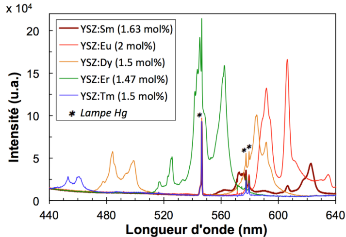
Figure 4.3 : Comparaison des spectres de fluorescence sous excitation UV (lampe à vapeur de mercure) des poudres d'aérogel optimisées YSZ: Ln^{3+} ( Ln=Sm, Eu, Dy, Er, Tm ) utilisées pour le dépôt de BT par trempage-retrait (cf. Chapitre 3 section 3.4).
