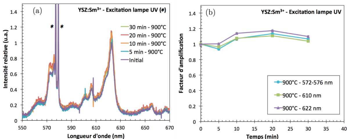
Figure A.IV.1: Évolution (a) des spectres de fluorescence et (b) de l'intensité intégrée des principaux pics de fluorescence de poudres d'aérogel de zircone YSZ:Sm 3+ (1.6 mol%) avec la durée de traitement thermique en conditions isothermes à 900°C. Les spectres et les intensités intégrées sont normalisés par rapport à l'état initial (poudre d'aérogel calcinée à 700°C).
