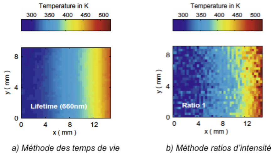
Figure 1.23: Comparaison du champ de températures d'un gradient thermique unidirectionnel mesuré sur un luminophore Mg_4FGeO_6:Mn (a) avec la méthode des temps de vie et (b) avec la méthode des ratios d'intensité.
