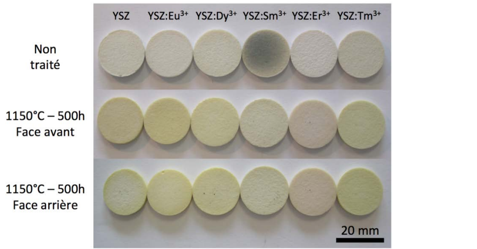
Figure 3.17: Photographies des pastilles frittées de YSZ:Ln 3+ avant et après le traitement thermique de vieillissement de 2 x 250h à 1150°C.
