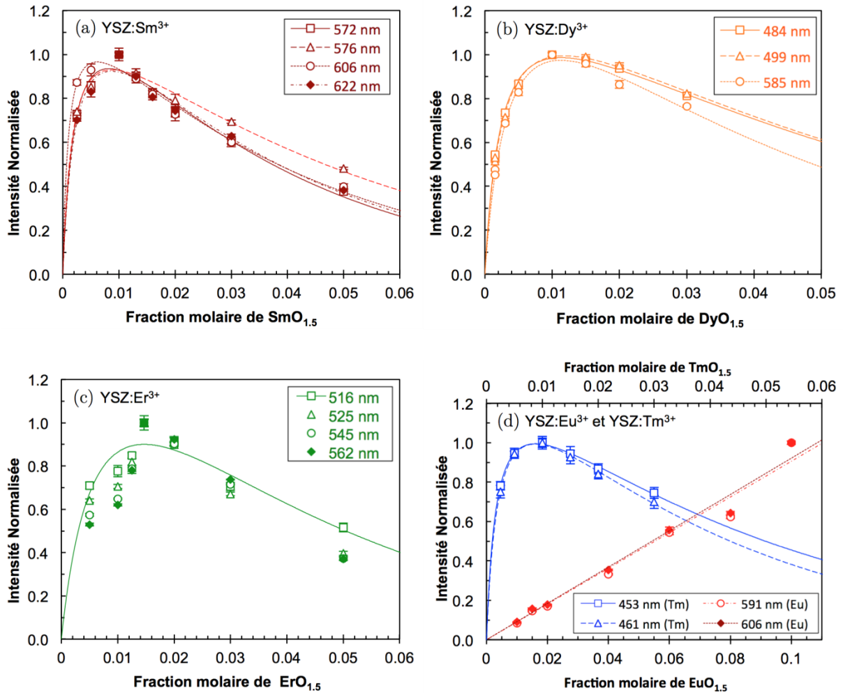
Figure 3.7: Évolution de l'intensité intégrée des pics de fluorescence des poudres de xérogel YSZ:Ln^{3+} avec la concentration en activateur Ln_{0.5} : (a) YSZ:Sm^{3+} , (b) YSZ:Dy^{3+} , (c) YSZ:Er^{3+} , (d) YSZ:Eu^{3+} et YSZ:Tm^{3+} . Les courbes sur chaque graphique ( YSZ:Eu^{3+} excepté) correspondent aux résultats de la régression des données expérimentales avec le modèle de self-quenching de Johnson-Williams [185,186], cf. équation 3.1.
