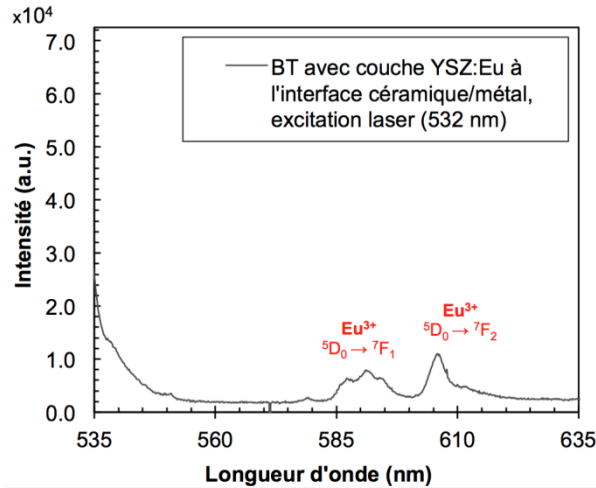
Figure 4.15: Spectre de fluorescence d'une BT de 200 µm d'épaisseur contenant une couche YSZ:Eu 3+ estimée à 15-25 µm d'épaisseur au niveau de l'interface céramique/métal. L'échelle et les conditions de mesure sont les mêmes que pour la Figure 4.14 (b).
