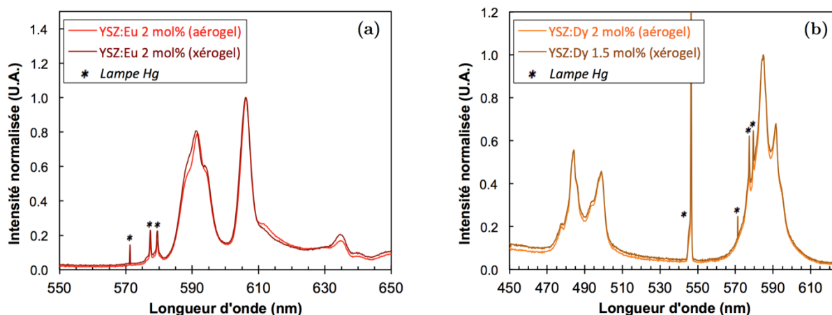
Figure 3.6: Comparaison des spectres de fluorescence normalisés de poudres d'aérogel et de xérogel (a) YSZ:Eu^{3+} 2 mol%, (b) YSZ:Dy^{3+} 1.5 mol%.
