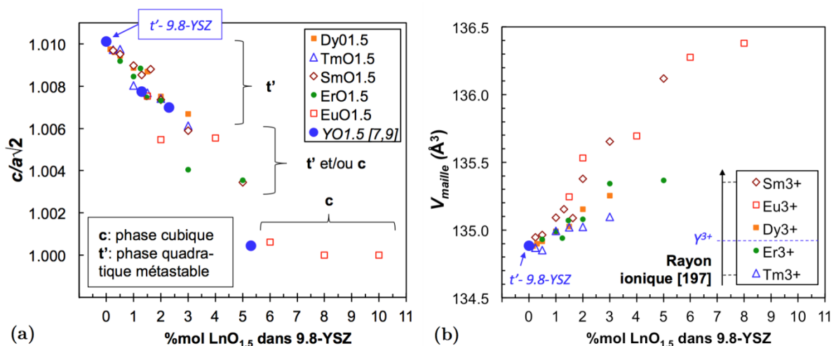
Figure 3.12: Évolution (a) du paramètre de tétragonalité c/a\sqrt{2} et (b) du volume de la maille cristalline en fonction de la concentration molaire en LnO_{1.5} ( Ln=Sm, Eu, Dy, Er, Tm ) dans la zircon ZrO_2 contenant déjà 9.75 mol% de YO_{1.5} .
