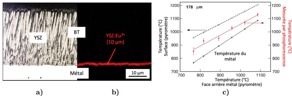
Figure 1.29: Micrographie optique de la section d'une BT contenant une couche de 10 µm de YSZ:Eu 3+ à l'interface TGO/YSZ [21] (a) sous lumière blanche, (b) sous UV ; (c) températures en surface, sur la face arrière et à l'interface TGO/YSZ de cette même BT capteur [21].
