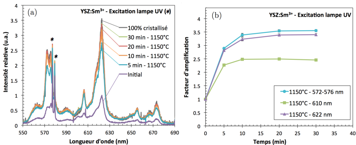
Figure A.IV.2: Évolution (a) des spectres de fluorescence et (b) de l'intensité intégrée des principaux pics de fluorescence de poudres d'aérogel de zircone YSZ:Sm 3+ (1.6 mol%) avec la durée de traitement thermique en conditions isothermes à 1150°C. Les spectres et les intensités intégrées sont normalisés par rapport à l'état initial (poudre d'aérogel calcinée à 700°C).
