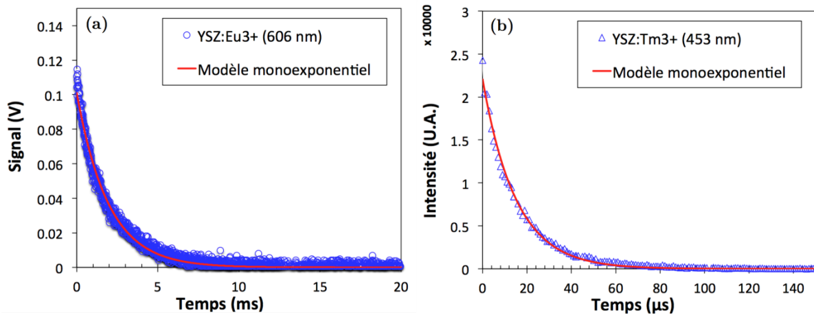
Figure 2.17: (a) Extinction du signal de fluorescence de la transition {}^5D_0 \rightarrow {}^7F_2 (606 nm) des ions \text{Eu}^{3+} mesurée sur une pastille frittée de \text{YSZ}:\text{Eu}^{3+} avec le banc de fluorescence, (b) extinction du signal de fluorescence de la transition {}^1D_2 \rightarrow {}^3F_{4L2} ou {}^1D_2 \rightarrow {}^3F_{4L1} (460 nm) des ions \text{Tm}^{3+} mesurée sur une pastille frittée de \text{YSZ}:\text{Tm}^{3+} avec le lecteur spectral multimodes Varioskan Flash. Les courbes en rouge correspondent à la régression des données expérimentales avec le modèle exponentiel ( n=1 ) présenté par l'équation 2.7.
