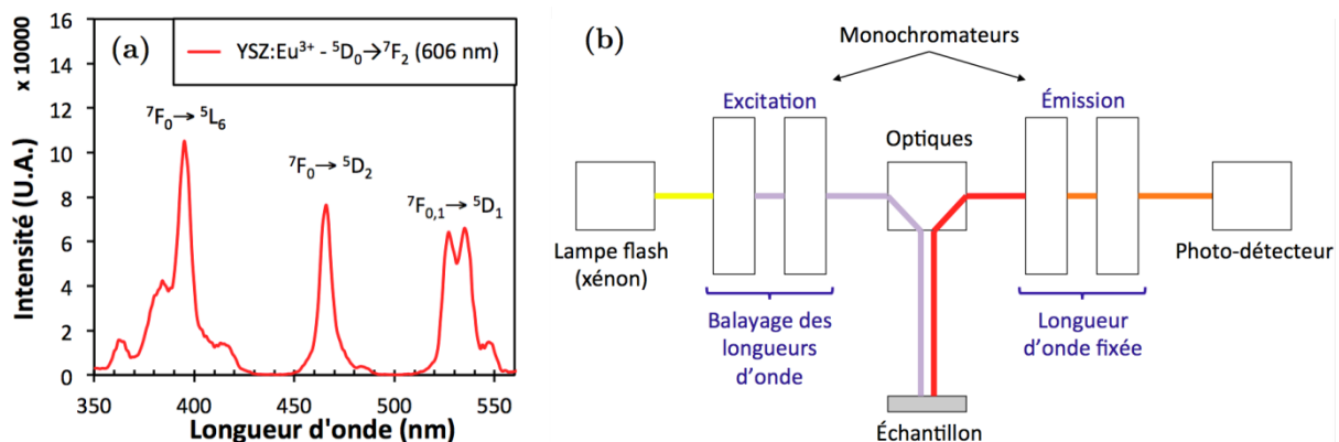
Figure 2.15: (a) Spectre d'excitation de la transition {}^5D_0 \rightarrow {}^7F_2 (émission à 606 nm) de la zircone YSZ:Eu 3+ , (b) principe de la mesure d'un spectre d'excitation avec le lecteur à balayage spectral multi-modes Varioskan Flash (Thermo Scientific).
