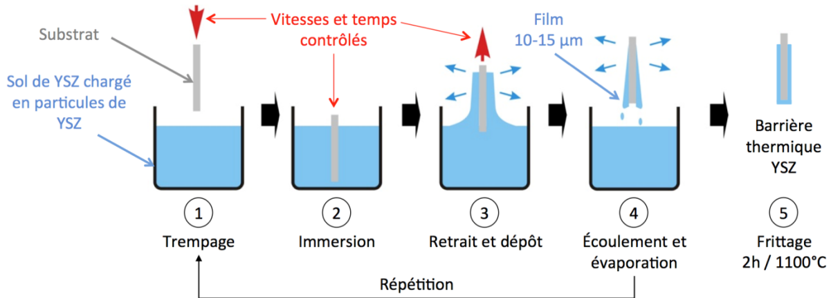
Figure 1.6: Illustration des étapes du procédé de trempage-retrait ( dip-coating ) pour le dépôt de BT en zircone YSZ [8].
