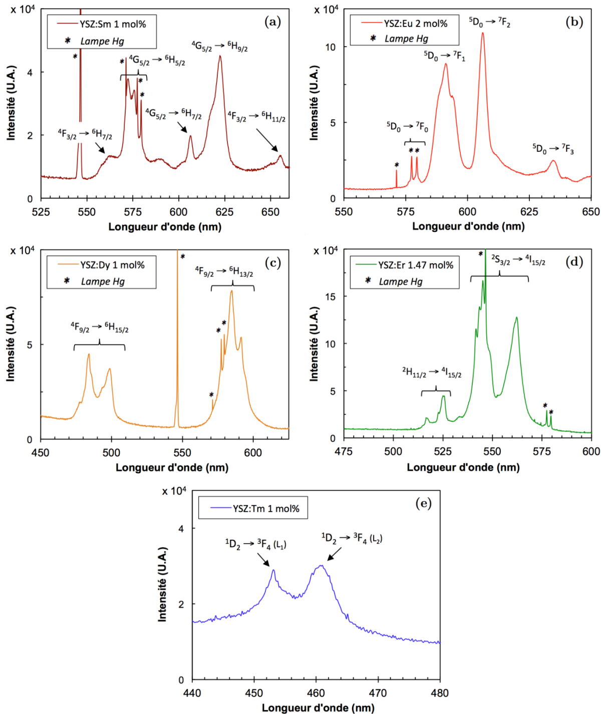
Figure 3.2: Spectres de fluorescence des différents luminophores \text{YSZ:Ln}^{3+} sous forme de poudres de xérogel de composition (\text{YO}_{1.5})_{0.098}(\text{ZrO}_2)_{0.902-x}(\text{LnO}_{1.5})_x traitées à 1100°C:
