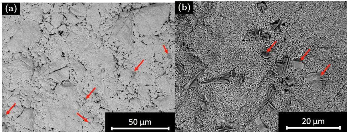
Figure 3.18: Micrographies MEB en mode électrons rétrodiffusés de la surface des pastilles YSZ et YSZ:Ln 3+ après le traitement thermique de vieillissement de 2 \times 250\text{h} à 1150^\circ\text{C} (a) 9.8-YSZ, (b) 8.2-YSZ :Sm 3+ .
