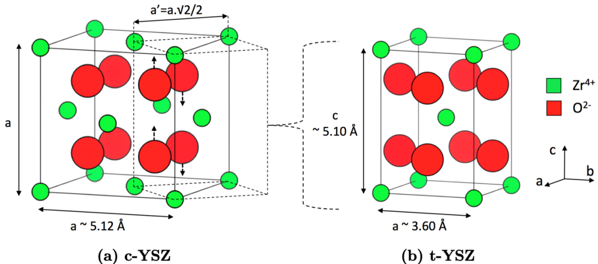
Figure 2.9 : Représentations schématiques des mailles cristallines primitives de la zircon (a) cubique c (groupe d'espace Fm\bar{3}m ) et (b) quadratique t' (groupe d'espace P4_2/nmc ) illustrant le lien entre les deux mailles.
