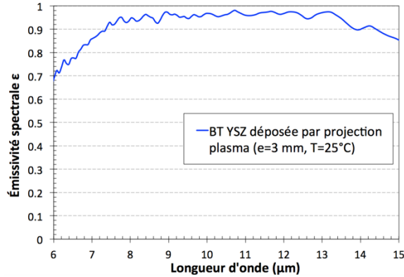
Figure 5.6 : Émissivité spectrale à température ambiante dans le domaine 7\text{-}14 \text{ }\mu\text{m} d'une BT YSZ de 3 \text{ mm} d'épaisseur déposée par projection plasma.
