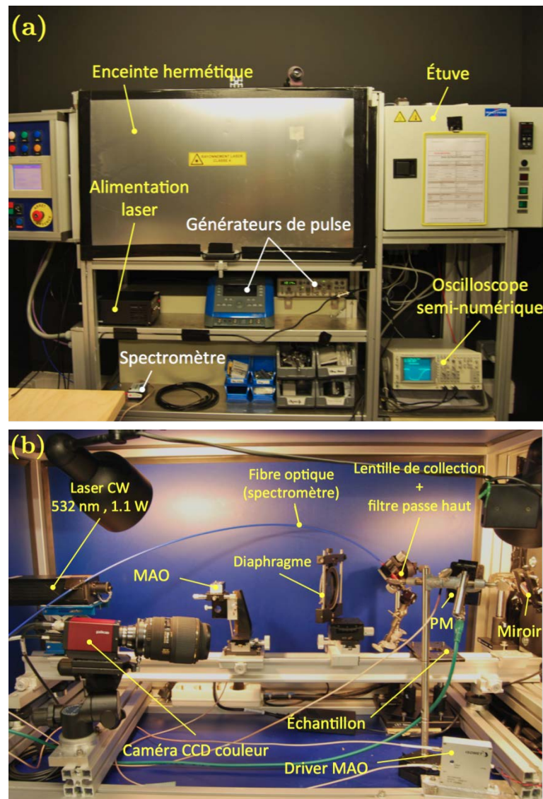
Figure 2.13: Photographies du banc de fluorescence dans la configuration pour la mesure de temps de vie de poudres de zircon YSZ:Eu^{3+} et YSZ:Er^{3+} (échantillons à l'horizontale).
