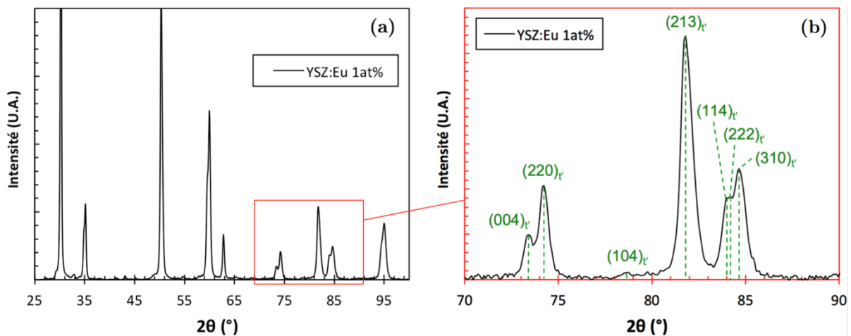
Figure 3.3: Spectre de diffraction des rayons X d'une poudre de xérogel 9.7YSZ dopée avec 1 mol% de EuO_{1.5} et traitée à 1100°C (a) dans tout le domaine angulaire, (b) limité au domaine 2\theta=70-90^\circ .
