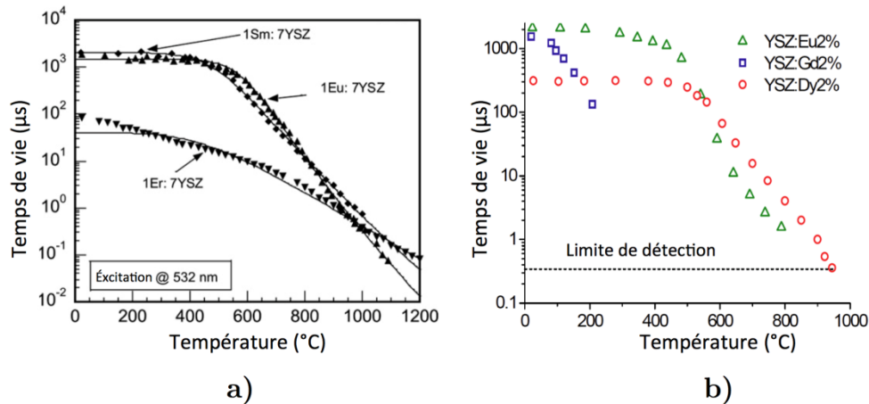
Figure 1.26: (a) Courbes d'étalonnage temps de vie/température (a) de poudres frittées de 1Eu:7YSZ, 1Sm:7YSZ et 1Er:7YSZ excitées à 532 nm [94], (b) de revêtements EB-PVD 2Eu:YSZ, 2Gd:YSZ et 2Dy:YSZ [22].
