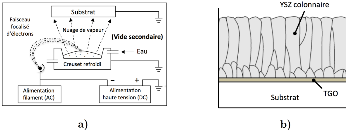
Figure 1.5: (a) Représentation schématique du principe de l'évaporation sous vide sous faisceau d'électrons (EB-PVD) [58], (b) vue en coupe schématique de la structure d'une BT déposée par EB-PVD [33].
