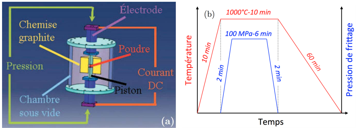
Figure 2.5 : (a) Principe du procédé de frittage flash [166], (b) cycle de frittage flash appliqué pour la fabrication de pastilles de YSZ:Ln 3+ à partir de poudres d'aérogel.
