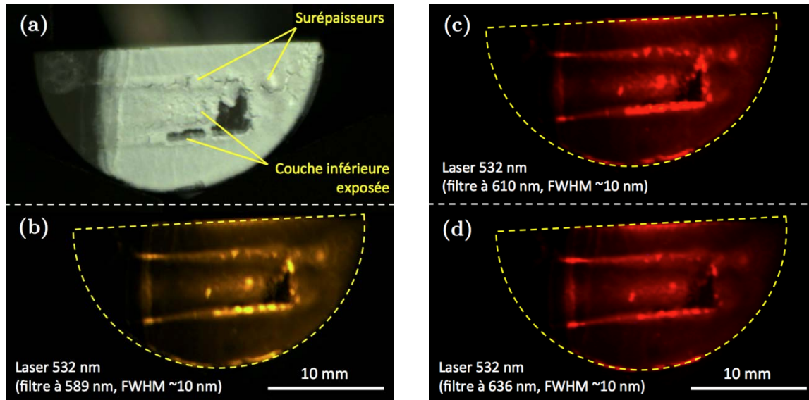
Figure 5.12: Photographies d'une BT sol-gel ( \sim 200 \mu\text{m} d'épaisseur) déposée sur un substrat base nickel (AM1) contenant une couche de zircone YSZ:Eu 3+ et un défaut pré-calibré au niveau de l'interface céramique/métal (a) sous lumière blanche ; sous l'illumination du faisceau étendu à 532 nm d'un laser Nd:YAG et avec un filtre interférentiel (FWHM \sim 10 nm) centré sur les pics principaux d'émission des ions Eu 3+ à (b) 589 nm, (c) 606 nm et (d) 635 nm.
