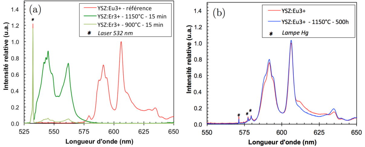
Figure 5.21: Comparaison des spectres de fluorescence (a) des poudres d'aérogel de zircone YSZ:Er 3+ traitées 15 min à 900°C et à 1150°C avec celui de la poudre d'aérogel de zircone YSZ:Eu 3+ (2 mol%) supposée complètement cristallisée, (b) de pastilles de zircone YSZ:Eu 3+ avant et après un traitement thermique de 500h à 1150°C (face arrière non exposée à l'atmosphère du four) illustrant la stabilité thermique de l'intensité émise par ce luminophore à l'état complètement cristallisé.
