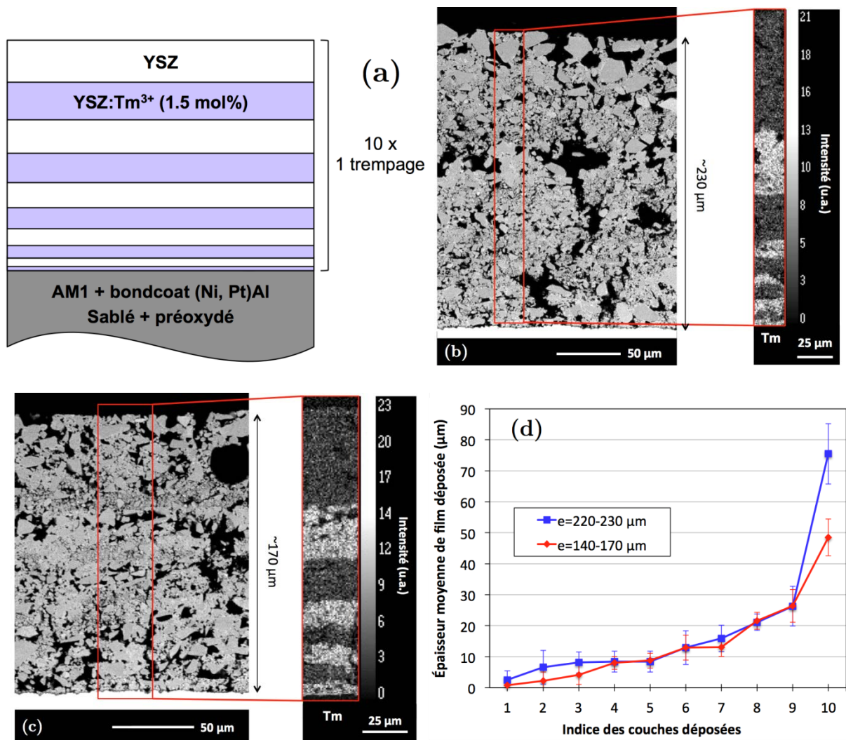
Figure 4.12: (a) Schéma de la section de la BT multicouches YSZ/YSZ:Tm 3+ utilisée pour caractériser les épaisseurs déposées à chaque trempage durant une campagne de trempage-retrait ; micrographies MEB et cartographies de composition par microsonde de l'élément Tm issues des zones (b) de forte et (c) de faible épaisseur de cette BT ; (d) évolution de l'épaisseur moyenne de film déposée à chaque trempage dans les zones de forte et de faible épaisseur.
