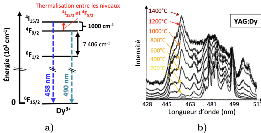
Figure 1.17: Illustration du phénomène de thermalisation : (a) extraits du diagramme de Dieke des ions trivalents dysprosium [17], (b) évolution du spectre de fluorescence de YAG:Dy 3+ avec la température [104].
