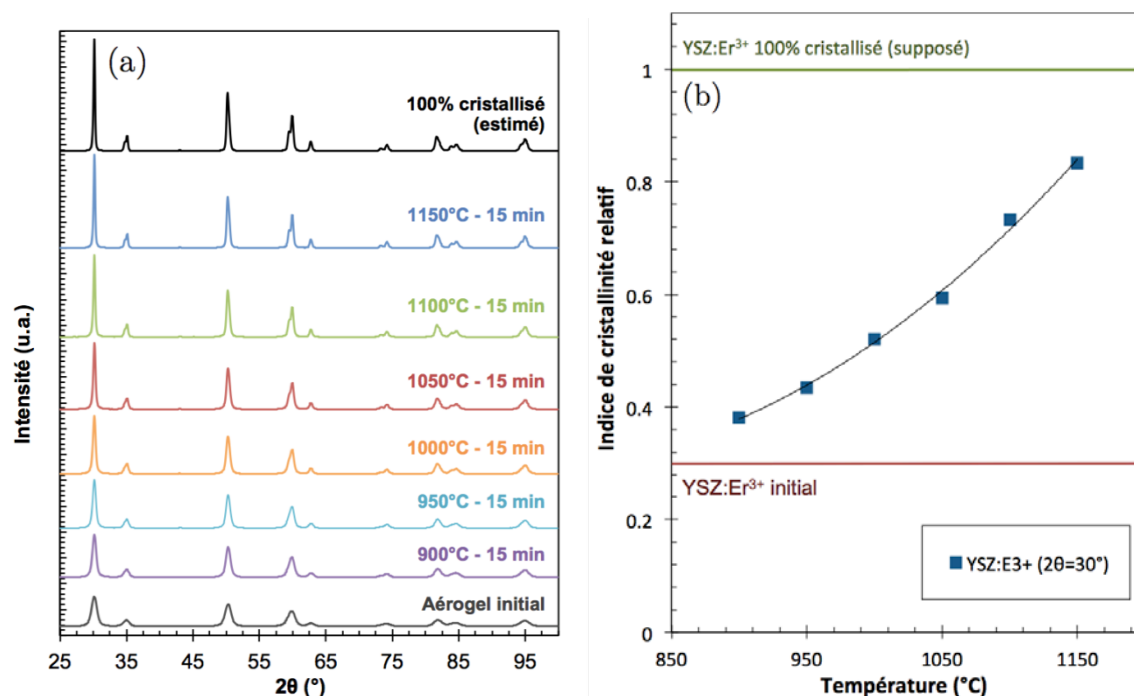
Figure 5.18: (a) Évolution des diagrammes de DRX et (b) de l'indice relatif de cristallinité de poudres de zircon YSZ:Er^{3+} (défini par rapport à l'intensité maximale du pic de diffraction à 30^\circ de la poudre supposée complètement cristallisée) pour différentes températures de traitement thermique entre 900^\circ C et 1150^\circ C .
