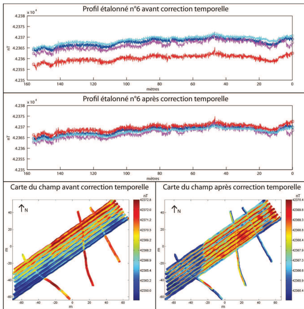
Figure 4.11 – Illustration des effets de la correction temporelle sur la cartographie C10 et son profil d'acquisition 6. L'échelle des cartes est en équi-population. Pour les profils, chaque couleur correspond à un des quatre magnétomètres.
