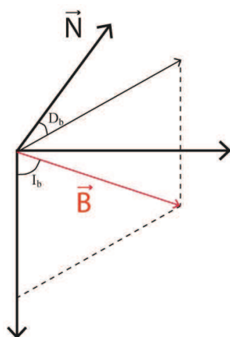
Figure 2.3 – Représentation de la déclinaison D_b et de l'inclinaison I_b du champ magnétique terrestre \vec{B} en rouge. L'intensité correspond à la norme de \vec{B} .
