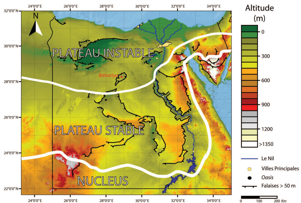
Figure 1.2 – Division structurelle de l'Égypte d'après Said (Meshref 1990) sur le fond topographique de la figure 1.1 (p. 20). Bahariya se trouve au niveau de la marge Sud du plateau instable.
