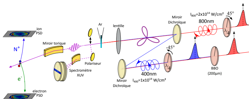
FIGURE 4.44 – Dispositif expérimental utilisé pour la mesure de l'état de polarisation des harmoniques générées par combinaison de champs à deux couleurs ( 800\text{nm} + 400\text{nm} ). Le bras 800\text{nm} n'est composé que d'une lame quart d'onde permettant de passer de linéaire à circulaire gauche/droite. Le bras 400\text{nm} est composé d'un cristal doubleur de BBO ( 200\mu\text{m} d'épaisseur) et d'une lame quart d'onde optimisée à 400\text{nm} . Un premier miroir dichroïque placé sur le bras du 400\text{nm} permet de filtrer le champ à 800\text{nm} non converti après passage dans le BBO. Un deuxième miroir dichroïque permet de recombinaison des deux faisceaux. Le délai entre les deux champs est fixe et de tel sorte à ce que les deux enveloppes soient superposées. Le système de caractérisation est le même que pour les dispositifs N_2/SF_6 . La PO n'a pas pu être faite avec ce dispositif, les miroirs d'insertion et le spectromètre XUV permettent uniquement l'observation du spectre harmonique.
