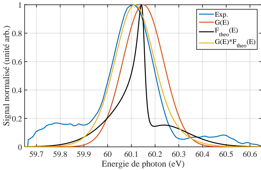
FIGURE 5.18 – Détermination de la fonction d’appareil/résolution du spectromètre à temps de vol dans la région 10\text{eV} . Voir texte pour plus de détails.
