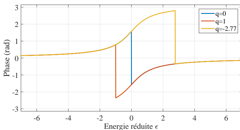
FIGURE 5.10 – Évolution de la phase du facteur résonant du dipole de transition \langle \psi_E | \mathcal{O} | g \rangle en fonction de l'énergie réduite \epsilon , pour différentes valeurs de q_{\tilde{a}g} = 0; 1; -2.77 .
