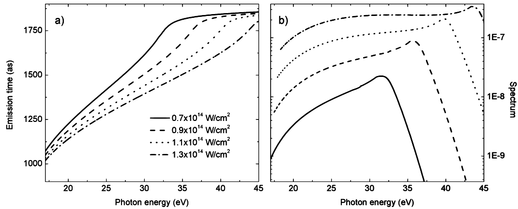
FIGURE 1.6 – Temps d'émission/Délai de groupe des trajectoires courtes uniquement a) et intensité harmonique b) en fonction de l'énergie de photon harmonique et pour différents éclaircements. Calcul fait pour l'Argon, avec un I_p = 15.58 eV et \lambda_L = 800 nm (Diveki [44])
