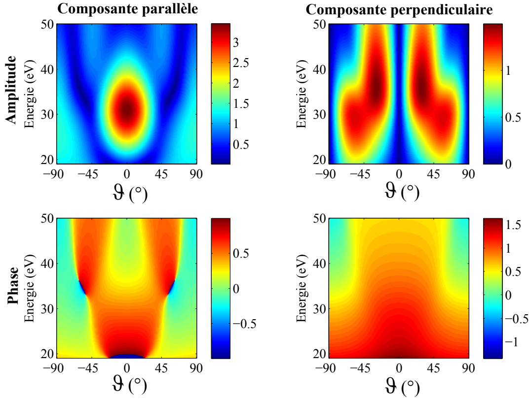
FIGURE 4.21 – Dipôle de photoionisation \mathbf{d}_{\parallel,\perp}^{ion.}(\omega,\vartheta) de la HOMO de N_2 en fonction de l'énergie de photon et de l'angle \vartheta pour les composantes parallèle \parallel et perpendiculaire \perp . La ligne du haut représente l'amplitude de ces composantes tandis que celle du bas représente leurs phases en unité de \pi radian.
