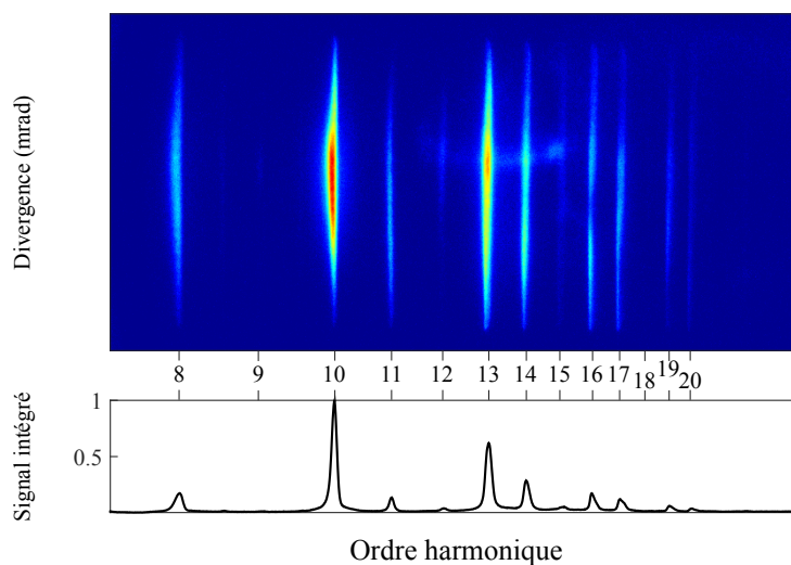
FIGURE 4.45 – Spectre harmonique résolu spectro-spatialement et spectre intégré spatialement obtenus par GHOE dans un gaz d'argon à partir d'une combinaison de deux champs ( 800\text{nm}+400\text{nm} ) de polarisations circulaires d'hélicité opposée.
