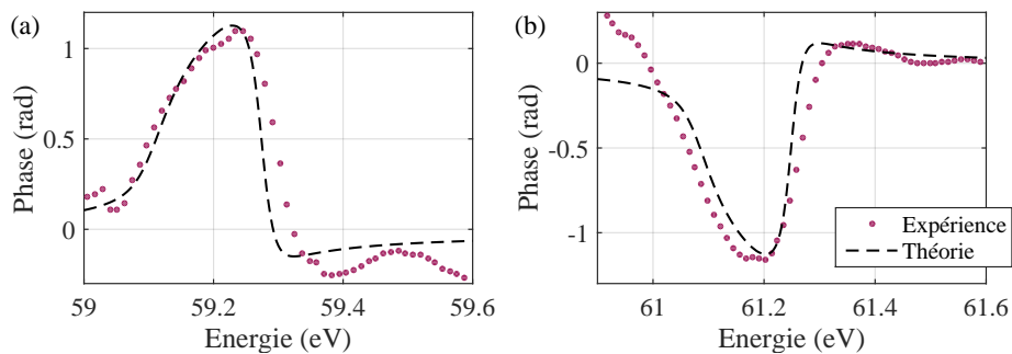
FIGURE 5.27 – Phase résolue spectralement des pics satellites SB62 (a) et SB64 (b), obtenue par GHOE à 1295\text{nm} . Une comparaison avec le modèle théorique est présentée (courbe noire en tirets), pour les deux pics satellites.
