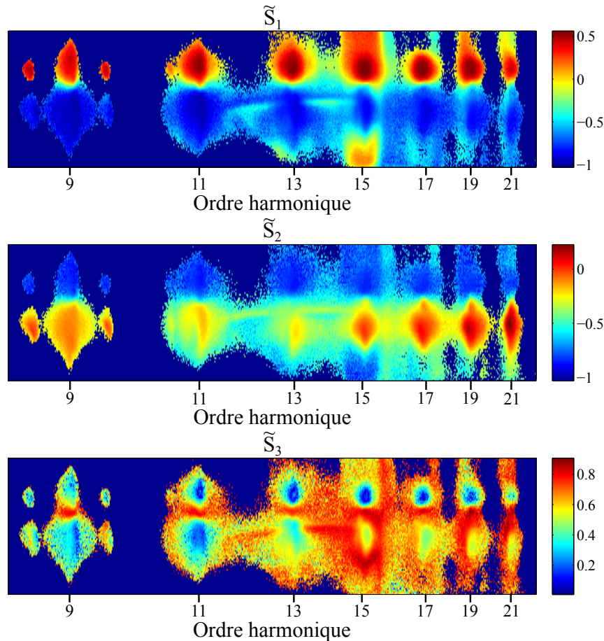
FIGURE 4.11 – Évolution des paramètres de Stokes \tilde{S}_1 , \tilde{S}_2 et \tilde{S}_3^{app} résolus spectrospatialement. Un seuil a été appliqué sur le signal total afin de rendre la figure plus visible.
