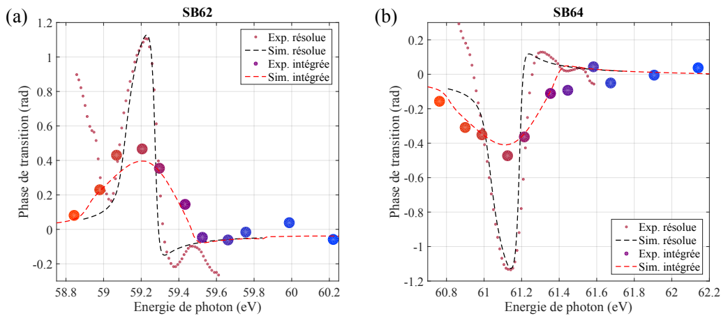
FIGURE 5.30 – Comparaison de l'évolution de la phase des pics satellites (a) SB62 et (b) SB64 pour les deux méthodes utilisées. Dans chaque cas, les courbes simulées et expérimentales sont présentées.
