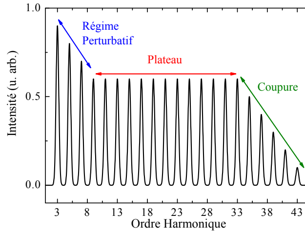
FIGURE 1.1 – Spectre typique obtenu par génération d'harmoniques d'ordre élevé : décroissance rapide pour les toutes premières harmoniques, suivi d'un plateau où l'efficacité est constante et qui se termine par une coupure, où l'efficacité diminue rapidement.
