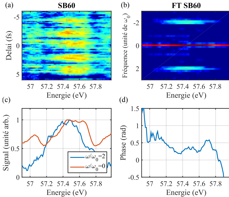
FIGURE 5.24 – (a) Trace RABBIT obtenue à l'aide d'un champ générateur à 1295\text{nm} , zoomée autour du pic satellite SB60. (b) Transformée de Fourier de la Trace RABBIT autour du pic satellite SB60. (c) Amplitude et (d) phase du pic à 2\omega_0 de la transformée de Fourier du pic satellite SB60.
