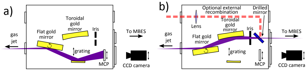
FIGURE 1.10 – Chambre de caractérisation de l'émission harmonique, ou "chambre carrée". Deux configurations sont possibles. Dans la première a) , le faisceau XUV est envoyé dans le spectromètre XUV, permettant de caractériser l'amplitude de l'émission harmonique avec une résolution spatiale suivant l'axe vertical ; dans la seconde b) , le faisceau XUV est envoyé dans un spectromètre à électrons de type bouteille magnétique, permettant une caractérisation de la phase spectrale (moyennée spatialement) de l'émission.
