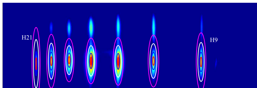
FIGURE 4.8 – Spectre harmonique brut. Présentation des différentes ROI utilisées. Rouge : 0.5 FWHM, bleu : 1 FWHM, blanc : 2 FWHM, mauve : 3 FWHM.
