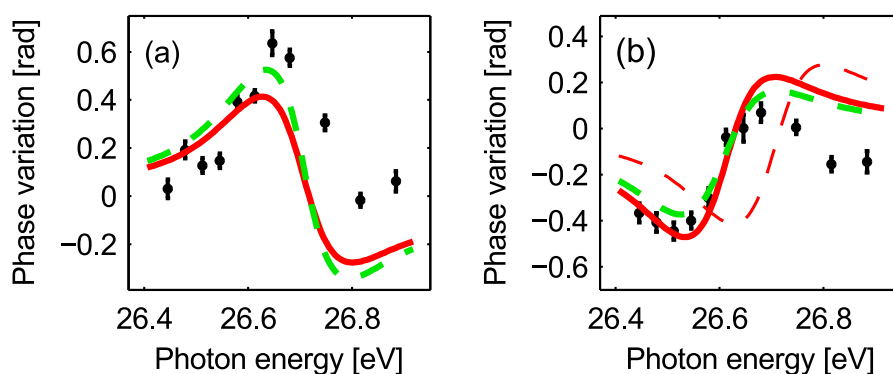
FIGURE 5.6 – Phase des pics satellites (a) SB16 et (b) SB18 en fonction de l'énergie de photon ramené à la position de l'harmonique H17 . Les résultats expérimentaux correspondent aux points noirs. Les résultats théoriques sont représentés par les courbes vertes/rouges avec/sans prise en compte du couplage laser entre l'état résonnant et l'état final dans le continuum. Sur (b), la courbe en tirets fins rouges correspond à l'opposé de la phase extraite de SB16 , afin d'effectuer une comparaison directe entre les deux. Le décalage de 50\text{meV} est associé à un léger décalage vers le bleu du laser fondamental du à l'ionisation du milieu générant les harmoniques (jet d'argon). Extrait de Kotur et al. [114].
