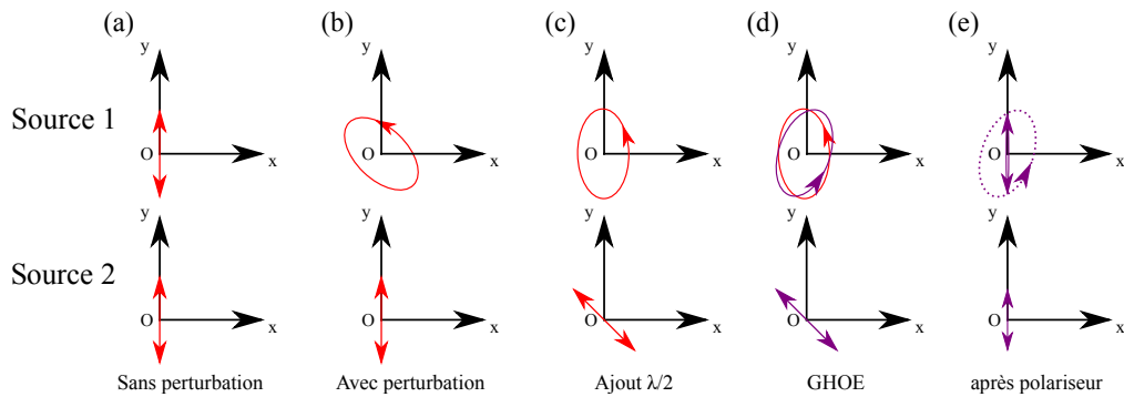
FIGURE 3.12 – Évolution de l'état de polarisation des deux sources lors de la propagation à travers les différents éléments optiques. (a) Juste après l'élément d'optique diffractive, (b), après avoir ajouté le bras de perturbation sur une des sources, (c) après la lame \lambda/2 et (d), après le polariseur.
