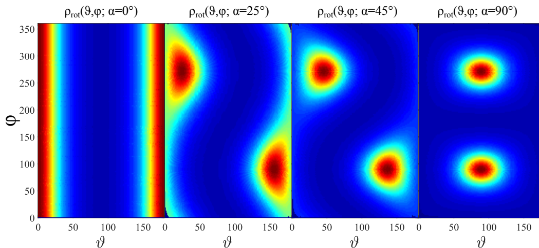
FIGURE 4.23 – Densité de probabilité d'alignement tournée de l'angle \alpha , projetée dans le plan (\vartheta, \varphi) .
