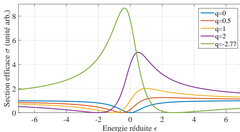
FIGURE 5.11 – Évolution de la section efficace en fonction de l'énergie réduite \epsilon autour d'une résonance autoionisante, pour différentes valeurs de q_{\tilde{a}g} .
