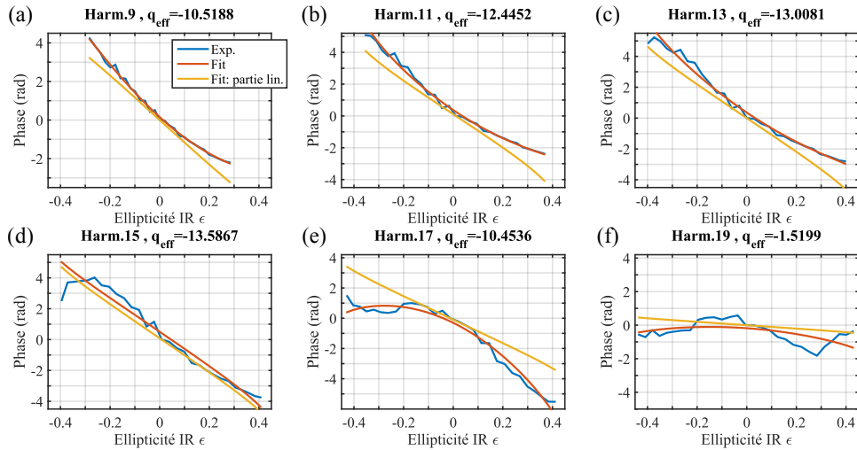
FIGURE 3.13 – Phase en fonction de l’ellipticité du fondamental, pour les ordres harmoniques 9 à 19. Pour chaque figure, 3 courbes sont tracées : la courbe expérimentale (bleu), la courbe lissée par un polynôme d’ordre 2 (rouge) et la partie linéaire de ce lissage (jaune). Pour chaque harmonique, on extrait la pente de la partie linéaire du lissage, dont la valeur est donnée en en-tête.
