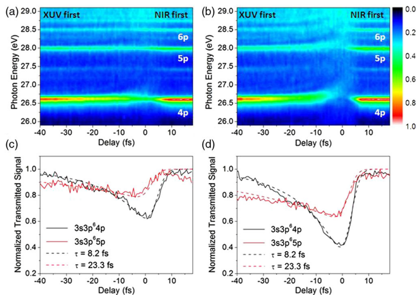
FIGURE 5.1 – Spectre XUV dans la gamme 26 – 29eV après absorption dans un gaz d'argon soumis à un fort champ laser IR, pour différents éclaircissements (a) 5 \times 10^{11} W/cm^2 et (b) 1 \times 10^{12} W/cm^2 . Les délais négatifs correspondent à l'arrivée de l'XUV en premier. Les résonances 3s3p^6 np sont modifiées quand les deux impulsions sont superposées. (c) et (d) : signal des résonances 3s3p^6 4p et 3s3p^6 5p pour les éclaircissements donnés en (a) et (b) resp. Un fit de l'évolution du signal en fonction du délai XUV-IR permet l'accès aux durées de vie des résonances. Extrait de Wang et al. [251].
