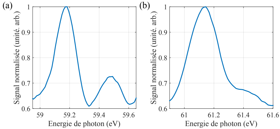
FIGURE 5.26 – Signal intégré en délai et résolu spectralement des pics satellites SB62 (a) et SB64 (b), obtenu par GHOE à 1295\text{nm} .
