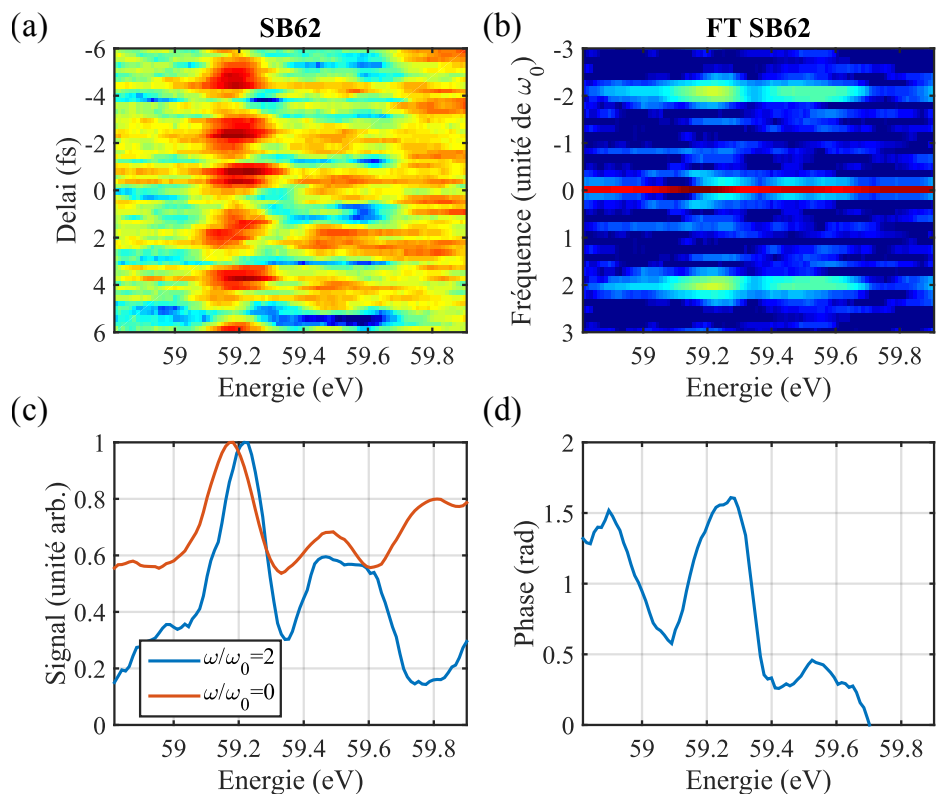
FIGURE 5.25 – (a) Trace RABBIT obtenue à l'aide d'un champ générateur à 1295\text{nm} , zoomée autour du pic satellite SB62. (b) Transformée de Fourier de la Trace RABBIT autour du pic satellite SB62. (c) Amplitude et (d) phase du pic à 2\omega_0 de la transformée de Fourier du pic satellite SB62.
