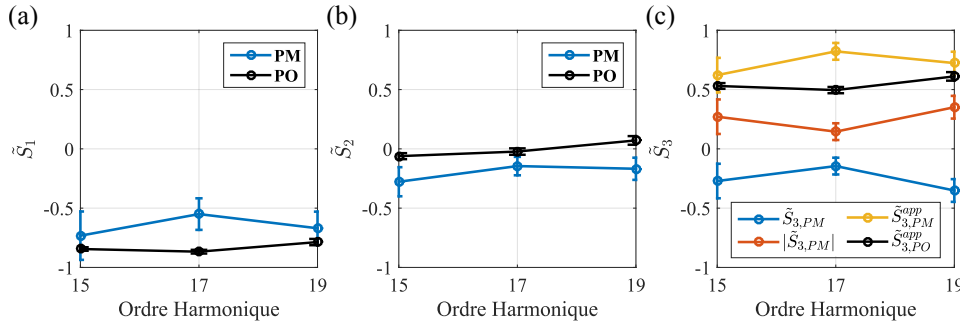
FIGURE 4.13 – Paramètres de Stokes (a) \tilde{S}_1 , (b) \tilde{S}_2 et (c) \tilde{S}_3 obtenus par polarimétrie moléculaire (en bleu) pour les ordres harmoniques 15, 17 et 19. Une comparaison avec les résultats obtenus par polarimétrie optique (en noir) est faite à chaque fois. Pour la Figure (c), deux courbes supplémentaires ont été ajoutées : la valeur absolue de \tilde{S}_3 (rouge) ainsi que l'évolution de \tilde{S}_3^{app} (en supposant la lumière complètement polarisée), les deux obtenus à partir de la polarimétrie moléculaire.
