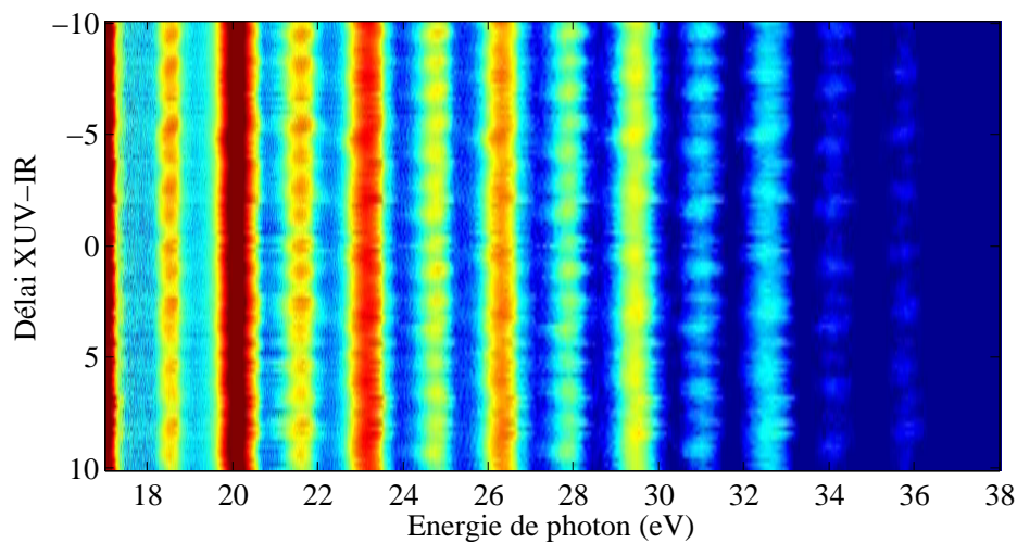
FIGURE 1.16 – Trace RABBIT obtenue à 800nm dans la photoionisation de l'Argon.
