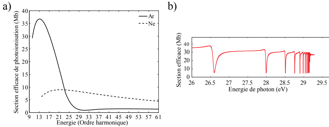
FIGURE 1.12 – Sections efficaces de photoionisation de l'argon et du néon en fonction de l'ordre harmonique à 800nm a) et b) , Section efficace de photoionisation de l'argon zoomée sur la gamme [26, 29.5] eV.
