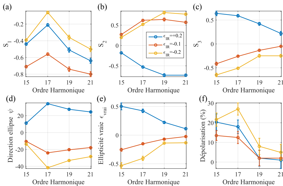
FIGURE 4.40 – Paramètres de Stokes (a-c), direction de l'ellipse de polarisation \psi (d), ellipticité vraie \epsilon_{vrai} (e) et apparente \epsilon_{app} . et taux de dépolarisation (f) pour les harmoniques 15 à 21 générées par un champ IR polarisé elliptiquement, avec \epsilon_{IR} = -20\% (jaune), \epsilon_{IR} = -10\% (rouge) et \epsilon_{IR} = +20\% (bleu), obtenus par combinaison des mesures effectuées par PO et PM .
