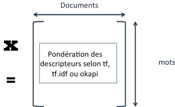
FIGURE 3.3: Représentation vectorielle
