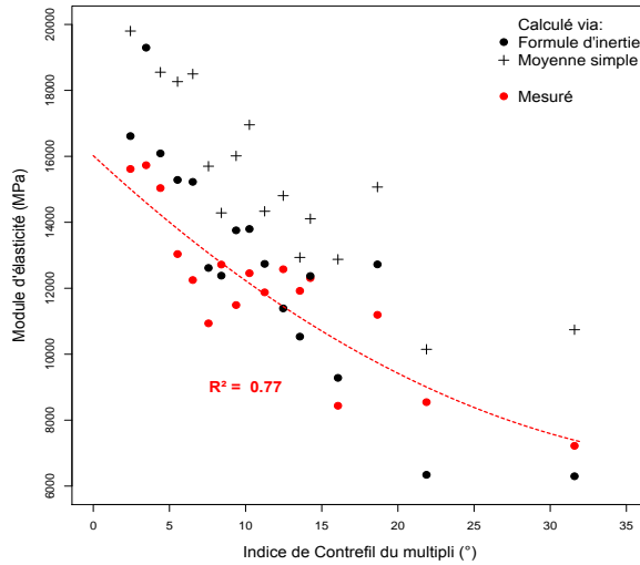
Figure 123 : Variation du module d'élasticité de l'éprouvette sèche selon l'ICF et comparaison aux valeurs calculées. Les points rouges représentent les valeurs mesurées. Les ronds et les croix noires correspondent aux modules calculés Inertie et E_{moy} . La droite pointillée rouge représente le modèle ajusté pour les valeurs mesurées ( R^2=0,77 ).
