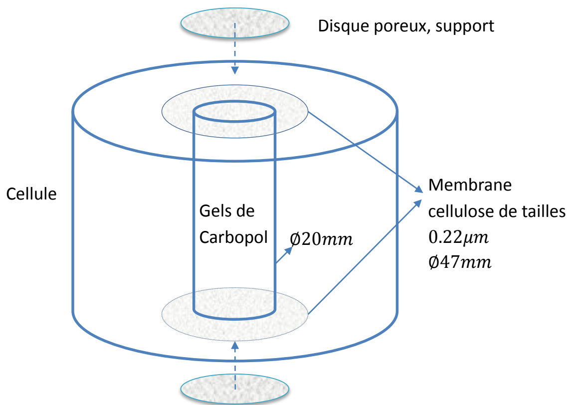
Figure.1- 9 Détail de la cellule de perméabilité
