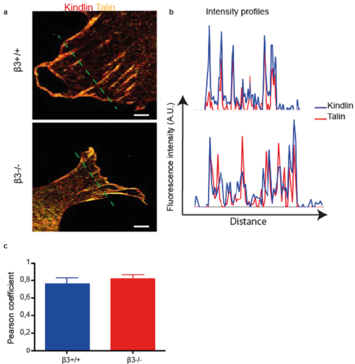
Figure III.4.4 La colocalisation de la taline et de la kindline n'est pas régulée par l'intégrine \beta3 . a) Zoom d'une image « merged » montrant la localisation de la kindline (rouge) et de la taline (jaune) dans les cellules \beta3^{+/+} et \beta3^{-/-} adhérentes sur des gels de 5kPa fonctionnalisés à la fibronectine. b) Profile d'intensité de fluorescence (unité arbitraire) mesuré le long de la ligne en pointillés vert montrant la colocalisation entre la taline et la kindline. c) Quantification du degré de corrélation via le coefficient de Pearson confirmant le haut degré de corrélation de ces deux protéines (1= colocalisation parfaite, 0= distribution non corrélée). n=5 cellules/ condition (moyenne \pm s.e.m). Bar d'échelle=6 \mu m.
