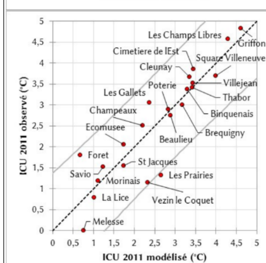
Figure 54, résultats de trois régressions linéaires de l'ICU moyen observé en 2011.
