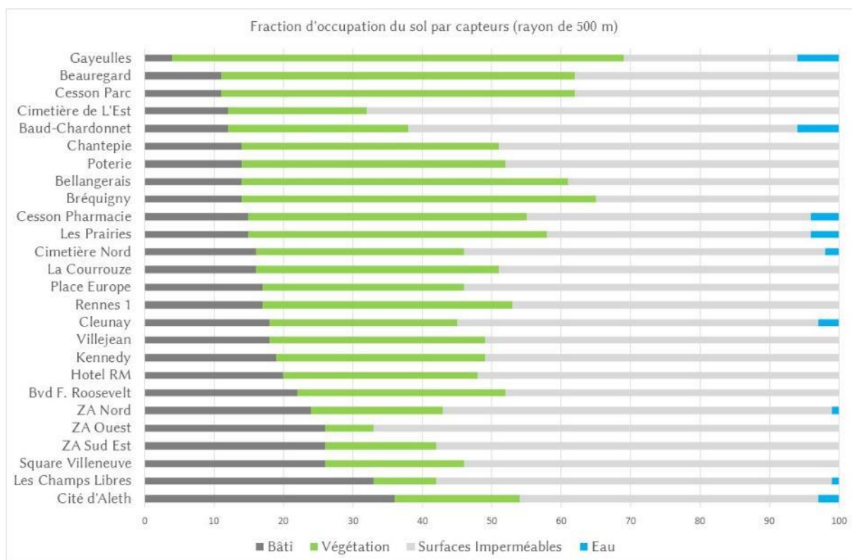
Figure 29, classement des capteurs de température installés dans l'espace intra-urbain à Rennes, trié par fraction de surfaces bâties.
