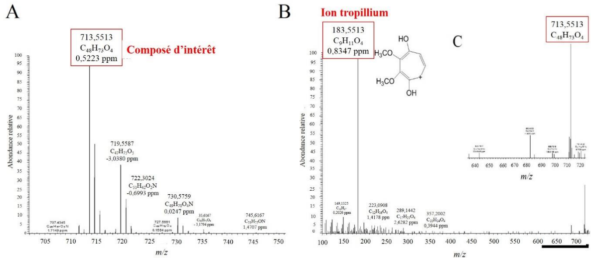
Figure 62 : (A) Spectre de masse du composé d'intérêt purifié élué à 7,5 min par analyse des extraits lipidiques de la souche ΔubiE cultivée dans du LB en conditions anaérobies. (B) Spectre de fragmentation de l'ion moléculaire 713,5513. (C) Zoom sur la région m/z=640-720 du spectre de fragmentation du B.
